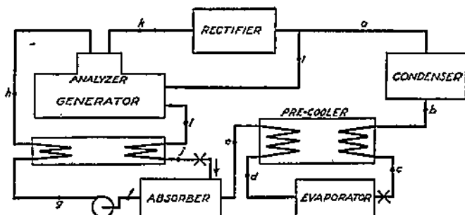
FIG. 5-2. Elements of Actual Absorption System.
