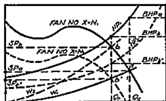
FIG. 15-10. Volume Control.
