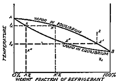
Fig. 5-3. Boiling Point Diagram.
