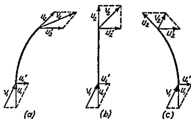
FIG. 15·2. Fan Blade Velocity Vectors.
