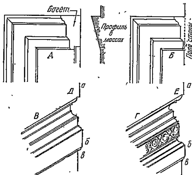
Рис. 94. Профили филленок.
