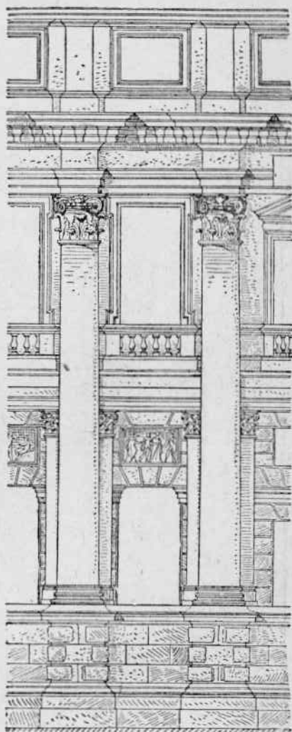
Рис. 63. Палаццо Вальмарана в Виченце. Палладио.
