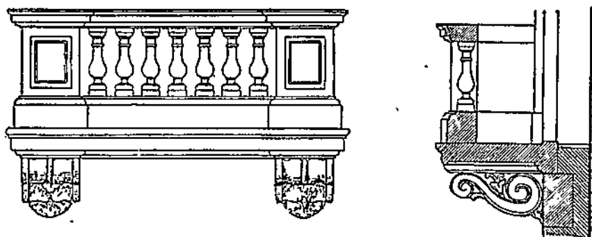
Рис. 191. Фасад и разрез балкона.
