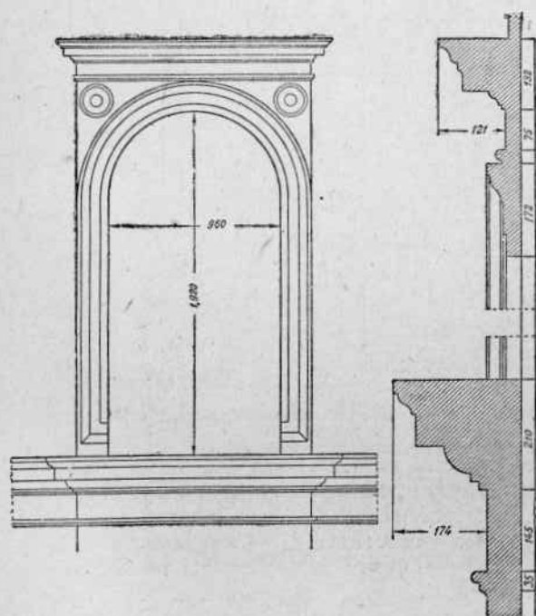
Рис. 164. Окно одного из домов на Виа дель Таверно Веккио в Риме.
