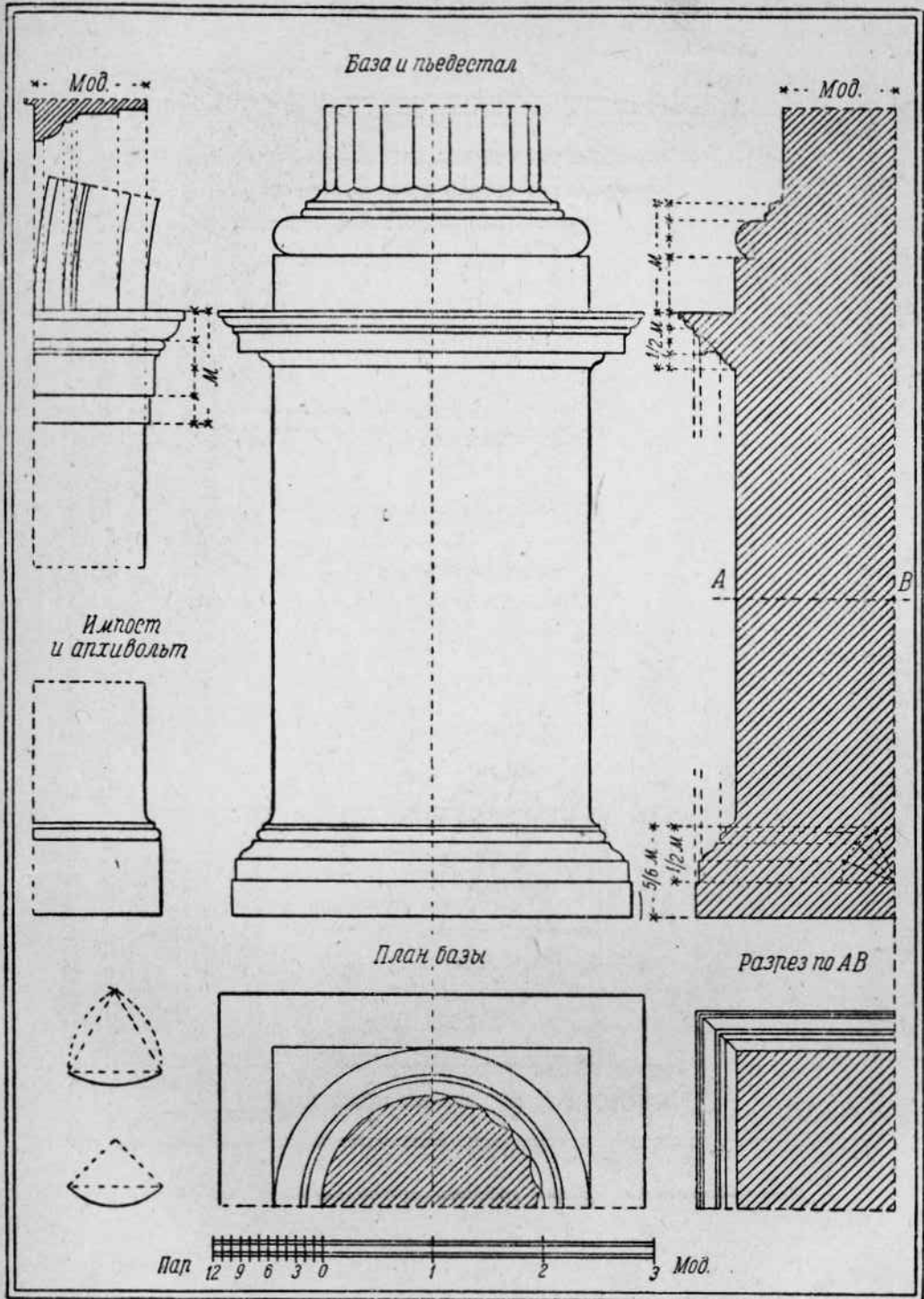
Римско-дорический ордер—база и пьедестал.
