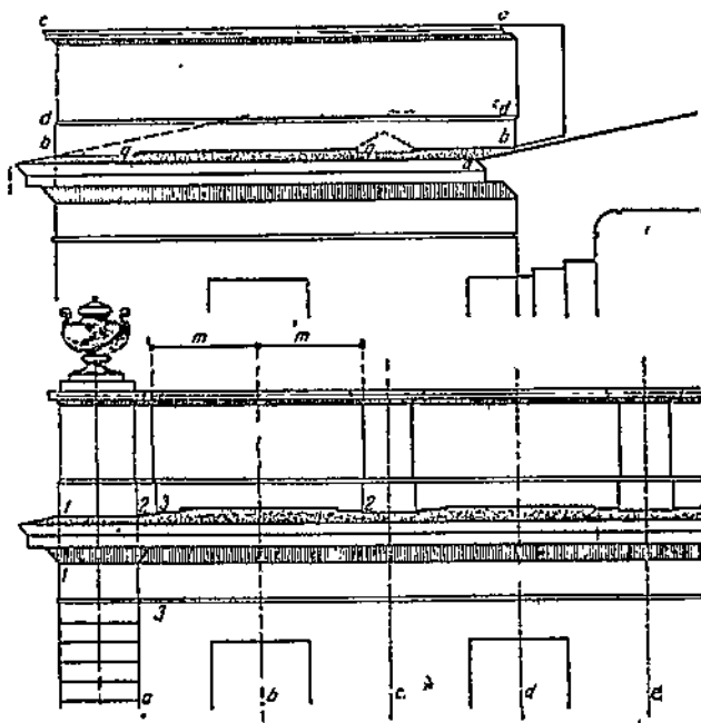
Рис. 145. Парапеты.
