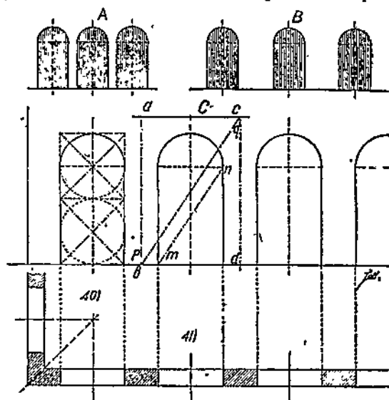
Рис. 40—41. Пропорции аркад.
