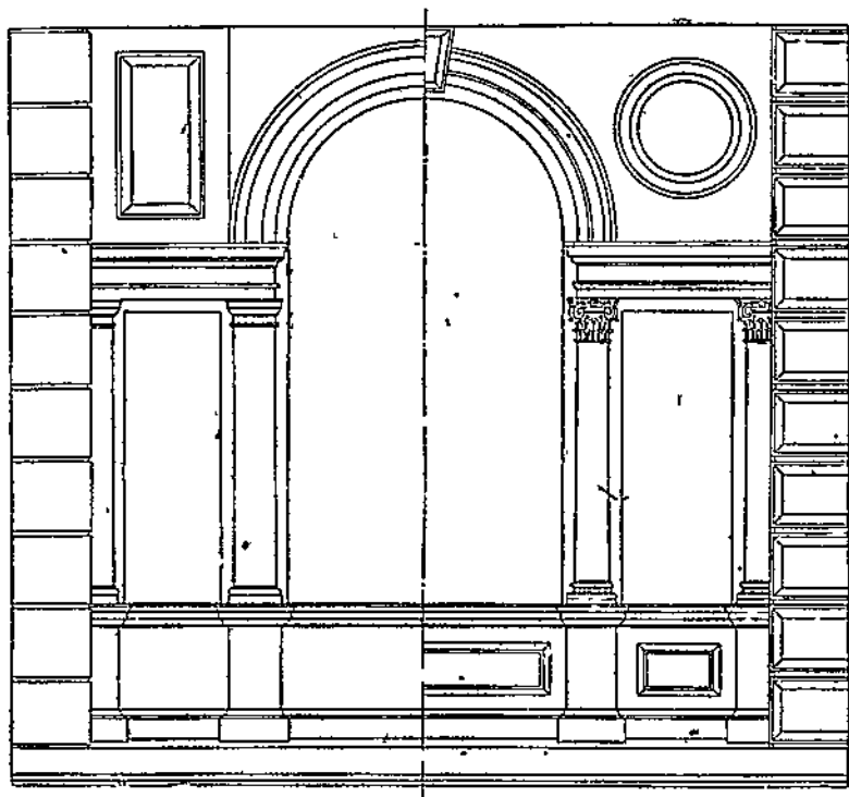
Рис. 179. Палладиева система.
