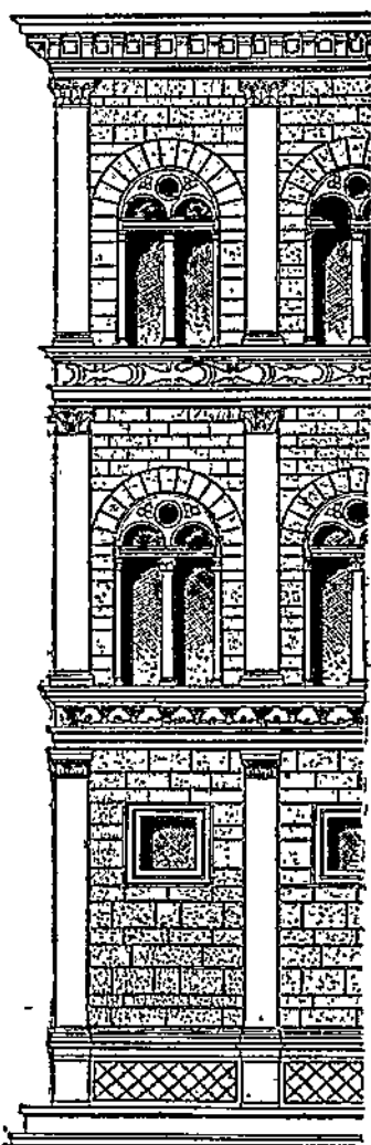
Рис. 60. Палаццо Ручеллаи во Флоренции. Альберти.
