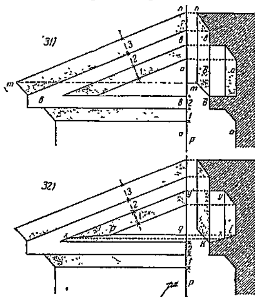
Рис. 31—32. Построение фронтона.
