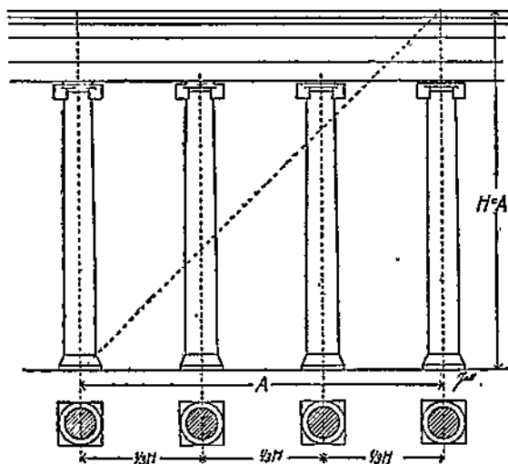
Рис. 25. Часть колоннады.
