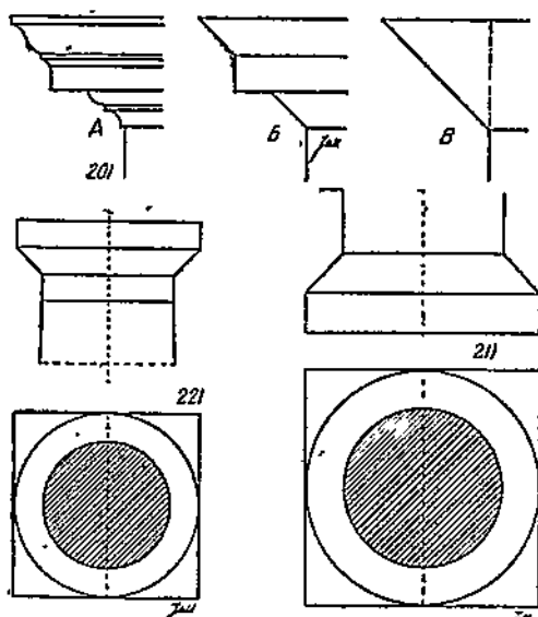
Рис. 20—22. Карниз, база и капитель.
