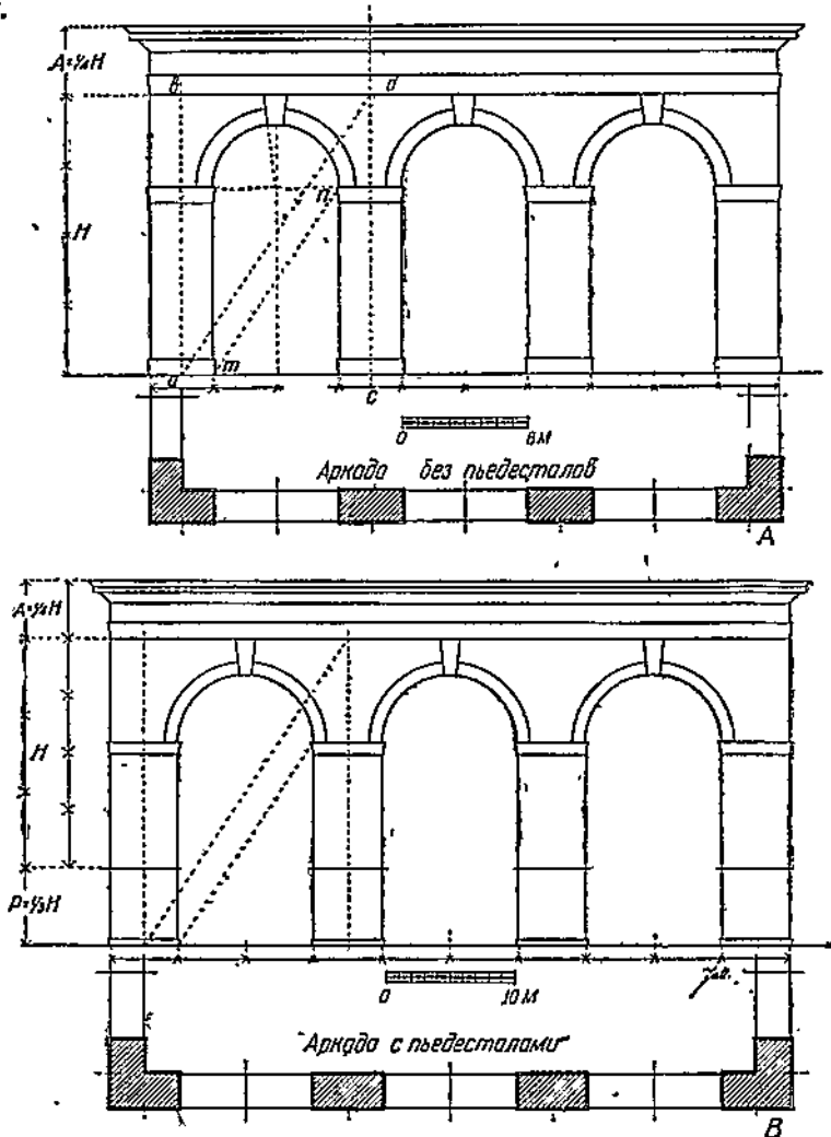
Рис. 42. Аркады без пьедесталов и аркады с пьедесталами.
