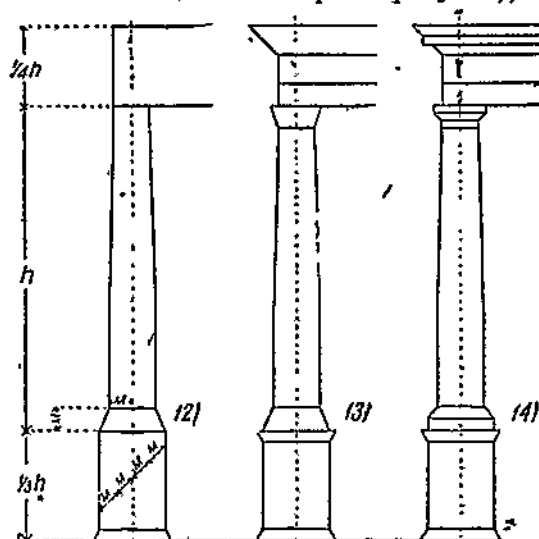
Рис. 12—14. Последовательное построение ордера.
