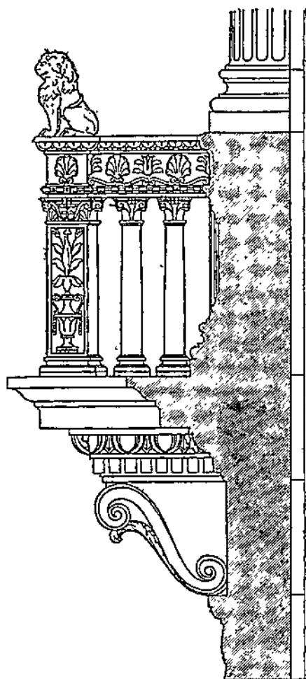
Рис. 193. Балкон палатцо Вендрамин в Венеции. Ломбардо.
