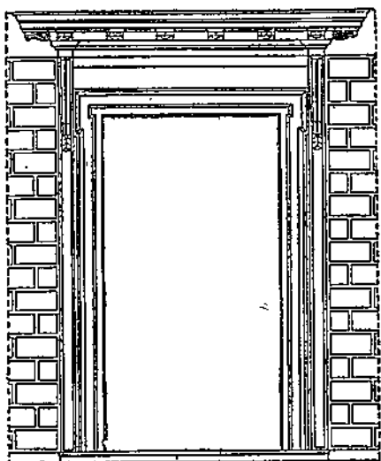
Рис. 185. Дверь с наличником, контр-наличником и сандриком. Визьола.
