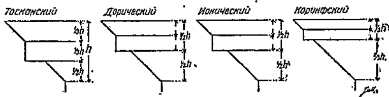
Рис. 23. Венчающие карнизы в массах.
