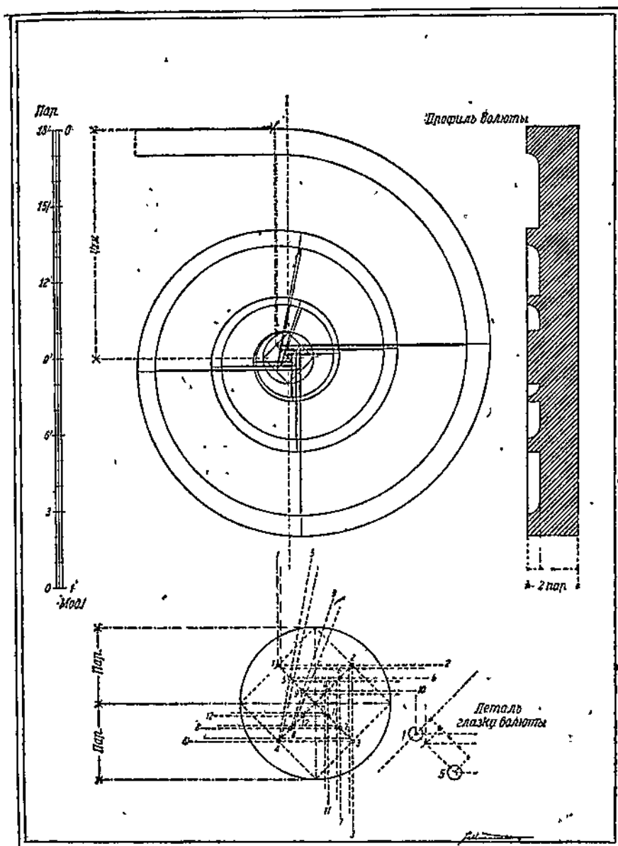
Построение вальюты ионической капители.
