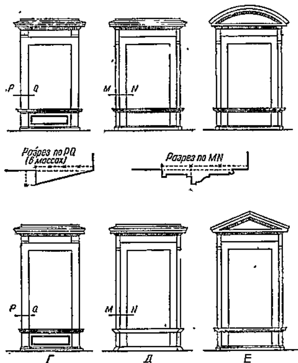
Рис. 154. Обработка прямоугольных окон.
