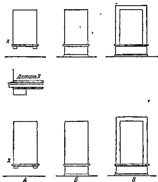
Рис. 153. Обработка прямоугольных окон.
