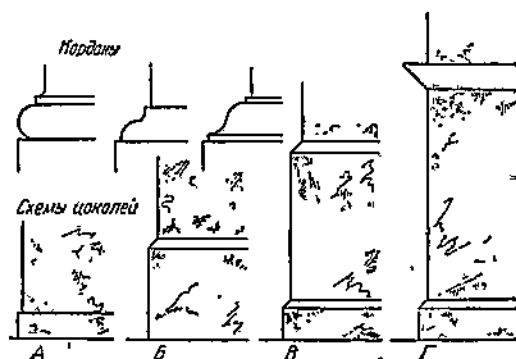
Рис. 66. Схемы цоколей.
