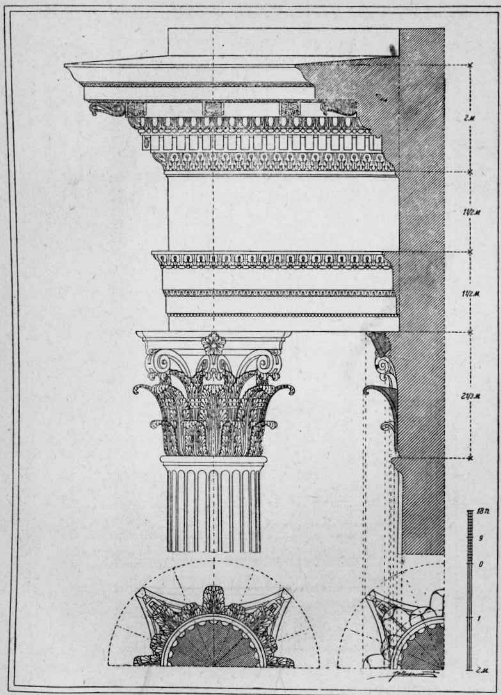
Римско-коринфский ордер—антаблемент и капитель.
