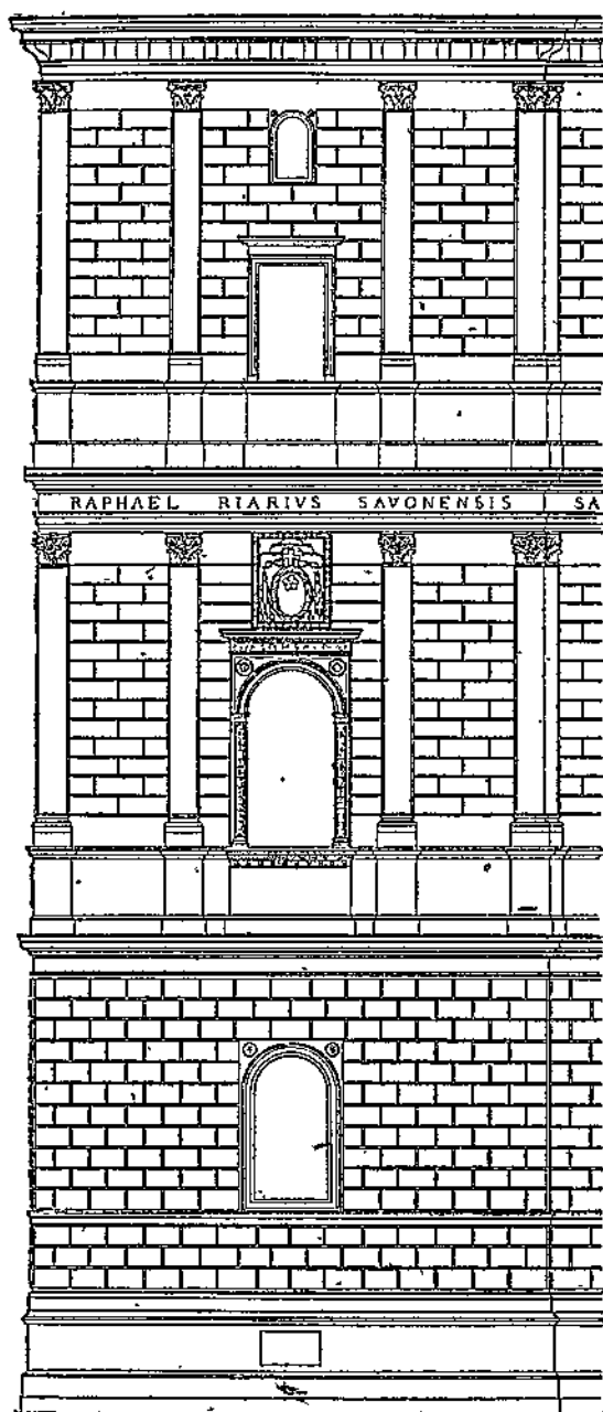
Рис. 72. Канцеллерия в Риме. Браманте.
