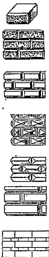
Рис. 76. Русты.
