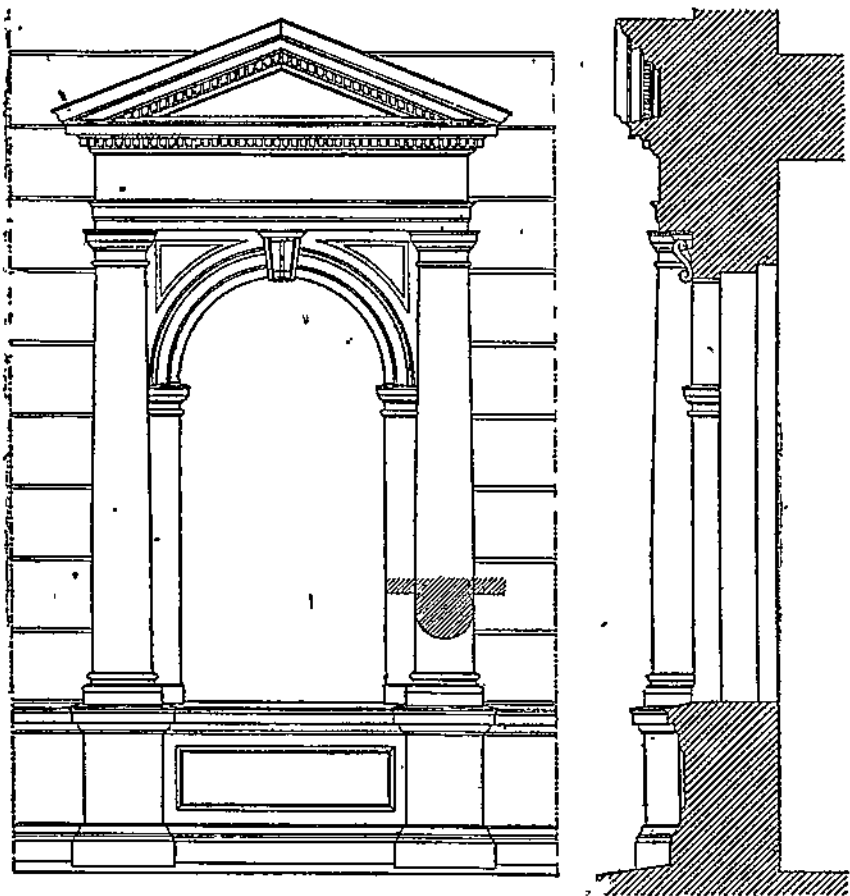
Рис. 166. Применение ордеров при обработке полуциркулярных окон.
