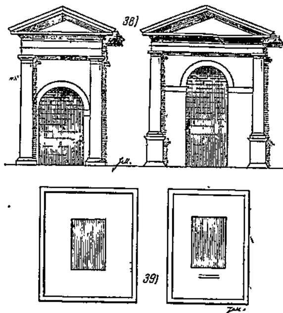
Рис. 38—39. Примеры неудачных пропорций обрамлений.
