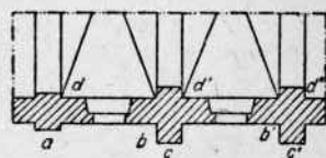
Рис. 115. Контрфорсы.
