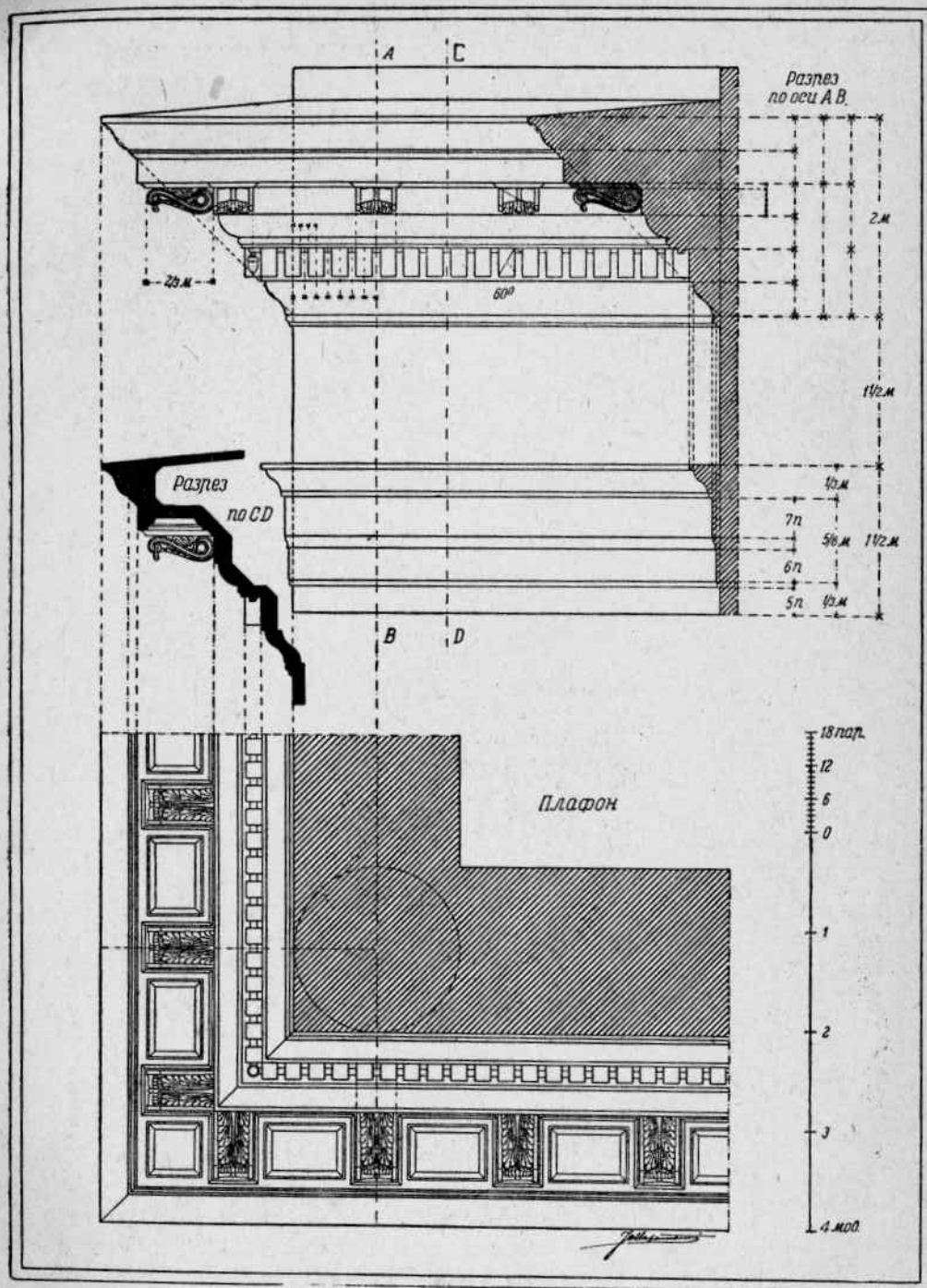
Римско-коринфский ордер—плафон.
