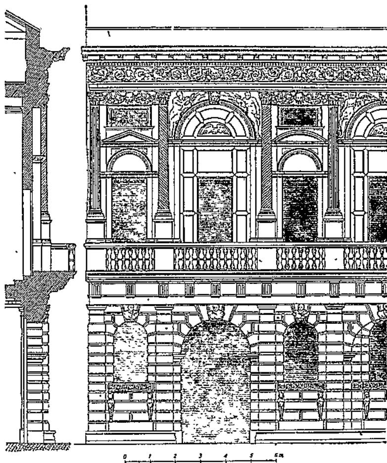
Рис. 124. Палаццо Бевилакка в Вероне. Санмикеле.
