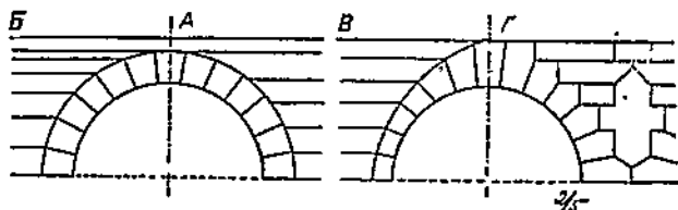
Рис. 82. Сопряжение швов рустов.
