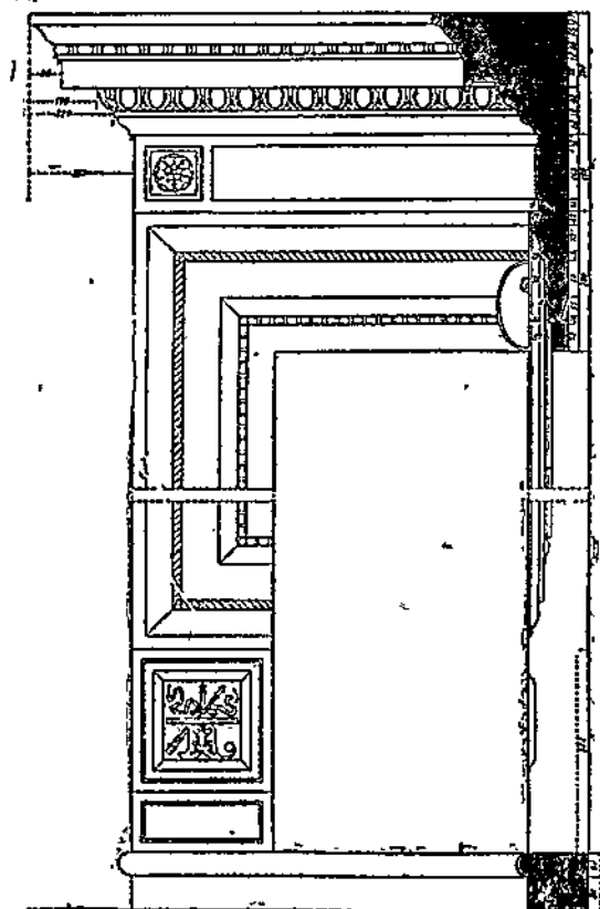
Рис. 184. Дверь с наличником и сандриком.
