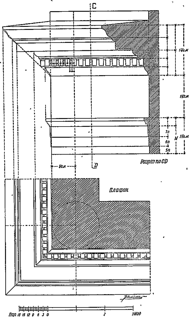
Римско-ионический ордер—плафон.
