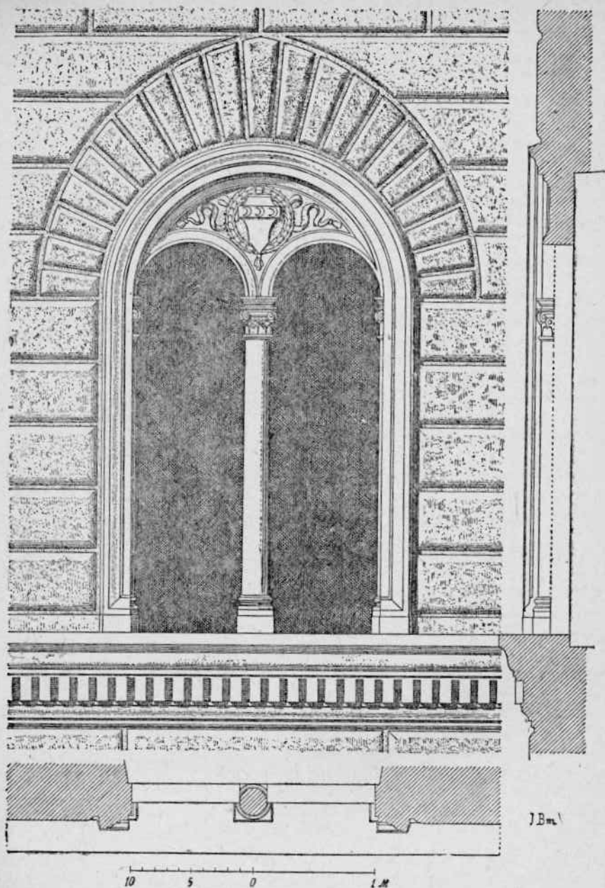
Рис. 168. Окно палатцо Строрци во Флоренции.
