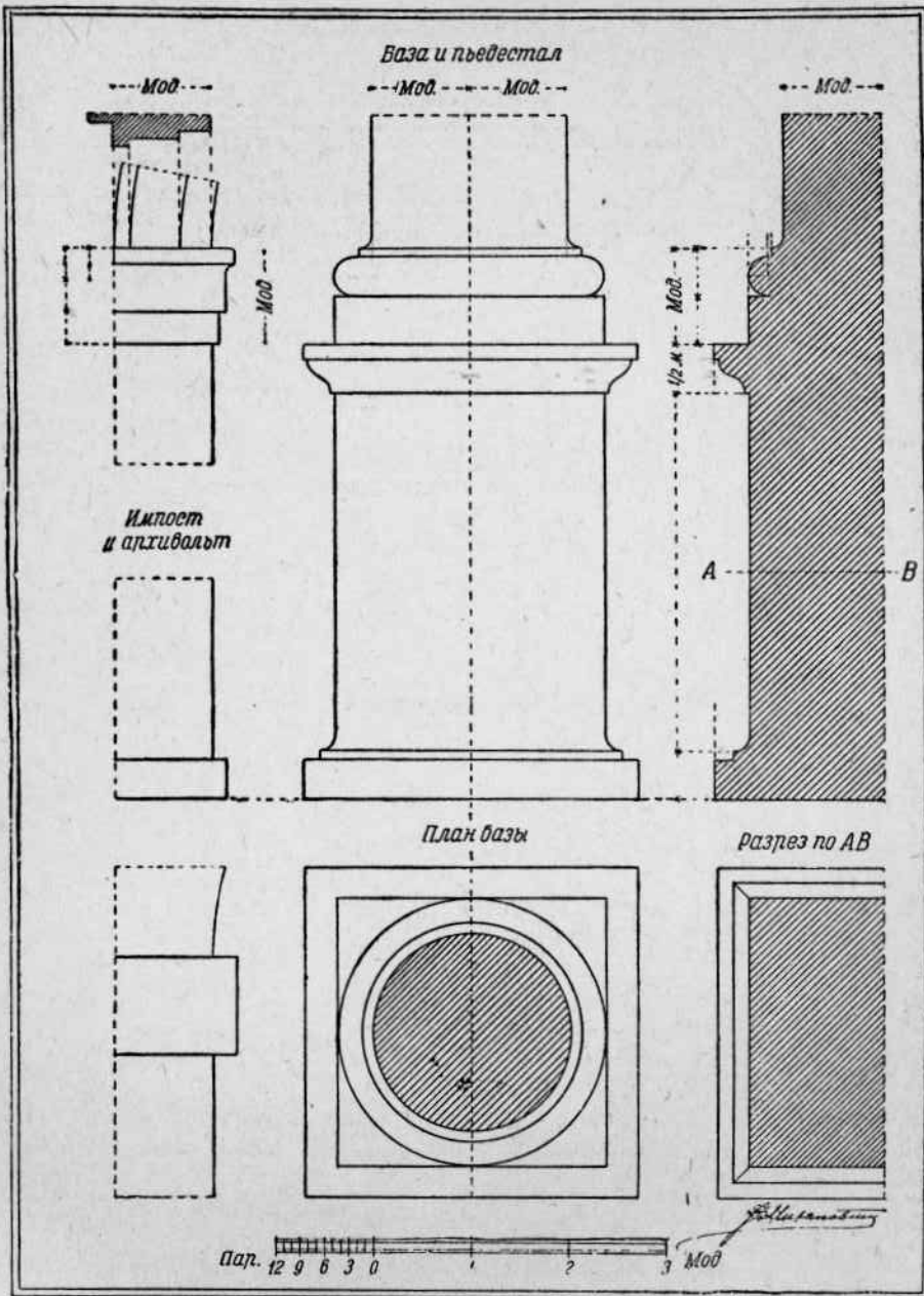
Тосканский ордер—база и пьедестал.
