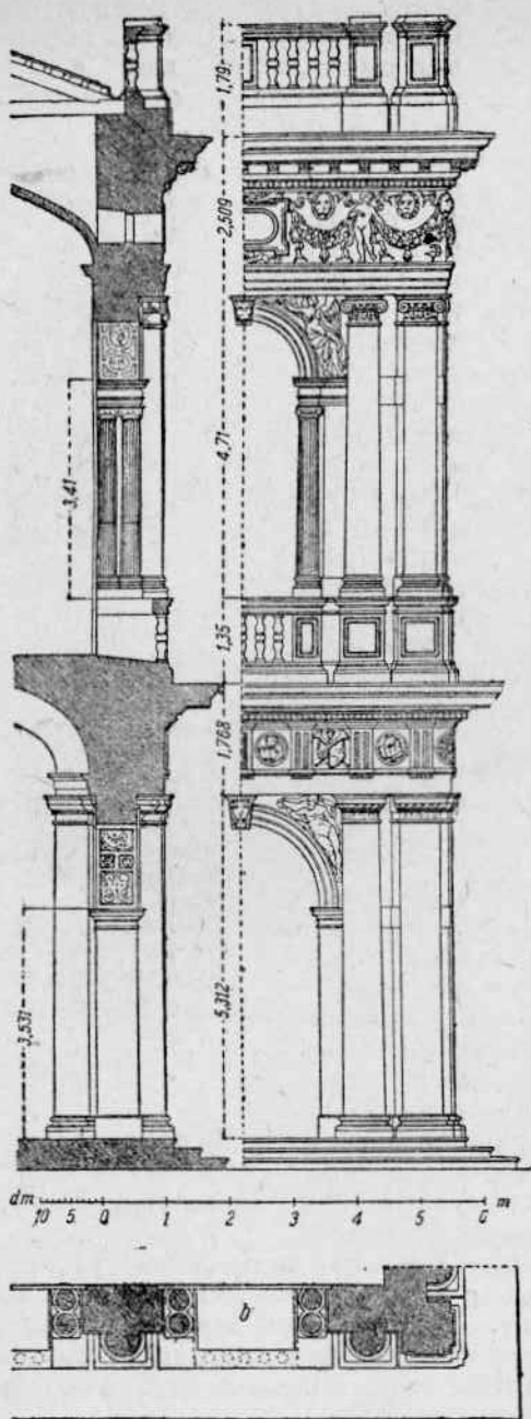
Рис. 131. Библиотека св. Марка в Венеции. Сансовино.
