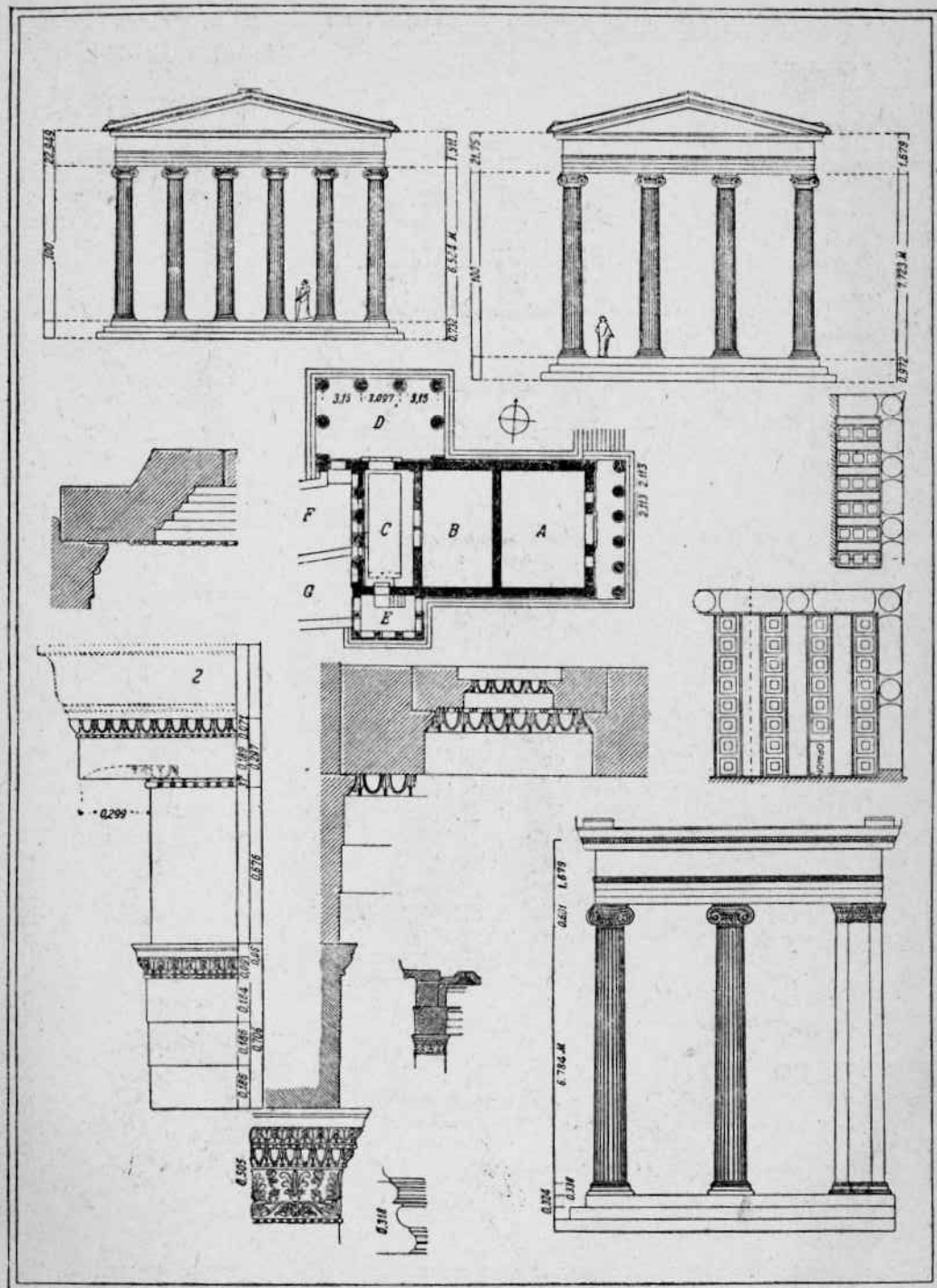
Греко-ионический ордер (Эрехтейон).
