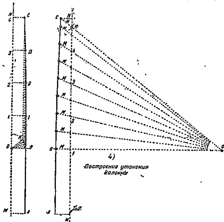
Рис. 3 и 4. Построение утонения колонны.
