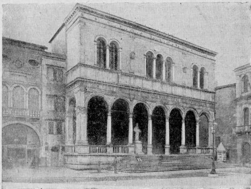
Рис. 177. Лоджия дель Консиглио в Падуе. Россетти.
