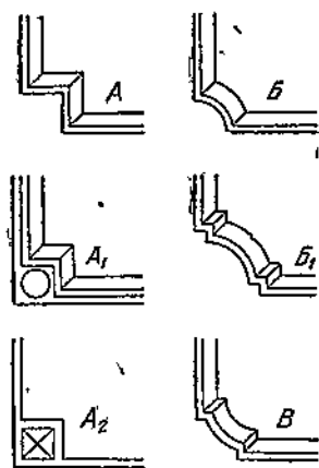
Рис. 95. Углы филенок.
