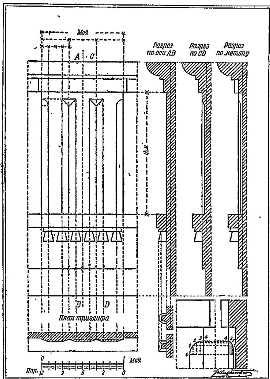
Римско-дорический ордер—детали триглифа.
