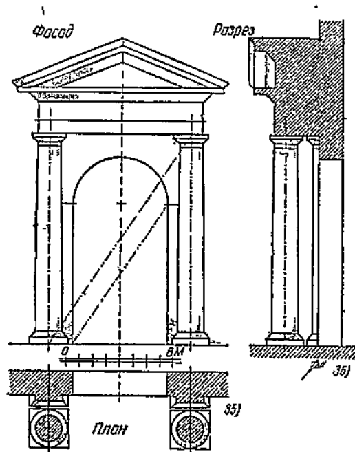
Рис. 35—36. Обработка входа отдельно стоящими колоннами.
