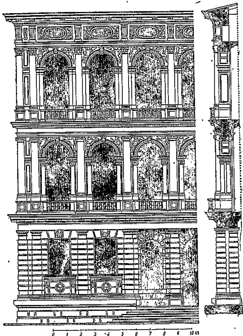
Рис. 125. Палаццо Реццоникьо в Венеции. Лонгена.
