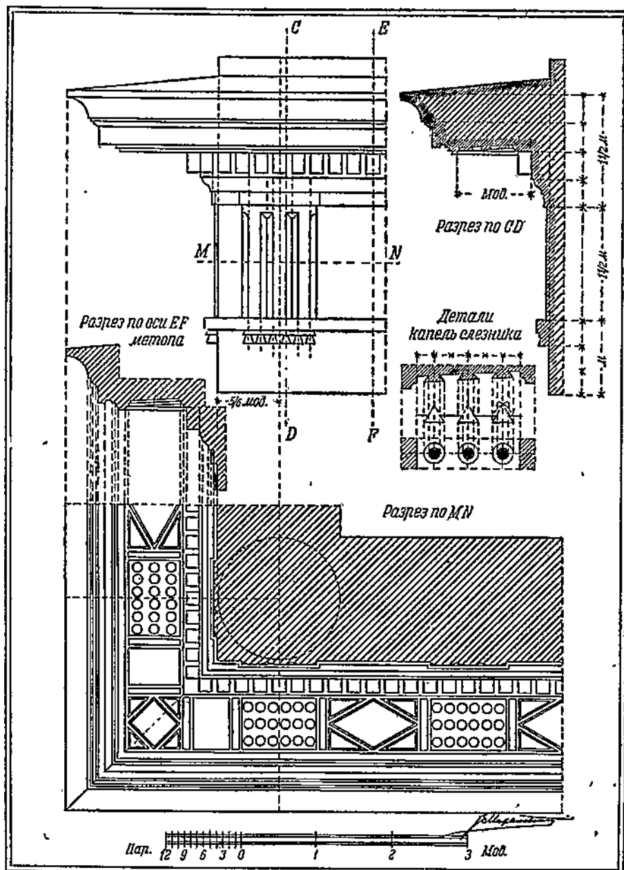
Римско-дорический ордер с зубцами—плафон.
