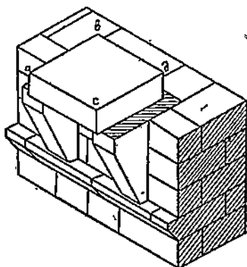
Рис. 72. Конструкция карниза на кронштейнах.
