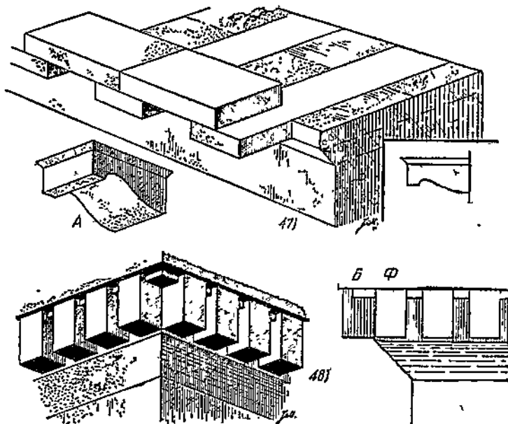
Рис. 47—48. Модульоны и зубцы.
