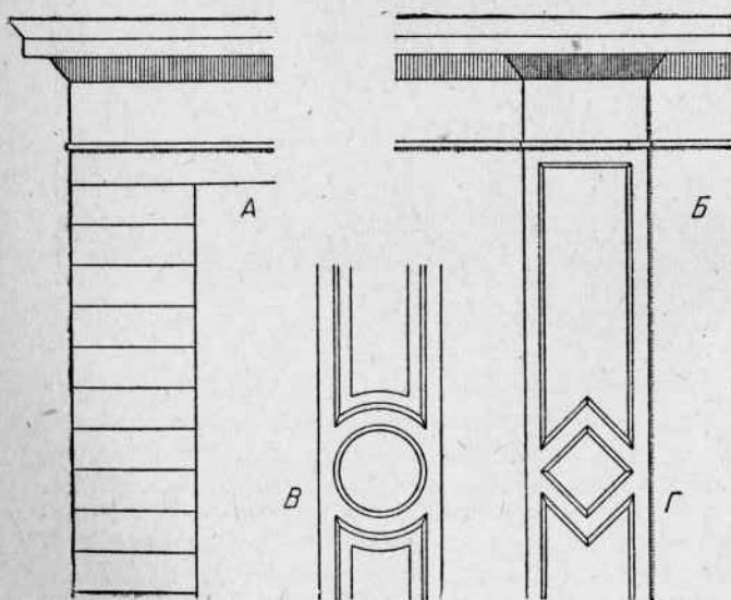
Рис. 114. Лопатки.
