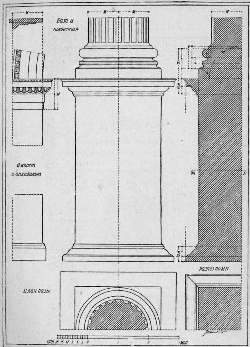
Римско-коринфский ордер—база и пьедестал.
