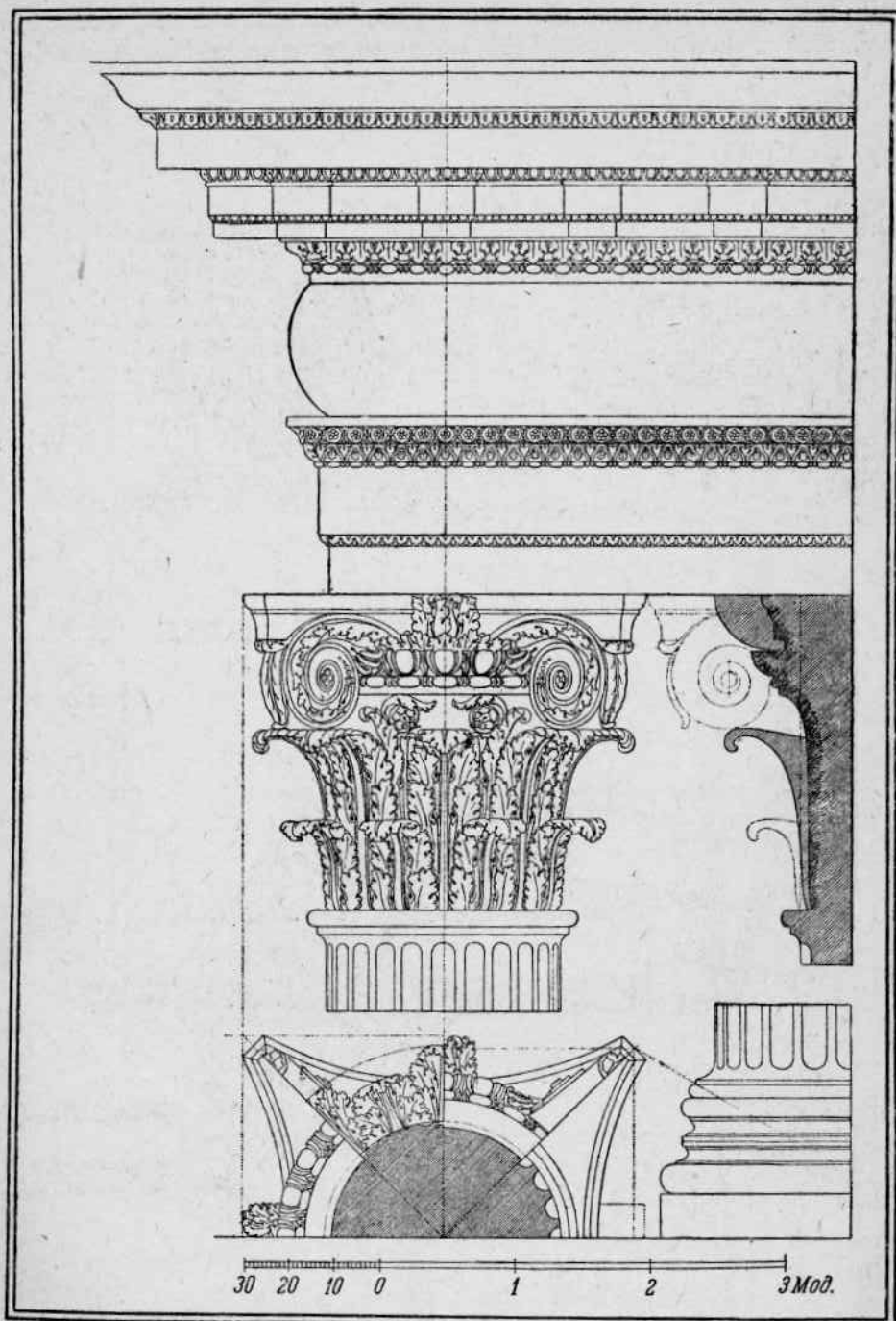
Сложный ордер (по Палладио).
