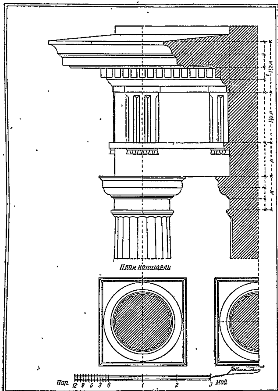
Римско-дорический ордер с зубцами—антаблемент и капитель.
