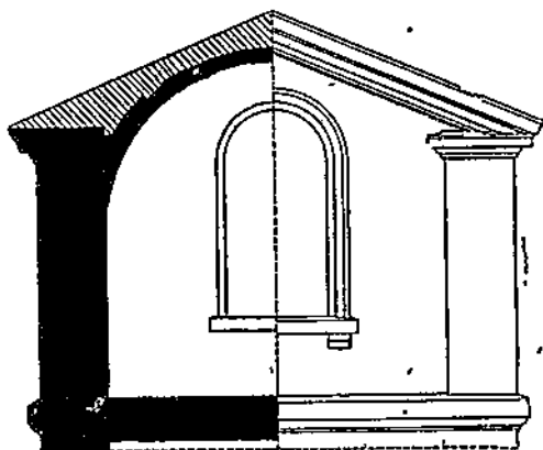
Рис. 144. Полуфронтон.
