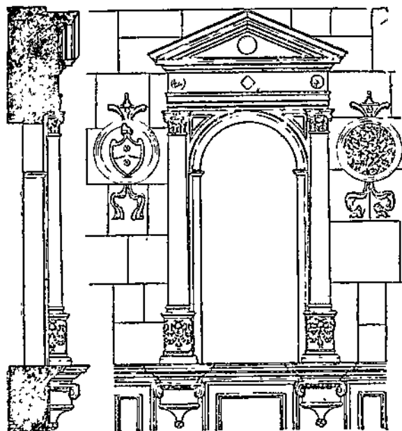
Рис. 160. Окно дворового фасада дворца Дожей в Венеции.
