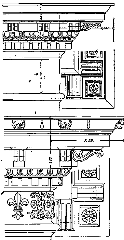
Рис. 70. Вверху — карниз палатцо Строцци во Флоренции. Кронана. Внизу — карниз палатцо Фарнеше. Микельанджело.
