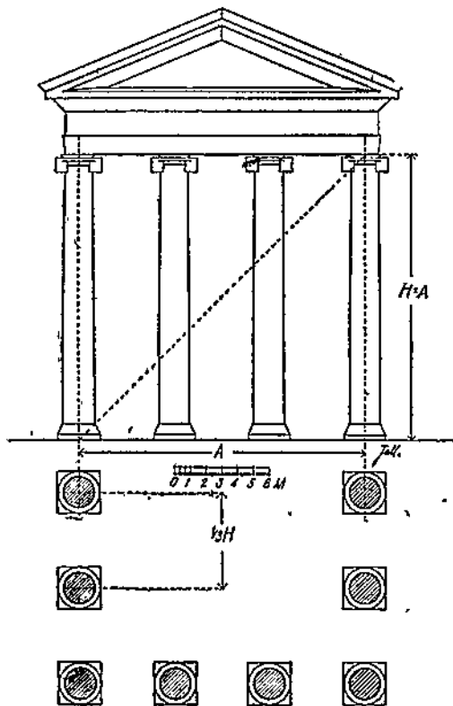
Рис. 24. Колоннада.
