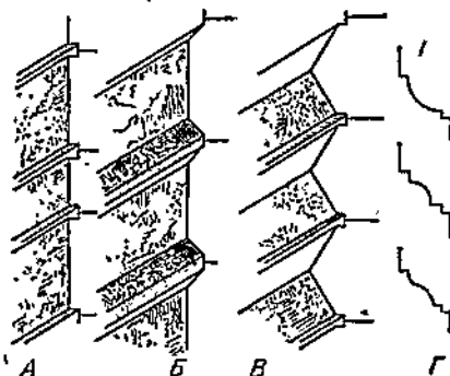
Рис. 77. Профили рустов.
