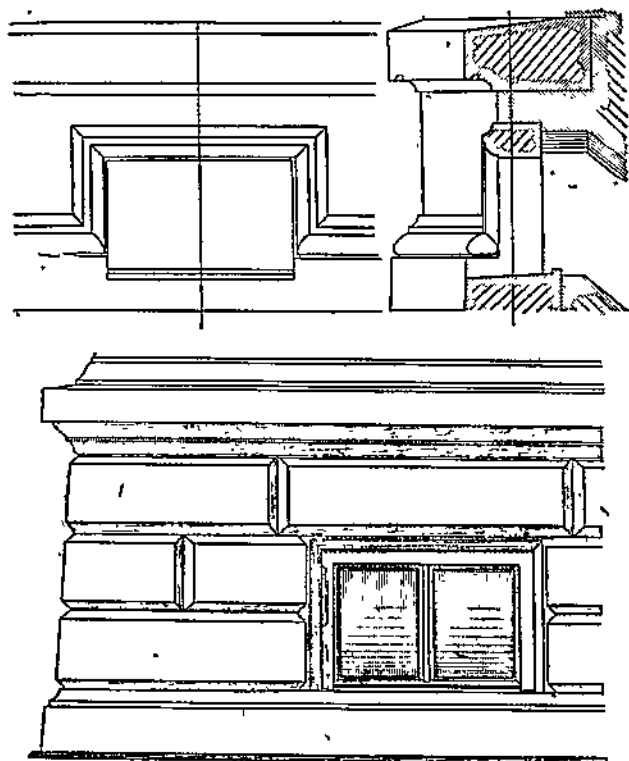
Рис 67. Цокольный этаж.
