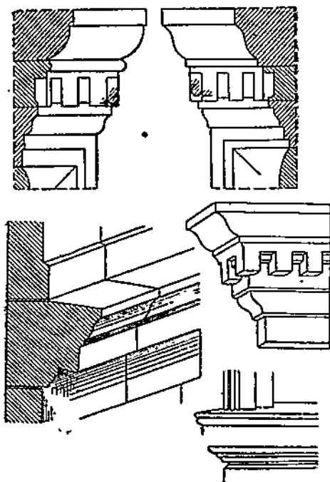
Рис. 107. Подоконные тяги.
