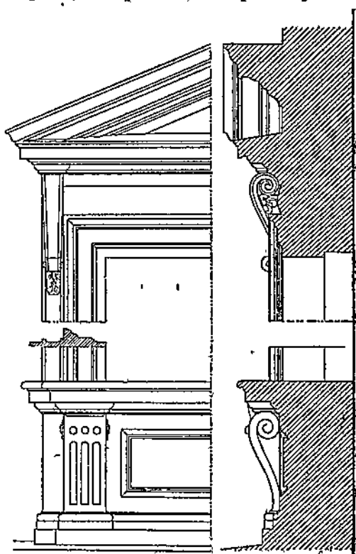
Рис. 155. Окно Виньола.
