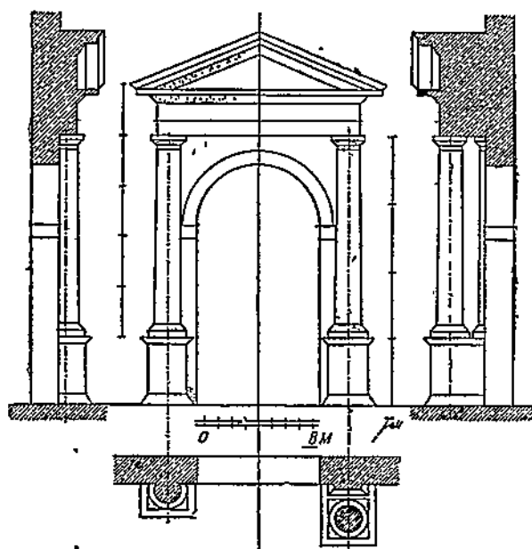
Рис. 37. Обработка входа колоннами с пьедесталом.
