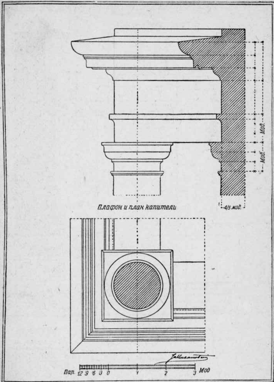
Тосканский ордер—антаблемент и капитель.
