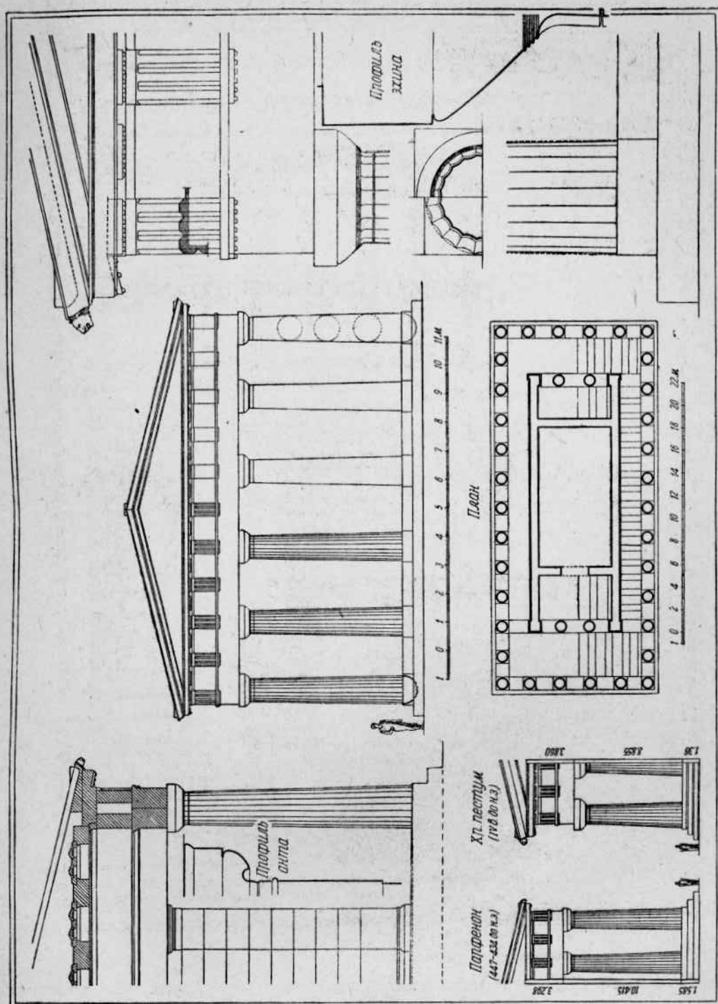
Греко-дорический ордер.
