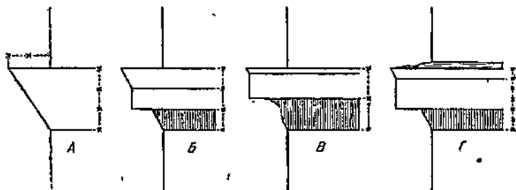
Рис. 103. Междуэтажные карнизы в массах.
