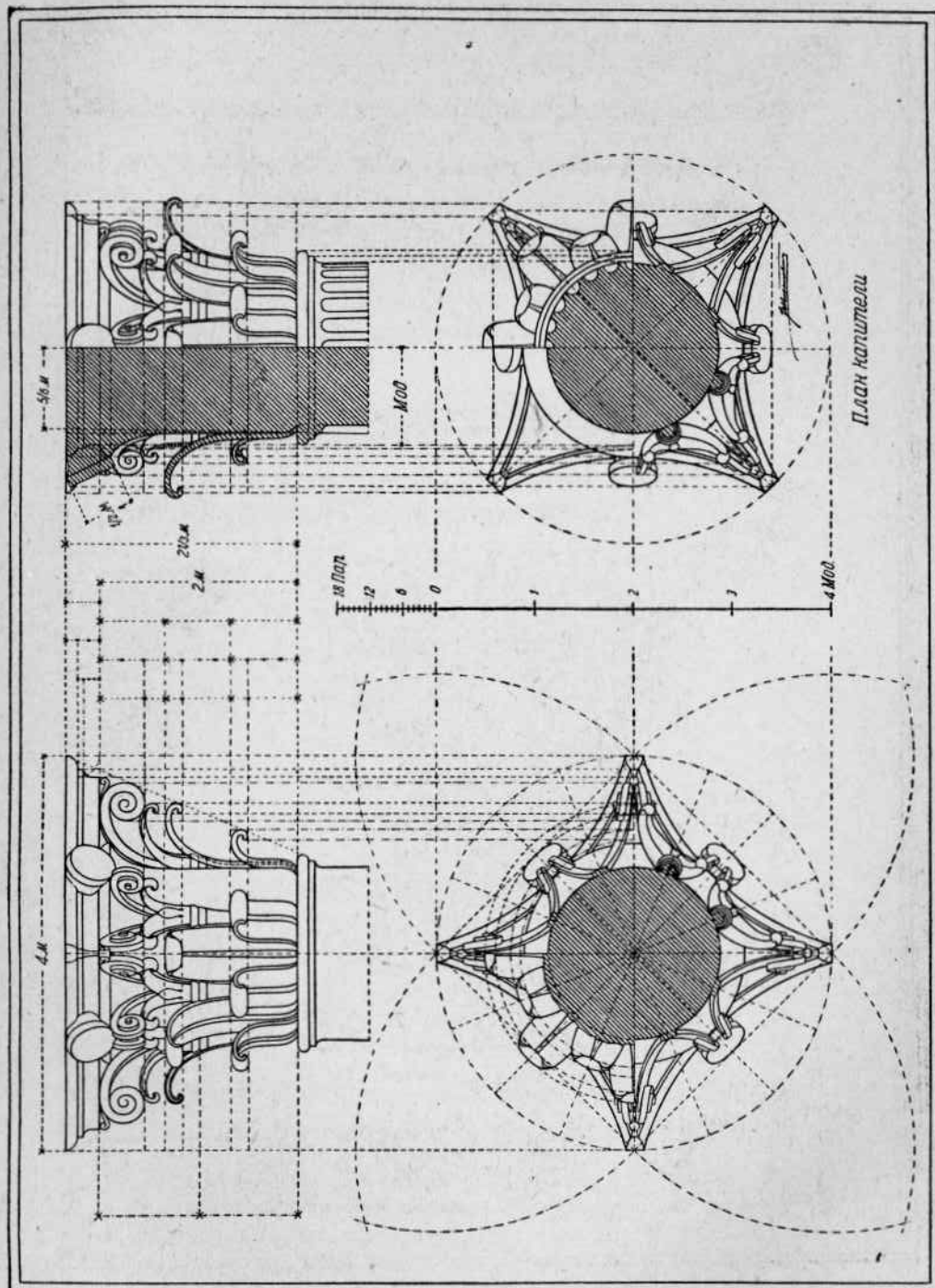
Построение римско-коринфской капители.
