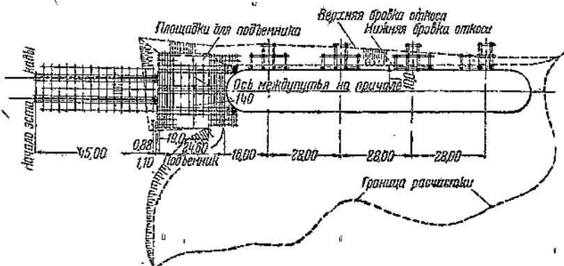
Фиг. 15. План расположения свайных причальных кустов и механического подъемника
