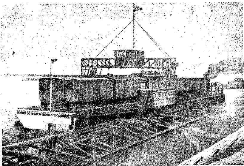
Фиг. 37. Самоходный железобетонный паром
