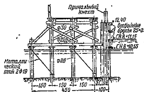
Деталь отбойного куста свай и отбойного бруса
