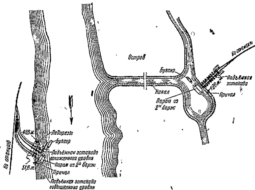
Фиг. 9. План расположения причалов и канала переправы поперечного типа
