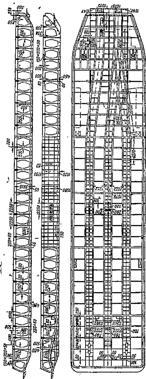
Фиг. 39. Конструкция корпуса железобетонного парама
