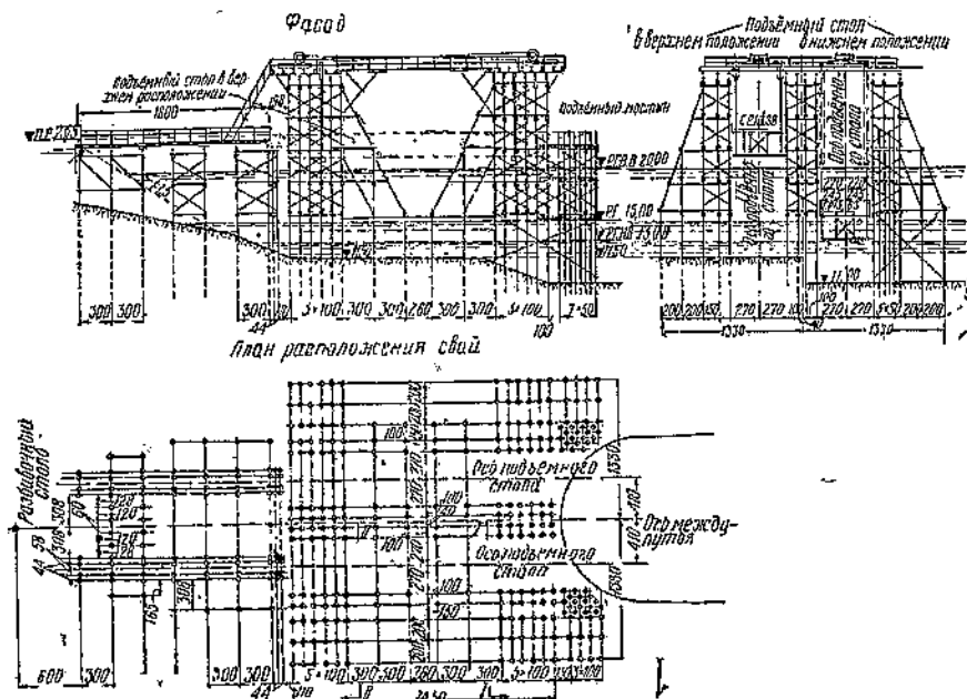
Фиг. 14. Береговой механический подъемник для передачи вагонов с берега на паром
