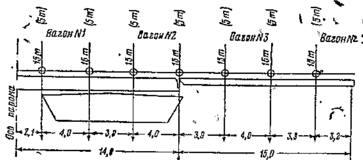
Фиг. 89. Расчётная схема загрузки спаренного паромы
