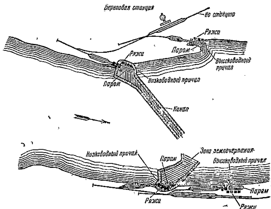
Фиг. 7. План расположения ряжевых причалов и береговых станций переправы продольного типа
