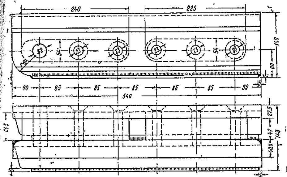
Фиг. 69. Переходный рельсовый составной башмак (вес 40 кг)
