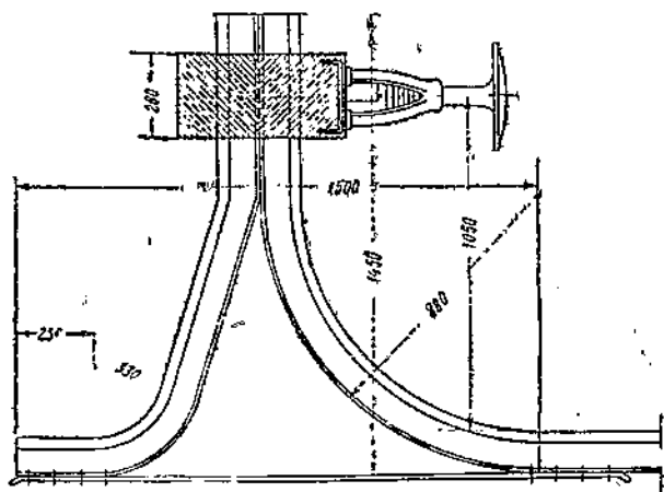
Фиг. 53. Упор для парома с продольными путями
