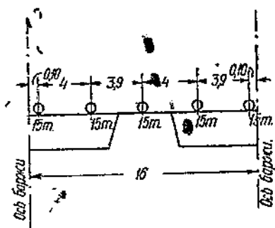
Фиг. 94. Расчётная схема загрузки поперечной надстройки
