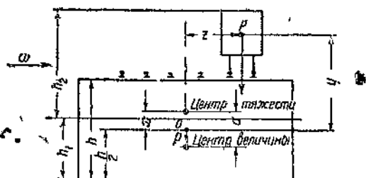
Фиг. 86. Расчётная схема загрузения для вычисления крена паромов откуда
