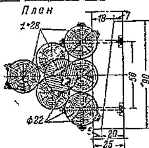
Фиг. 23. Свайный одиночный причальный куст
