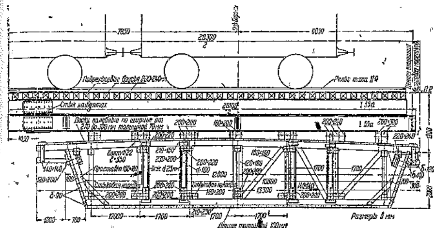
Фиг. 44. Поперечный разрез деревянного спаренного паромы с металлической надстройкой
