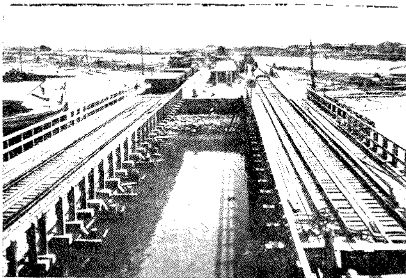
Фиг. 11. Двухпутная стационарная эстакада
