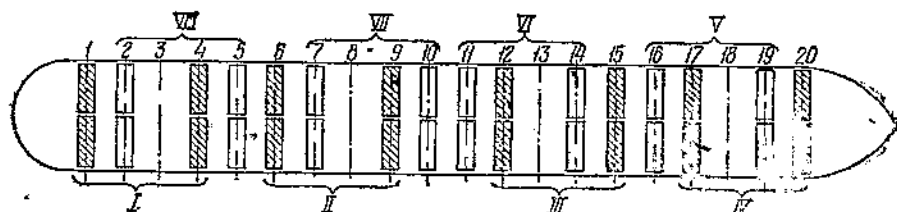
Фиг. 77. Схема загрузения парома с 20 поперечными путями
