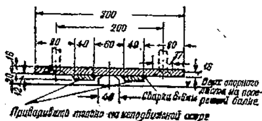
Фиг. 63. Опирание деревянного пакета на поперечную балку
