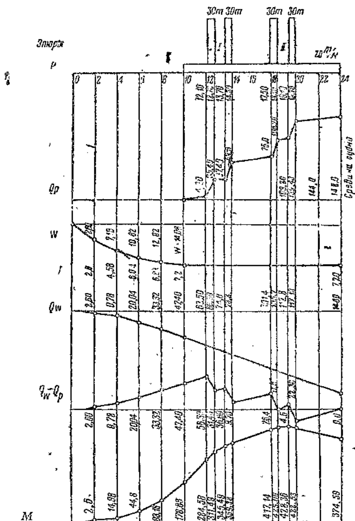
Фиг. 90. Эпюры изгибающих моментов и поперечных сил в корпусе судна при загрузке парома 12 вагонами
