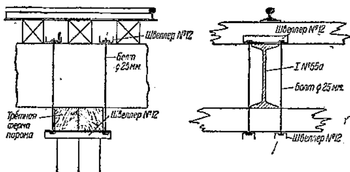
Фиг. 49. Скрепление металлической проезжей части с корпусом деревянного парома
