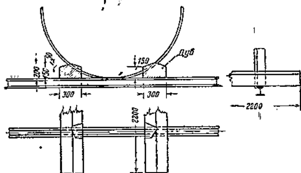
Фиг. 54. Передовые тормозные брусья
