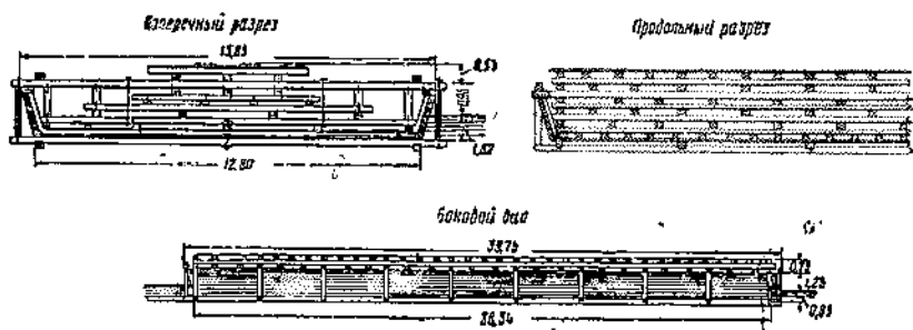
Фиг. 79. Баржа для зимней переправы
