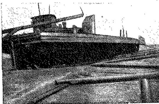
Фиг. 73. Вытаскивание баржи на берег для ремонта черепового бруса
