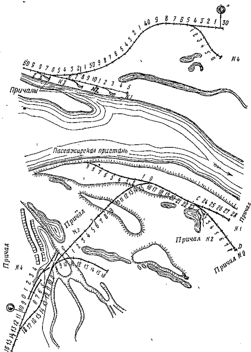
Фиг. 4. План расположения причалов переправы через Волгу у Свияжска
