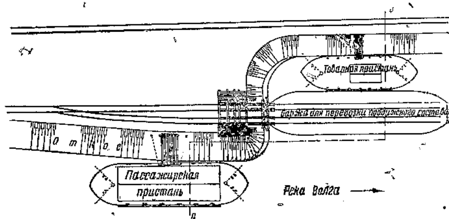
Фиг. 2. План причала переправы через Волгу у Свияжска
