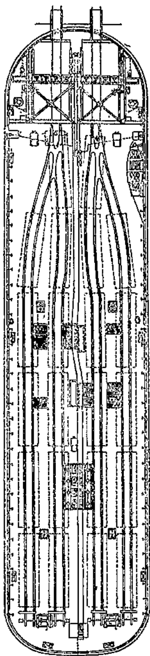
Фиг. 29. Паром «Саратовская переправа» (план верхней палубы)
