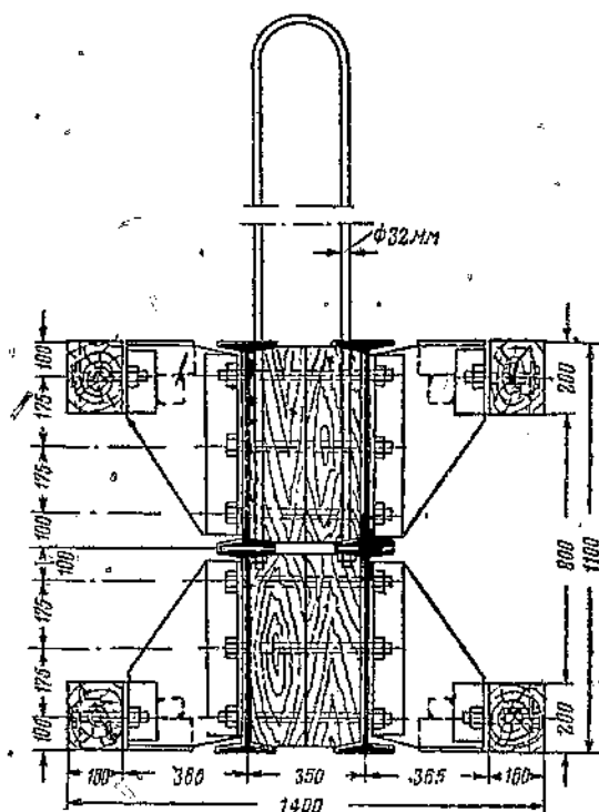
Фиг. 61. Подъемная поперечная балка и скоба для подвешивания
