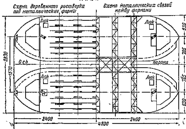
Фиг. 43. Спаренный деревянный паром с пятью поперечными путями
