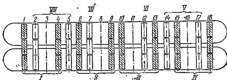
Фиг. 76. Схема загрузки парома с 18 поперечными путями
