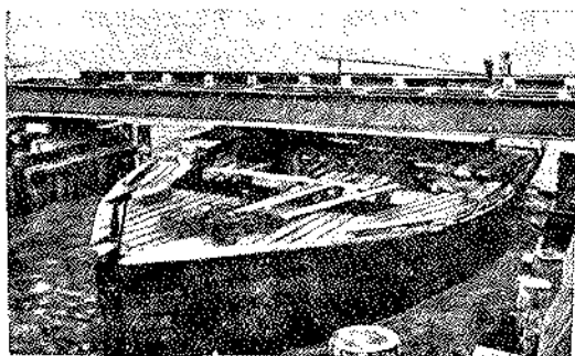
Фиг. 75. Доставка готовых пакетов на барже и установка в пролёте
