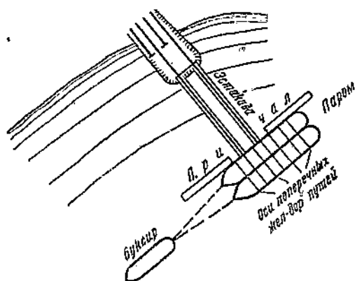
Фиг. 1. Паром с поперечным накатом подвижного состава
