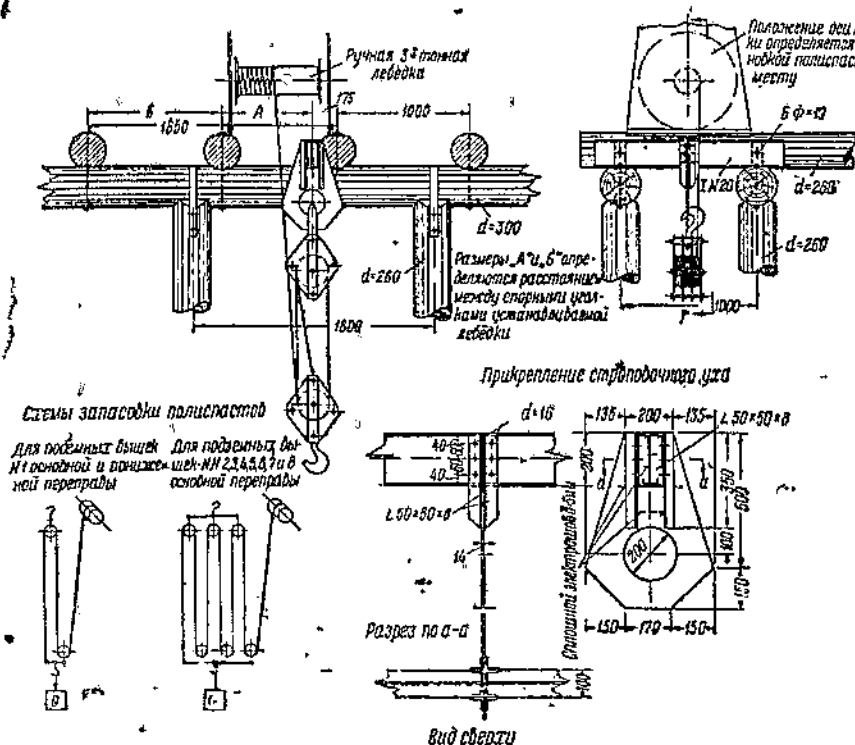
Фиг. 59. Приспособления для подъёма мостиков
