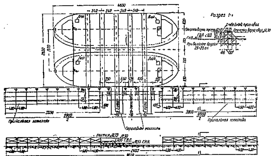
Фиг. 22. Причальная пристань переправы поперечного типа
