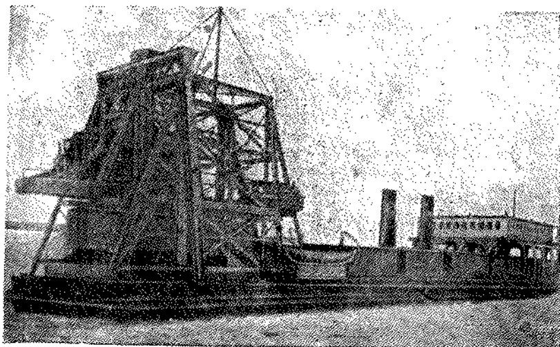
Фиг. 33. Самоходный паром «Переправа вторая»
