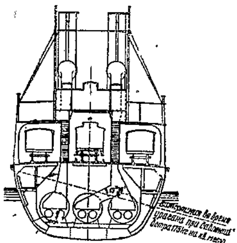
Фиг. 36. Паром-ледокол «Байкал» (поперечный разрез по средней части)
