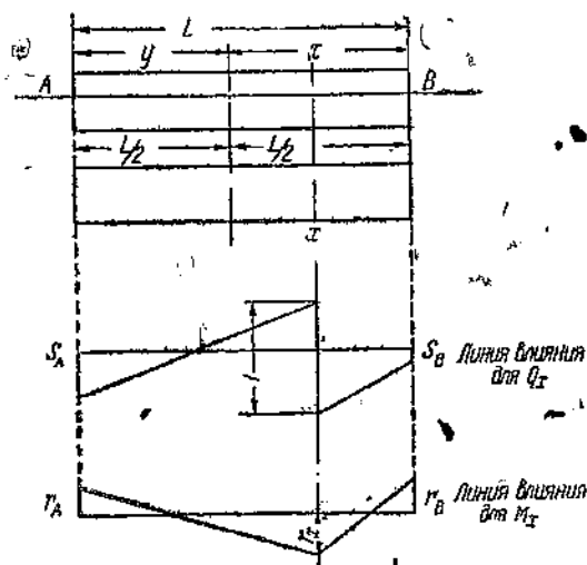
Фиг. 87. Линия влияния для поперечной силы и момента
