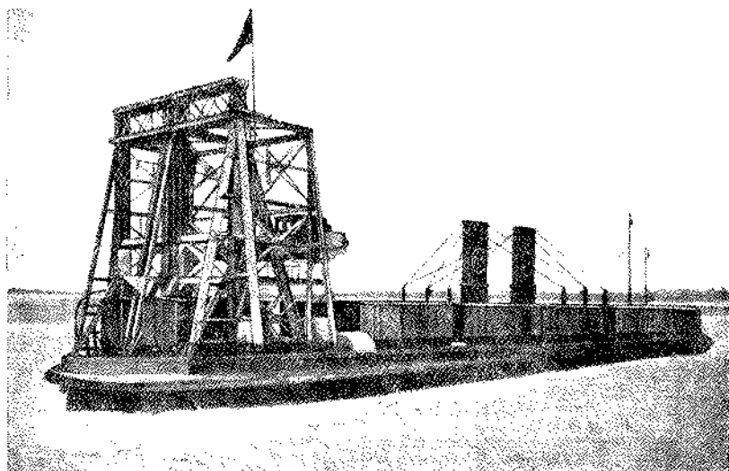
Фиг. 13. Самоходный паром «Саратовская переправа»
