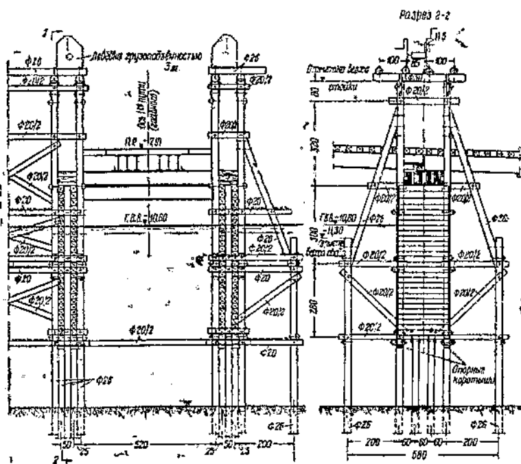
Фиг. 58. Подъемные вышки, мостики и закладные брусья
