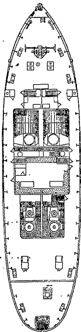
Фиг. 32. «Саратовский ледокол» (план верхней палубы)
