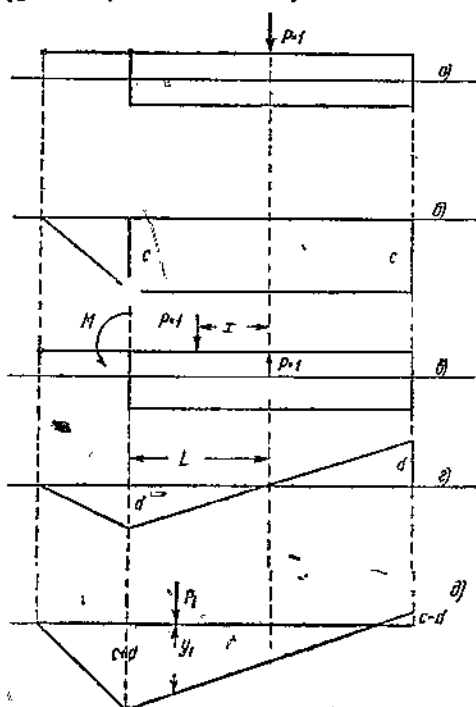
Фиг. 85. Линия влияния осадки паром
