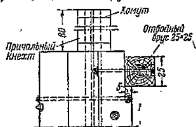
Деталь отбойного куста свай и отбойного бруса
