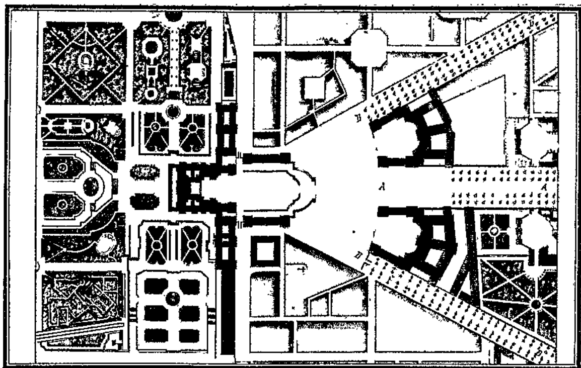
197. Версаль. Большой дворец и Площадь Армии (по Блонделю): А—А—Парижский проспект; Б—Б—проспект Сен-Клу; В—В—проспект Со
