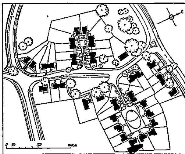
283. Город-сад Уэльвин. Планировка кварталов и жилых улиц. На плане — тупики, обстроенные домами-коттеджами
