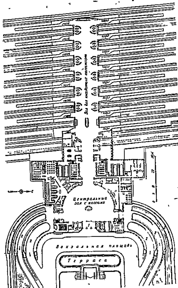
264. Цинциннати (США). План центрального вокзала. Вокзал расположен над путями железных дорог и тоннелями-завездами для городского транспорта: 1 — вестибюль; 2, 2 — заезды для автомобилей; 3 — петля для рельсового транспорта. Авторы проекта — Феллгеймер и Вагнер
