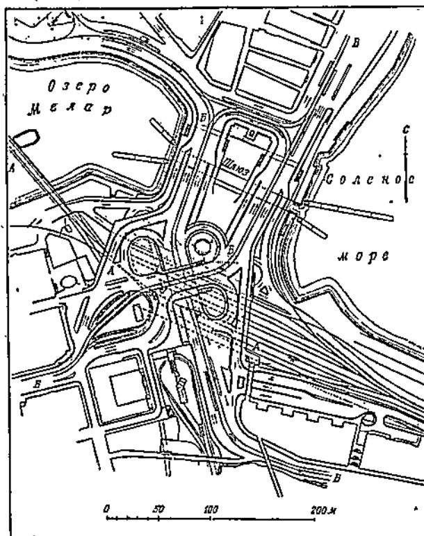
263. Стокгольм. Развязка движения в пункте пересечения главной улицы и железнодорожного диаметра: А—А—главные железнодорожные пути; Б—Б—направления наиболее напряженных потоков городского движения
