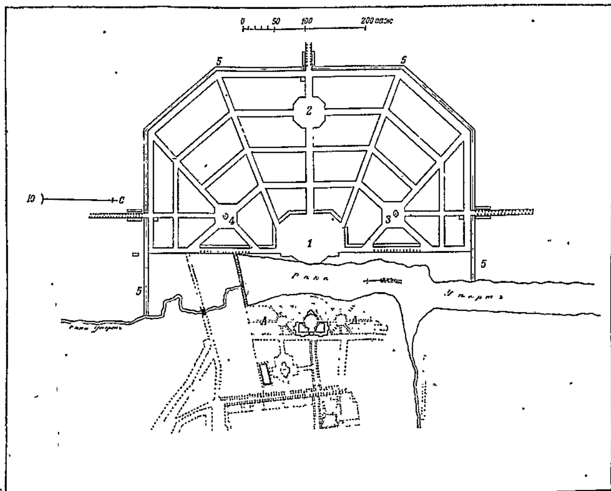
249. Богородицк (планировка города произведена в 1778 г.):
