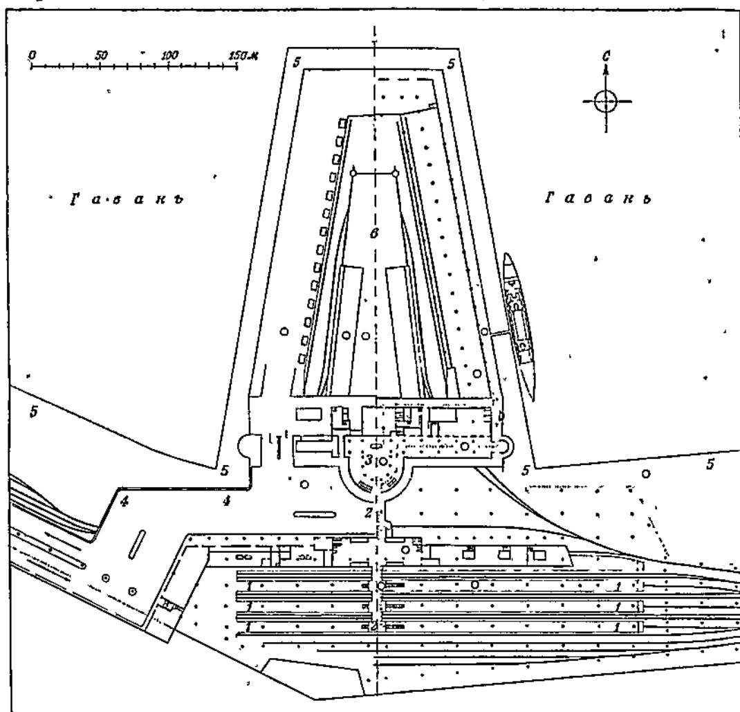
315. Алжир. План комбинированного железнодорожного и морского вокзала: 1—1 — пассажирские железнодорожные платформы; 2—2 — переход на уровне 2-го этажа; 3 — вестибюль вокзала; 4—4 — терраса-набережная для городского автомобильного движения; 5—5 — причальная набережная; 6 — внутренний товарный двор
