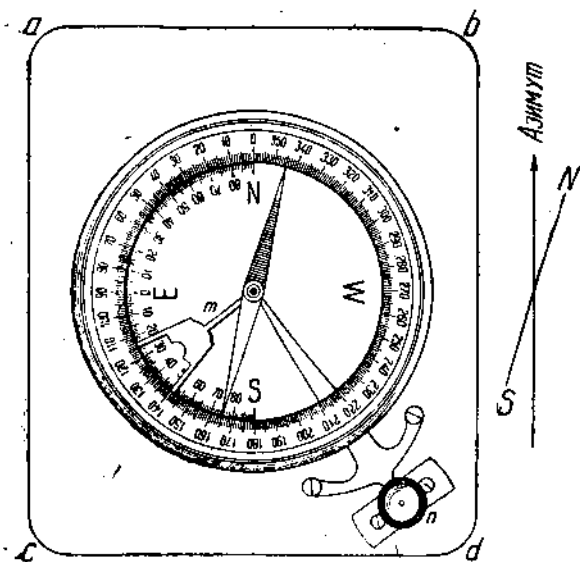
Рис. 28. Горный компас.
