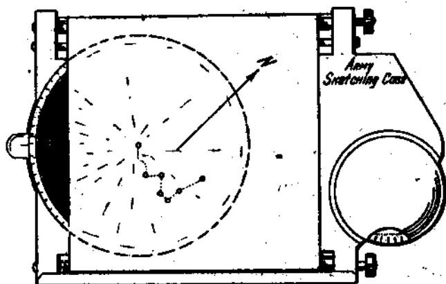
Рис. 36. Американский прибор для нанесения глазомерной съемки.
