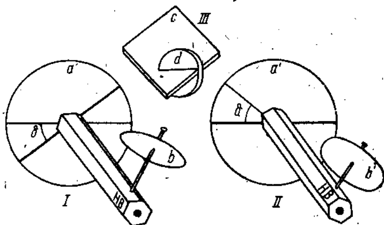
Рис. 79. Прибор для определения первоначального наклона гальки в нарушенных пластах (Бурачка). a, a' — диск в плоскости падения пласта, b, b' — диск наклона гальки, \angle \delta — угол падения пласта. I — диск b в нарушенном положении, II — диск b' в первичном положении, III — c пласт, d плоскость гальки.
