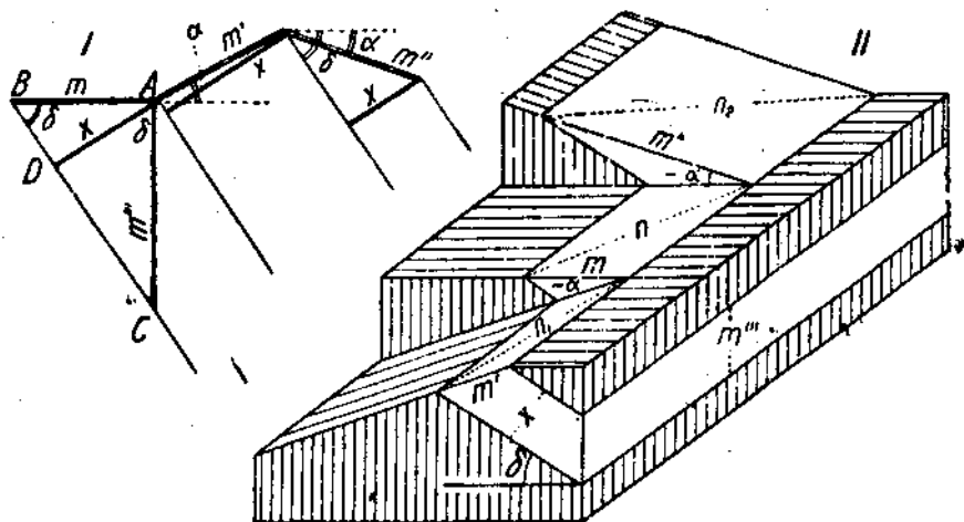
Рис. 134. Измерение мощностей при различных случаях: I — измерение вкрест простирания; II — блок-диаграмма различных случаев.
