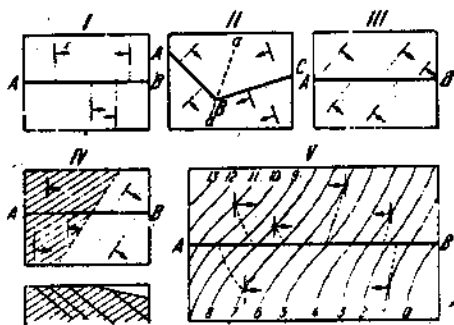
Рис. 94. Различные случаи направления геологического разреза.
