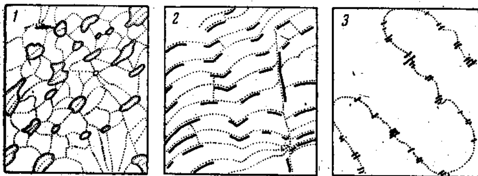
Рис. 38. Три способа расположения маршрутов при геологической съемке: 1 — оконтуриванием обнажений, 2 — съемкой по простирацию, по контактам, 3 — маршрутно, вкрест простираения. Пунктир — маршруты.
