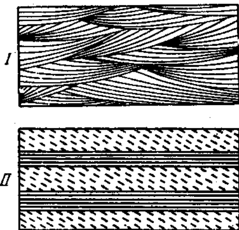
Рис. 56. Косослоистость золовая — I и временных потоков — II.
