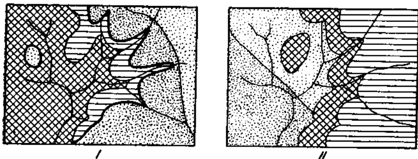
Рис. 23. Слева — старая свита (точки) надвинута на молодую (штриховка), жирная линия — разрыв. Справа — молодая свита (штриховка) несогласно налагает на старую (точки).
