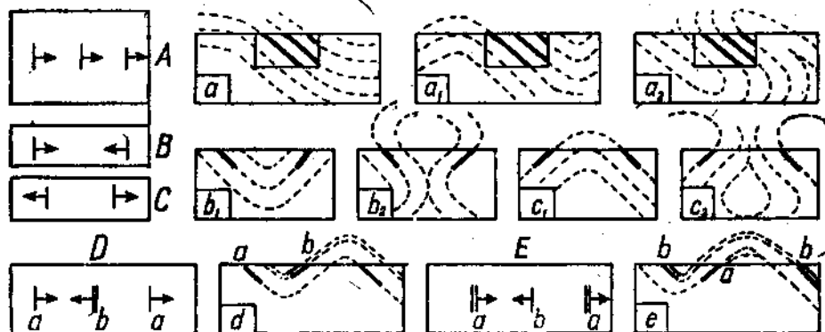
Рис. 103. Различная трактовка данных для разреза: большие буквы — карты, маленькие — разрезы (по Lahee).
