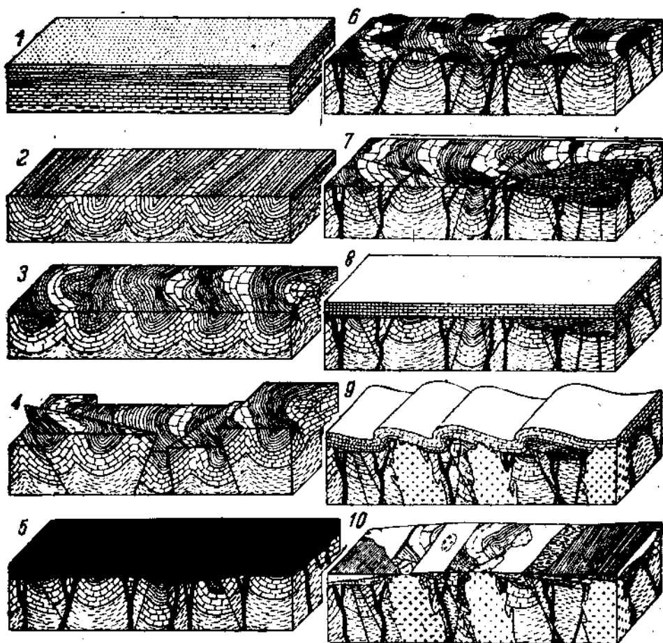
Рис. 120. История геологического развития южной части средней Сибири от середины протерозойской эры до нижне-силурийской эпохи включительно. В блок-диаграммах от 1 до 6 — протерозой, 7 — нижний кембрий, 8 — средний кембрий, 9 — верхний кембрий, 10 — нижний силур (по Чуракову).
