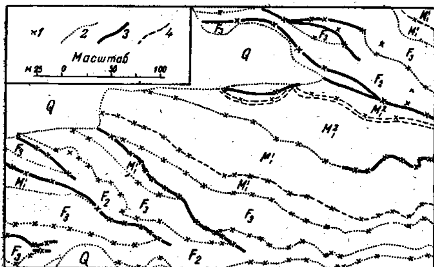
Рис. 45. Пример инструментальной съемки по простираанию. 1 — пункт стояния рейки; 2 — нормальная геологическая граница; 3 — тектонический контакт; 4 — опорный пласт; Q — нанос; M_1^1 , M_1^2 , F_1 , F_2 , F_3 — различные горизонты палеогена.
