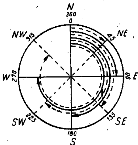
Рис. 31. Азимуты отсчитываются по часовой стрелке.
