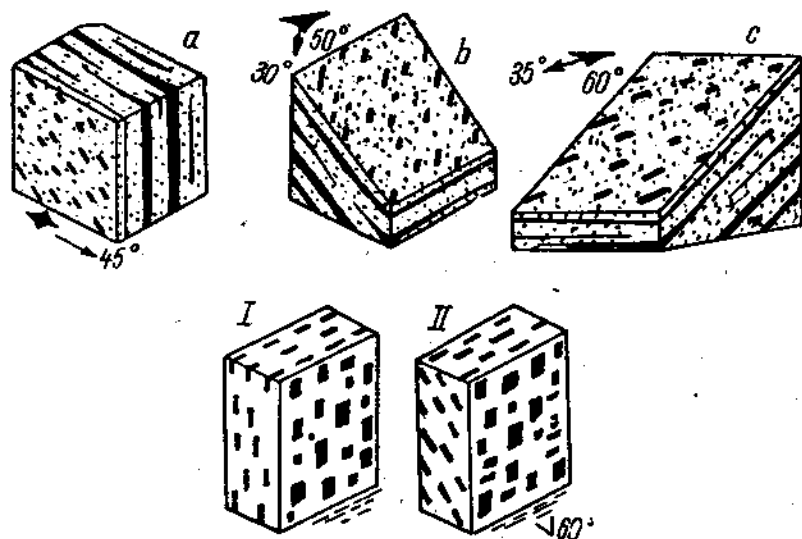
Рис. 46. a, b, c — полосатая (или шлировая) текстура (черные полосы) и линейные элементы (черные черточки); a — вертикальная, линейные элементы пад. \angle 45^\circ , b — под углом в 50^\circ , лин. элем. пад. \angle 30^\circ , c — под углом 60^\circ , лин. элем. пад. \angle 35^\circ . I и II — флюидальное расположение табличчатых минералов; I — вертикальное и II — под углом 60^\circ (внизу значки).
