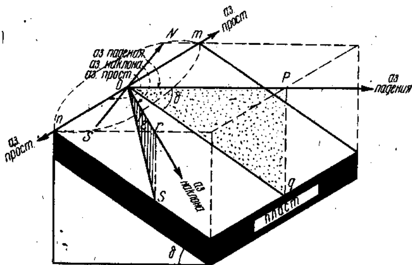
Рис. 72. Элементы залегания пласта: ml — простираение пласта (азимуты простираения: Om на SE и Ol — на SW); OP — азимут падения; \angle POq — угол падения ( \delta ); Or — азимут одного из наклонов пласта; \angle rOS — угол этого наклона ( \alpha ). По левой кромке диаграммы показаны отсчеты азимутов концентрическими дугами. Плоскость падения — в точках, плоскость наклона пласта — заштрихована.
