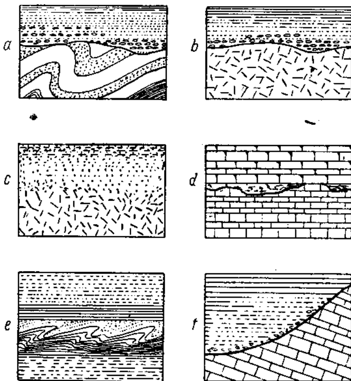
Рис. 57. a и b — угловое несогласие, c — скрытое несогласие, d — параллельное несогласие, e — местное несогласие, f — прислоненные пласты (несогласное прилегание).
