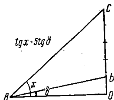
Рис. 100. Определение угла падения в преувеличенном вертикальном масштабе: \delta — угол падения, \angle x — искомым.
