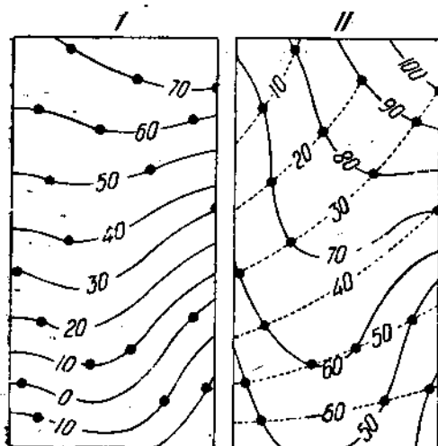
Рис. 116. Построение подземного рельефа картой схождения: II — сплошные линии — горизонталь опорного горизонта, пунктирные — изохоры; на пересечениях — точки горизонталей искомого горизонта в кратных 10 числах; I — искомые горизонталы.
