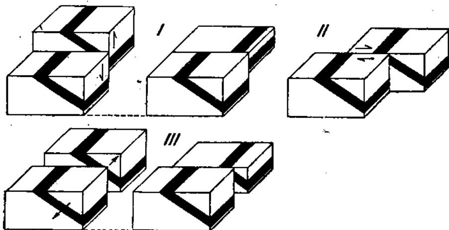
Рис. 19. Одинаковый результат (на карте, справа) при различных направлениях перемещений: I — вертикальном, II — горизонтальном и III — диагональном.
