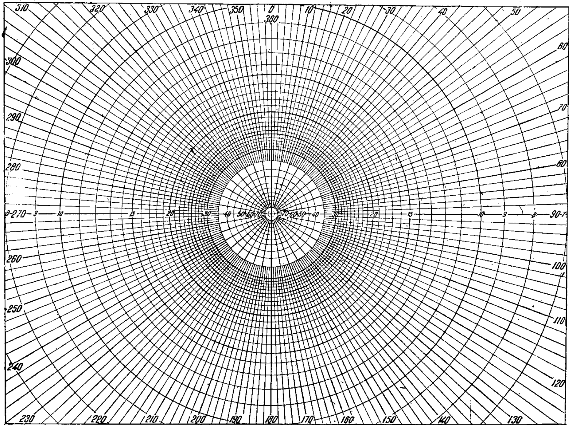
Рис. 129. Сетка Баумана. Радиусы — азимуты направлений наклонов, круги — углы наклонов пласта.
