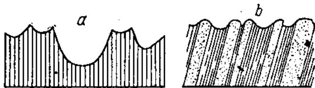
Рис. 53. Желоба растворения — а и дифференциальное выветривание — б (в разрезе).
