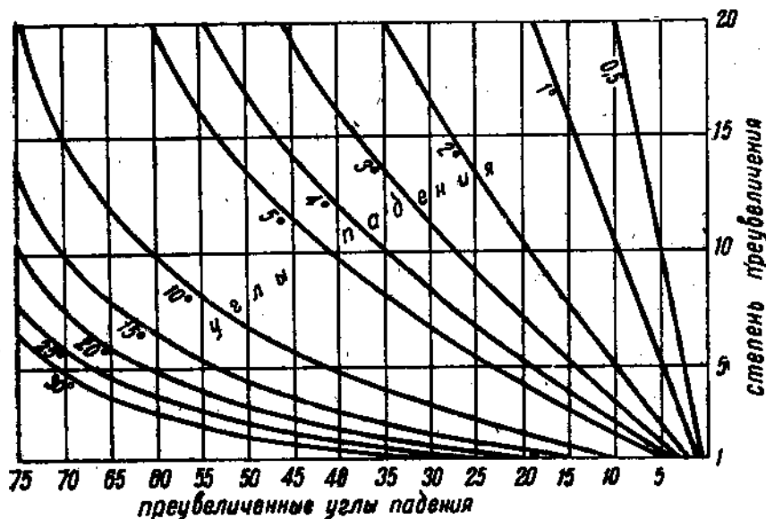
Рис. 99. Диаграмма соотношений истинных углов падения (кривые), преувеличенных на разрезе углов (абсциссы) и степени увеличения вертикального масштаба (ординаты).
