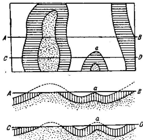
Рис. 11. В направлении AB на карте не отобразилась антиклиналь, видная в сечении CD . Сверху—карта, внизу — разрезы по AB и CD .
