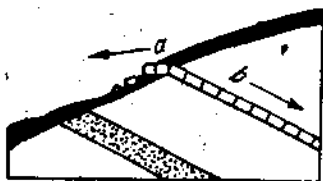
Рис. 78. Ложное падение (а) на склоне.
