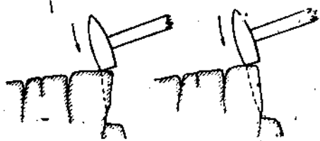
Рис. 84. Отбивание образца. Заштрихована кора выветривания.
