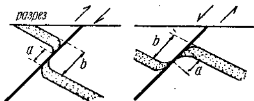
Рис. 140. Завороты пластов при сбросах: a — видимая амплитуда передвижения, b — истинная.
