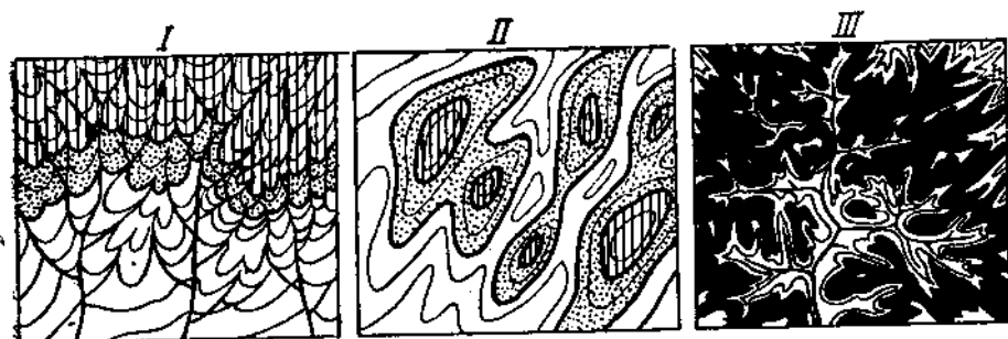
Рис. 5. Границы горизонтальных отложений на карте.
