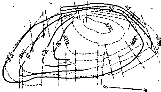
Рис. 124. Подземный рельеф (пунктир) пласта песка и температурные градиенты (жирные линии) в футах на 1° F (Salt Creek Dome, Wyoming, упрощенный чертеж из Lane).
