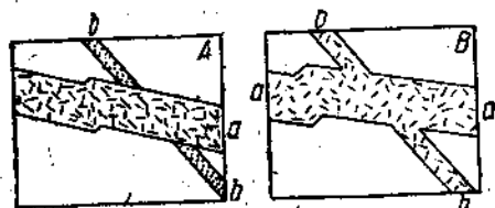
Рис. 68. А — дайка a моложе b . В — обе дайки одного возраста.
