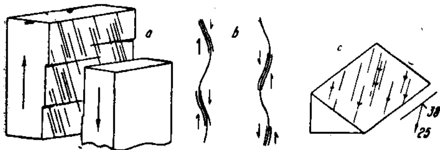
Рис. 54. Признаки направления движения крыльев на сбрасывателе: а — по уступам, б — на волнистых поверхностях, с — по выбоинам.
