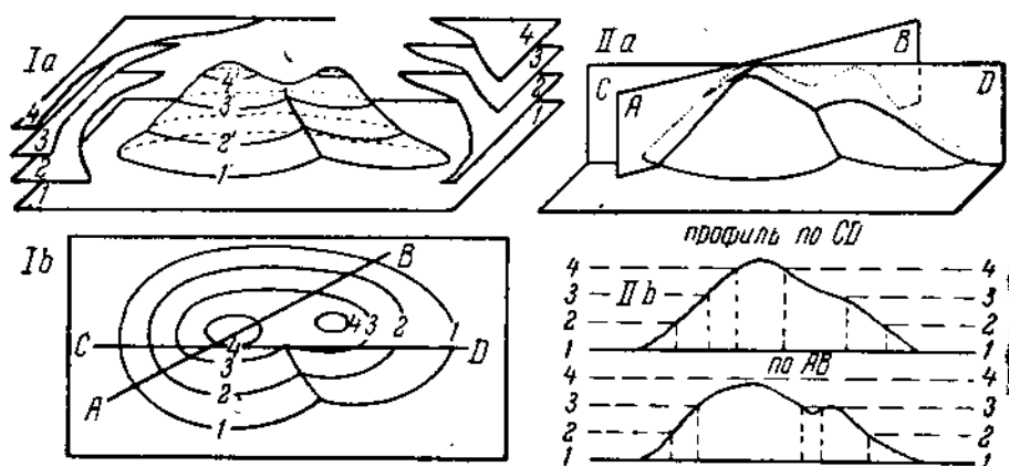
Рис. 1. Топографическая карта в горизонталях и профили. Ia — гора с двумя вершинами, рассеченная четырьмя горизонтальными плоскостями 1, 2, 3 и 4, Ib — карта в горизонталях, IIa — та же гора, рассеченная двумя вертикальными плоскостями AB и CD , IIb — профили по этим сечениям.
