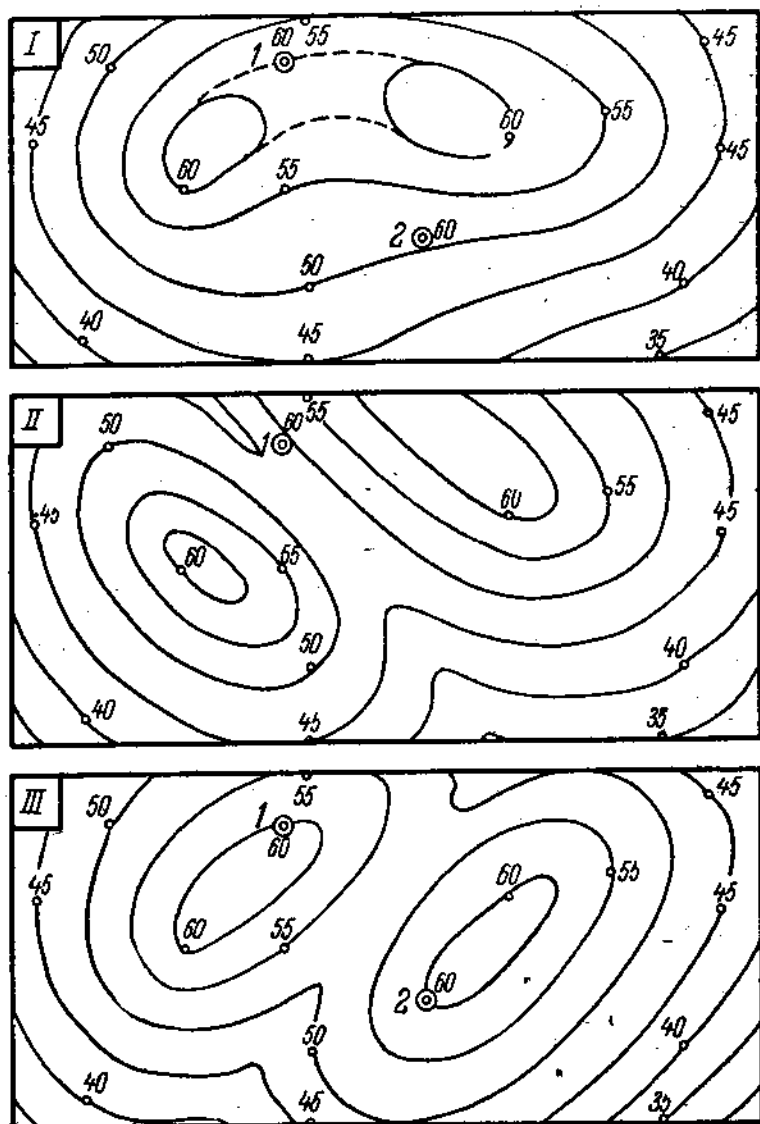
Рис. 113. Три варианта подземного рельефа по отметкам пласта в одинаковых 14 скважинах. После проведения 15-й скважины (№ 1, двойной кружок) отпал вариант II, после проведения 16-й скважины (№ 2) отпал вариант I, остается наиболее вероятным вариант III (см. рис. 114).
