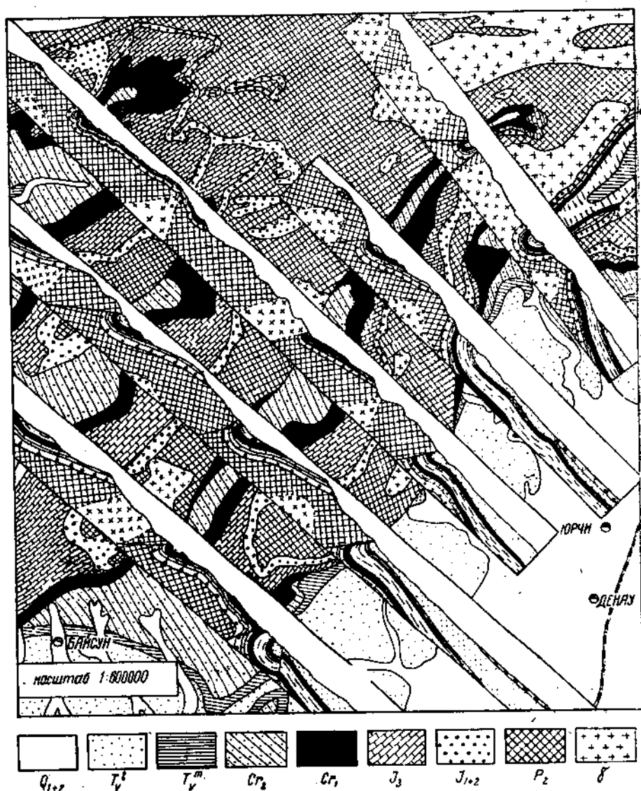
Рис. 104. Расположение разрезов по американскому методу по вырезам в геологической карте (по Чуенко).
