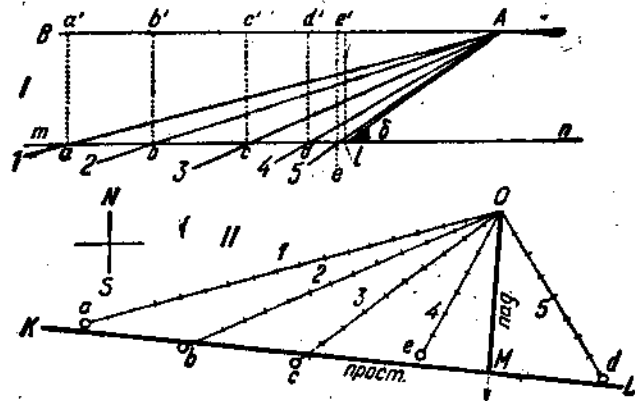
Рис. 130. Определение залегания по нескольким углам наклона неровной поверхности пласта.
