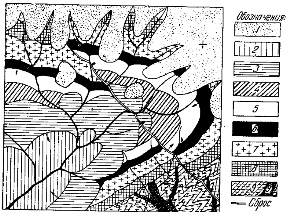
Рис. 24. Геологическая карта с несогласиями и разрывами.
