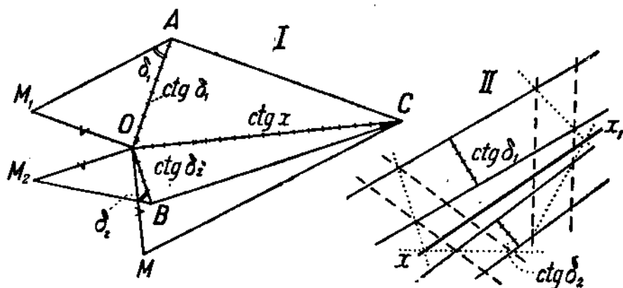
Рис. 139. Нахождение проекции пересечения двух плоскостей.
