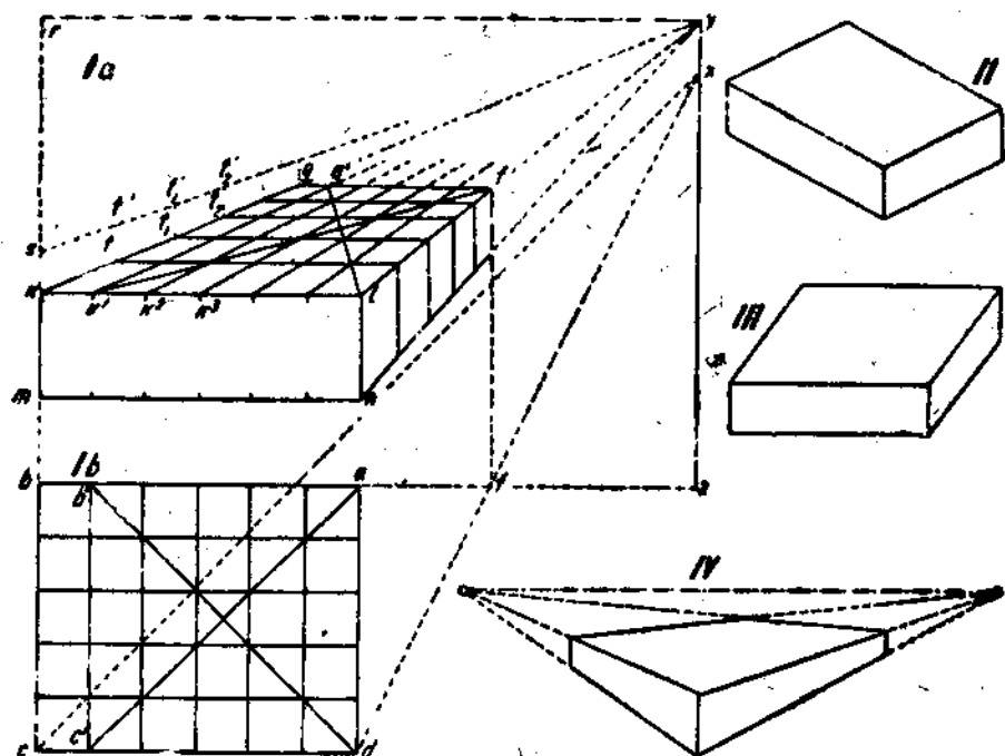
Рис. 119. Построение блок-диаграммы (I) и различные виды блок-диаграмм (II—IV).
