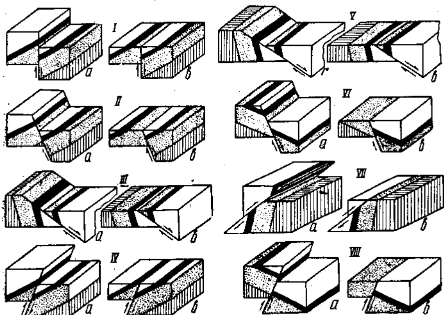
Рис. 16. Влияние продольных разрывов на „выпадение“ и „удвоение“ свит на поверхности (справа—b—после смыва поднятого крыла).
