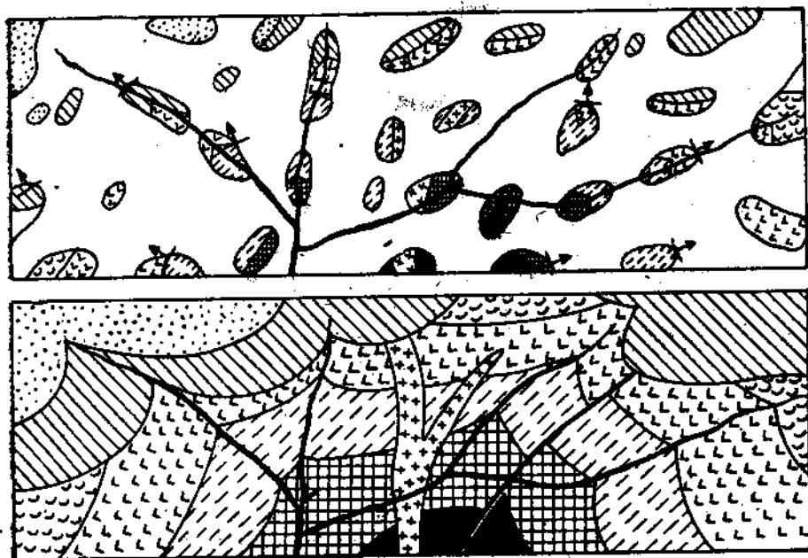
Рис. 40. Съемка оконтуриванием обнажений. Внизу геологическая карта.
