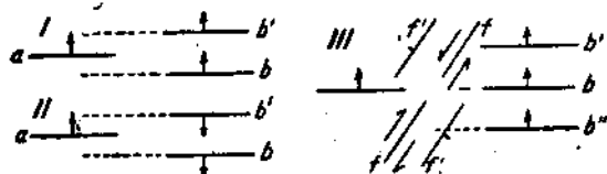
Рис. 30. Значение взаимного расположения обнажений.
