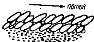
Рис. 55. Расположение плоской гальки в потоке.
