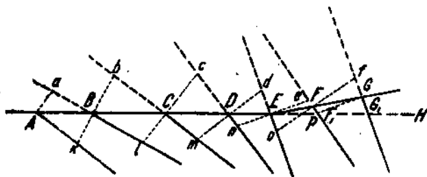
Рис. 111. Определение мощности свиты при изменчивом ее падении. Разрез вкрест простирания (по Hayes).
