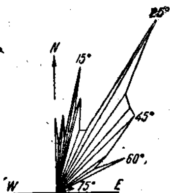
Рис. 49. Роза-диаграмма числа различных простираний трещин Q .
