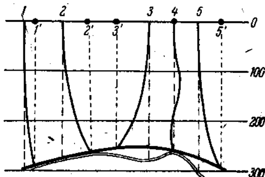
Рис. 123. 1, 2, ... 5 — устья искривленных скважин, 1', 2', 3' и 5' — точки, к которым должны быть отнесены результаты бурения. Жирная линия — исправленный разрез, двойная — неисправленный.
