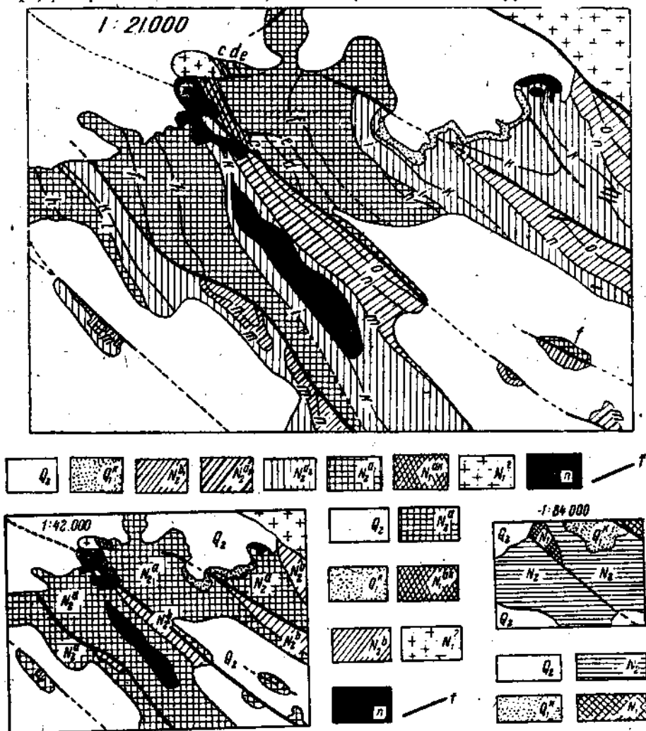
Рис. 93. Геологическая карта части о. Челекена в трех масштабах (1:21000, 1:42000 и 1:84000). Легенды: Q_2 — аллювий, Q_1^A — древне-каспийские отложения, N_2^a — бакинский ярус, N_2^b — апшеронский ярус ( a_1 — нижний, a_2 — средний, a_3 — верхний), N_1^a — акчагыльский ярус, N_1^b — красноцветная толща, p — кировые покровы, f — сбросы. Нижняя легенда: N_1 и N_2 — неоген.
