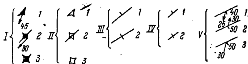
Рис. 47. Обозначения текстуры, трещины и линейных элементов. I — 1 и 2 — см. рис. 46, a, b и c , 3 — горизонтальное расположение элементов. II — L-трещины: 1 — наклонные, 2 — вертикальные, 3 — горизонтальные. III — S-трещины: 1 — наклонные, 2 — горизонтальные. IV — то же, Q-трещины. V — борозды скольжения (черточки — падение сбрасывателя): 1 и 2 — направление движения налегающей глыбы известно (стрелка), 3 — то же, когда неизвестно.
