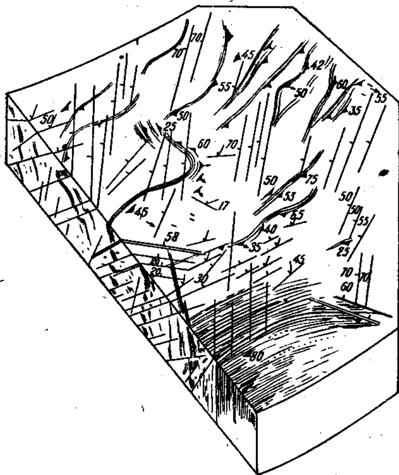
Рис. 48. Блок-диаграмма с нанесенными знаками по Клоосу (на верхней поверхности).
