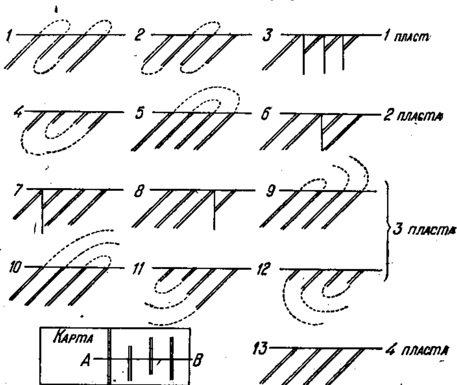
Рис. 4. Комбинации четырех сходных пластов на разрезе.
