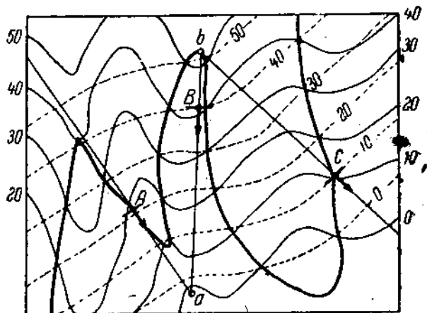
Рис. 90. Построение выхода пласта по обнажениям A, B и C с переменными азимутами и постоянными углами падения. a и b — пересечения азимутов падения и центры дуг горизонталей пласта.
