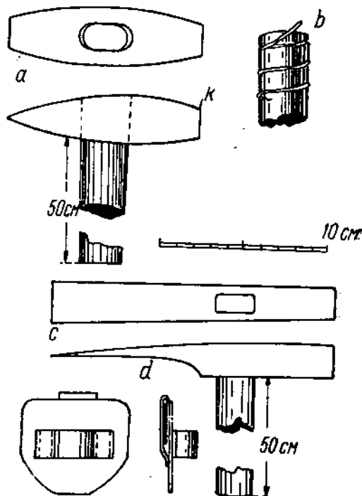
Рис. 26. Различные геологические молотки. а — златоустовский тип, с, d — кайла для рыхлых пород.
