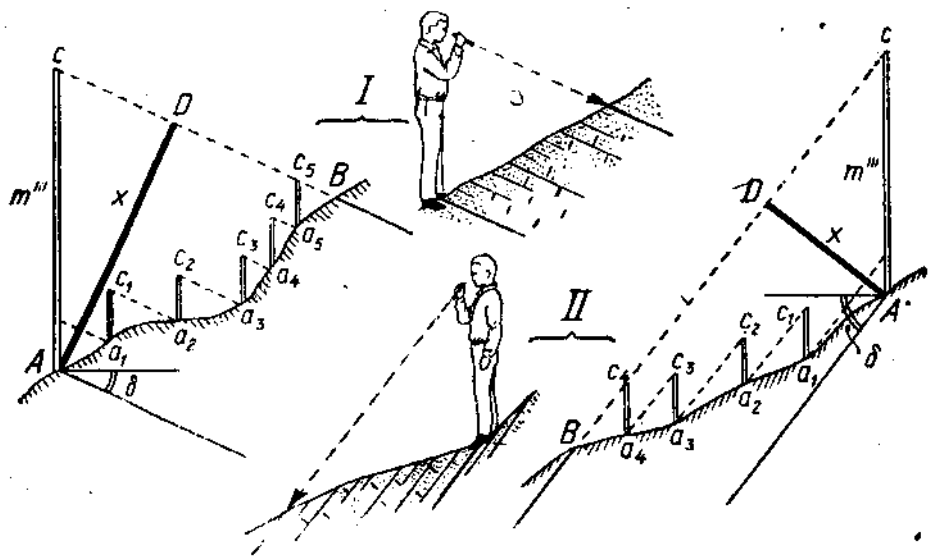
Рис. 136. Определение мощности с помощью эклиметра: I — склон обратно падению; II — склон по падению.
