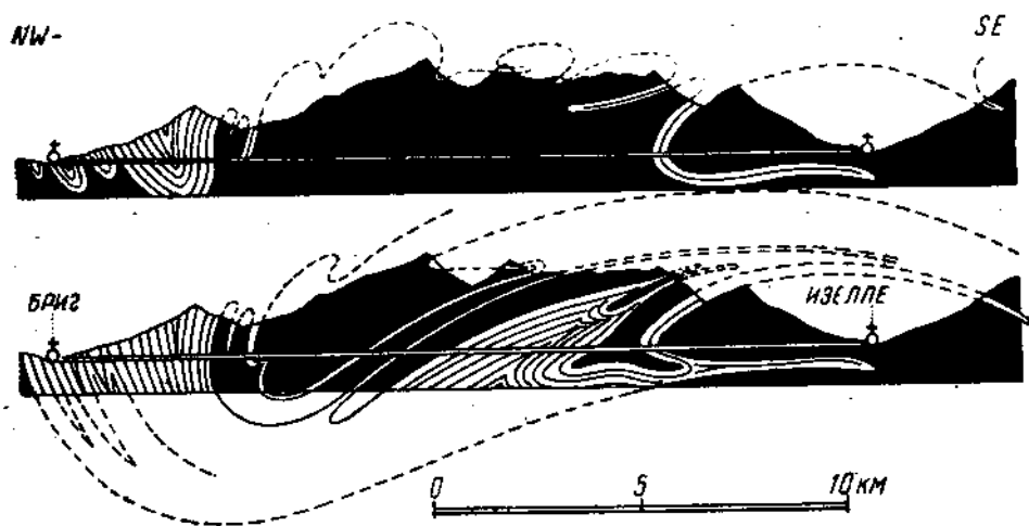
Рис. 3. Геологический разрез через Симплонский тоннель. Сверху старое толкование, снизу (после проведения тоннеля) — новое. Черное — гнейсы, белое — триас и юра.
