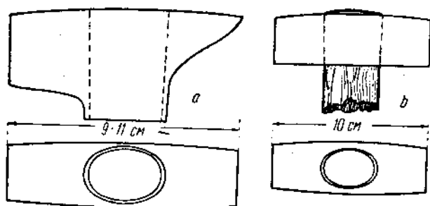
Рис. 27. Молоток с длинным отверстием (а) и с двумя плоскими бойками (b).
