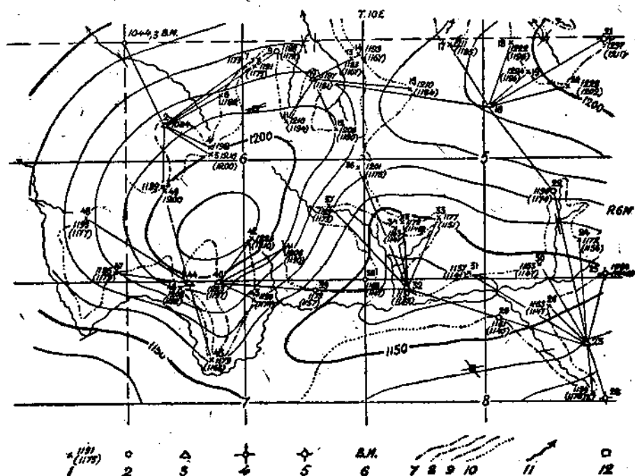
Рис. 44. Структурная карта, полученная мензульной съемкой. Горизонталы подземного рельефа пласта (изобаты) показаны сплошными контурами с сечением через 10 фут. Прочие условные обозначения: 1 — пункт стояния рейки; сбоку высотные отметки данного обнажения (без скобок) и пересчитанные на пласт, по которому составляется структурная карта (в скобках); 2 — пункт стояния рейки для прямого и обратного отсчетов; 3 — пункт стояния нивсрунта; 4 — угол участка; 5 — буровая скважина; 6 — репер; 7—10 — линии выхода на поверхность пластов (7 — пласт, по которому составляется структурная карта; 8, 9 — стратиграфически более высокие пласты; 10 — предполагаемая линия выхода); 11 — ручей, русло оврага; 12 — строения.
