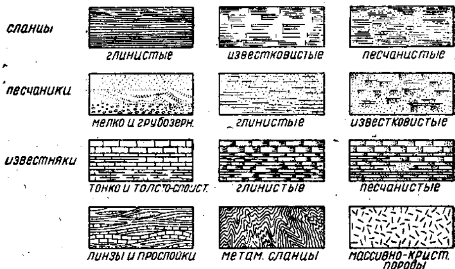
Рис. 101. Американская литологическая легенда колонок и разрезов.
