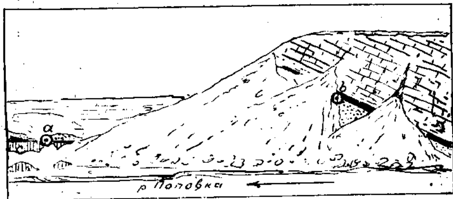
Рис. 80. Измерение мощности унгулитового песчаника на р. Поповке по случайному направлению.
