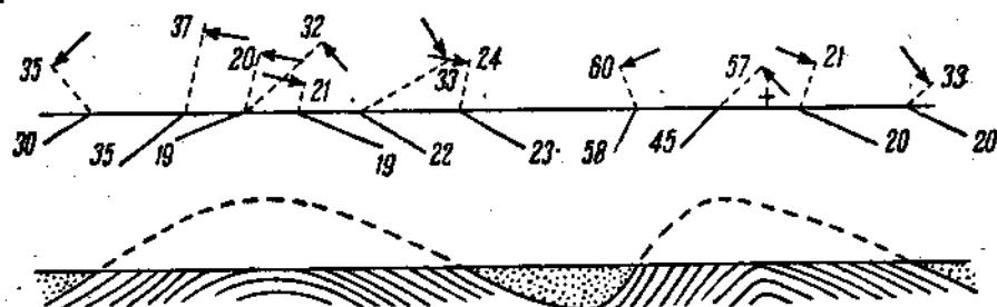
Рис. 106. Перенесение на линию разреза выходов, не приходящих на нее (в зависимости от простирания и угла падения) (по Greenly и Williams).
