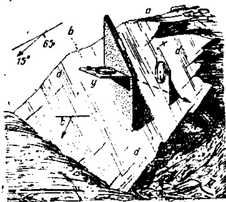
Рис. 76. Измерение на сбрасывателе борозд скольжения.
