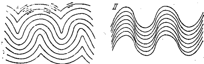
Рис. 95. Складки „параллельные“ ( I ) и „подобные“ ( II ).
