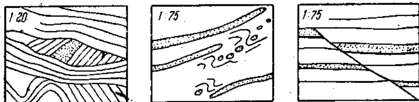
Рис. 60. Зарисовки с натуры подводных деформаций в толще глины акчагыльского яруса. Точками показаны вулканические пеплы (по В. В. Веберу).
