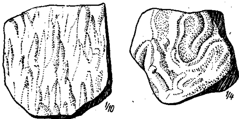
Рис. 59. Флишевые образования (гнероглифы) на песчанике (по Вассоевичу).
