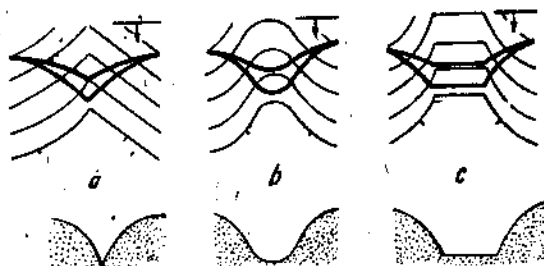
Рис. 87. Очертание выхода двух различных пластов (сверху) при пересечении долины разного сечения (снизу).
