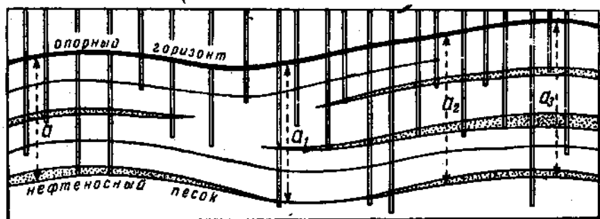
Рис. 115. Разрез свиты с переменной мощностью a , a_1 , a_2 , a_3 , пересеченной скважинами.
