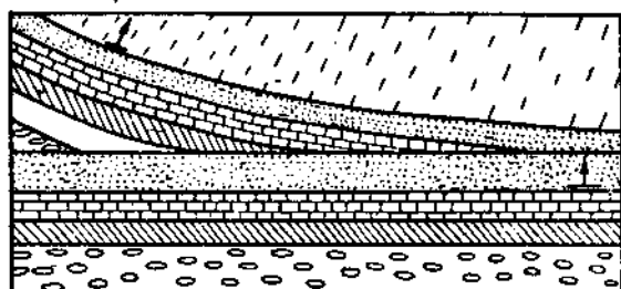
Рис. 18. Геологическая карта со сбросом, затухающим к востоку (по Мидановскому).
