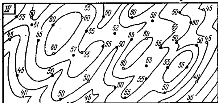
Рис. 114. Подземный рельеф того же пласта, что и рис. 113, с прибавлением новых отметок в 28 скважинах (черные кружки).
