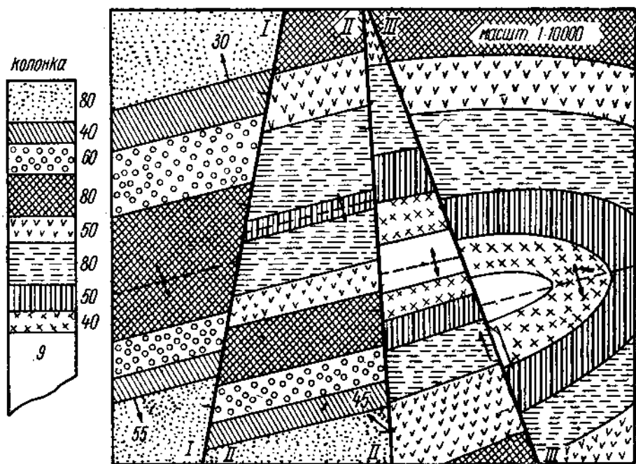
Рис. 21. Различные диагональные разрывы антиклинальной складки (оси показаны пунктиром). Справа пласты замыкаются.
