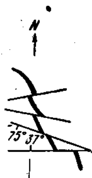
Рис. 50. Позднейшие перемещения трещин Q , заполненных жильными образованиями.
