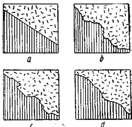
Рис. 63. Типы контактов интрузий (в разрезе): а — прямолинейный, б — зазубренный, с — глыбовый и d — волнистый.
