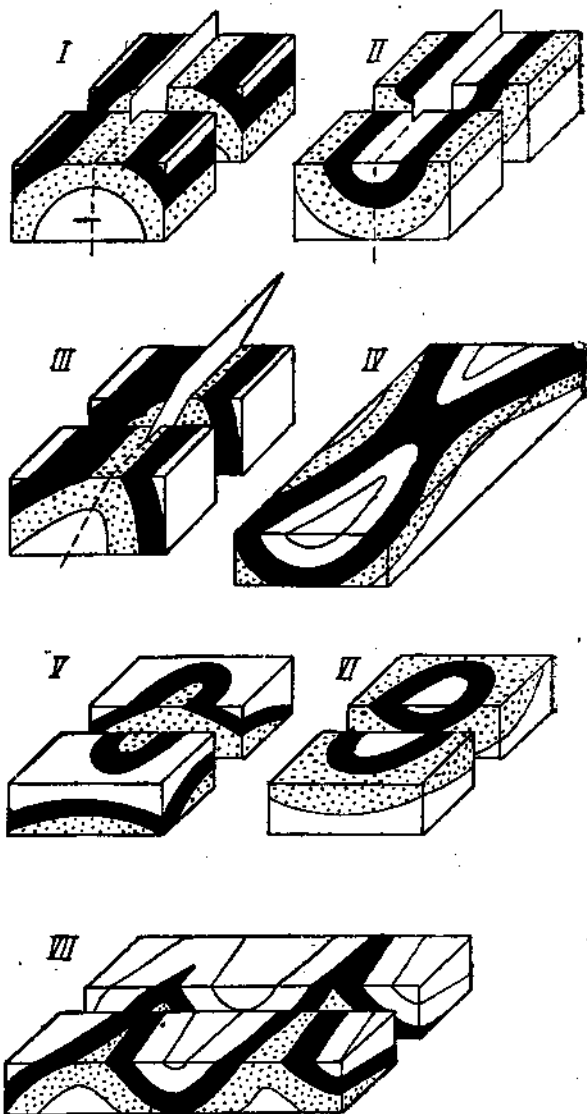
Рис. 15. Блок-диаграммы различных складок. Верхняя поверхность — карта, передняя стенка — разрез.
