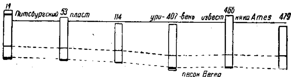
Рис. 117. Построение подземного рельефа в листе Steubenville (С. Америка): сверху — подземный рельеф опорного горизонта (сплошные линии) и изохоры (пунктир); верхние цифры — номера скважин, нижние — расстояния между двумя горизонтами; по середине — искомый подземный рельеф; внизу — разрез.
