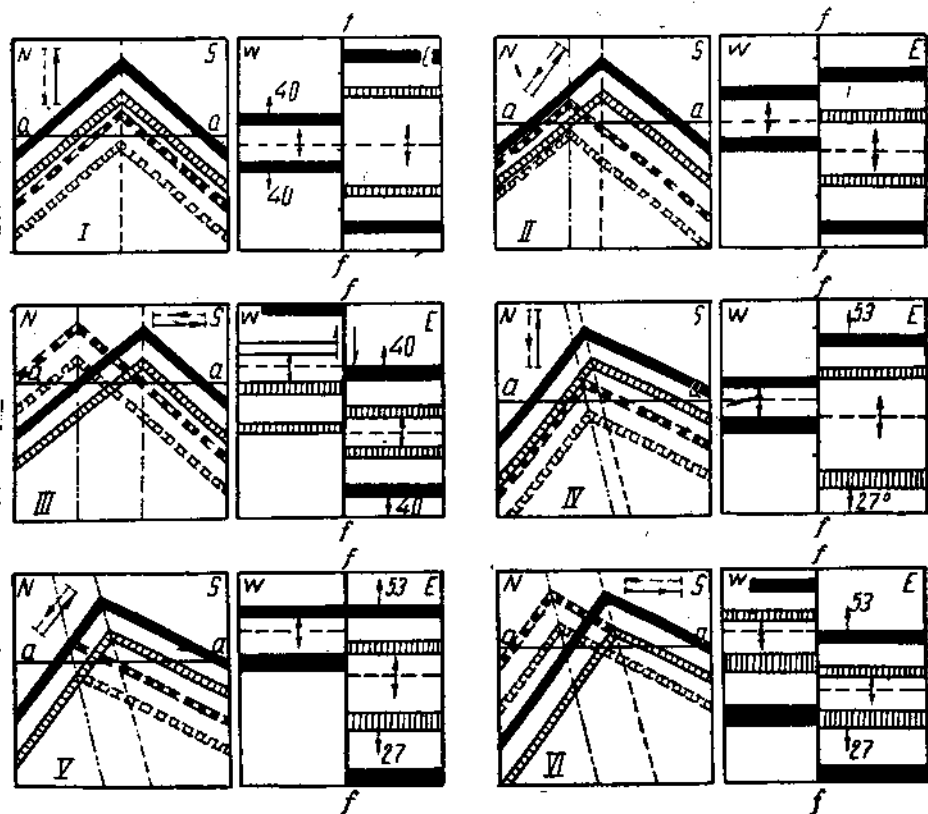
Рис. 20. Схемы различных поперечных разрывов складок. Слева — в меридиональном разрезе, справа — на карте. На разрезах показаны стрелками направление и величина передвижения. I—III — складка симметричная, IV—VI — несимметричная.
