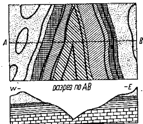
Рис. 9. Геологическая карта с симметричным расположением отложений в зависимости от рельефа (не антиклиналь). Внизу разрез.
