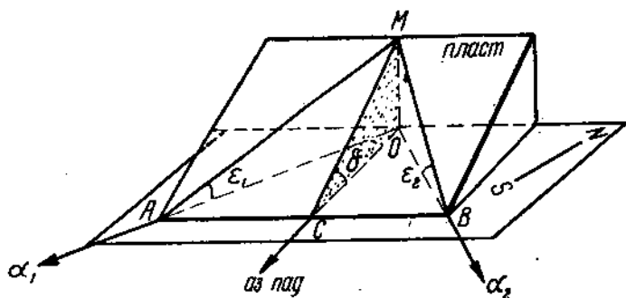
Рис. 127. Диаграмма определения залегания по двум наклонам пласта.
