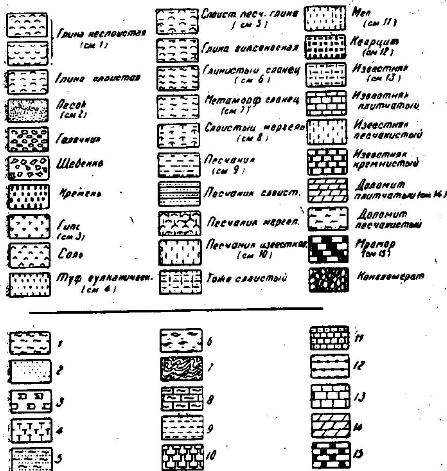
Рис. 102. Литологическая легенда для колонок и разрезов (сверху по Разумовскому, Хабакову, Малютину, снизу по Багратуни).
