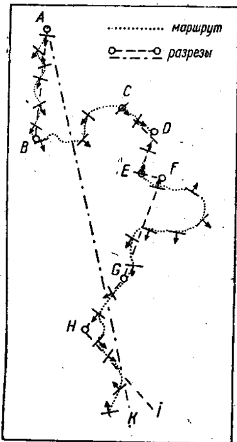
Рис. 107. Расположение линий разрезв по маршруту.
