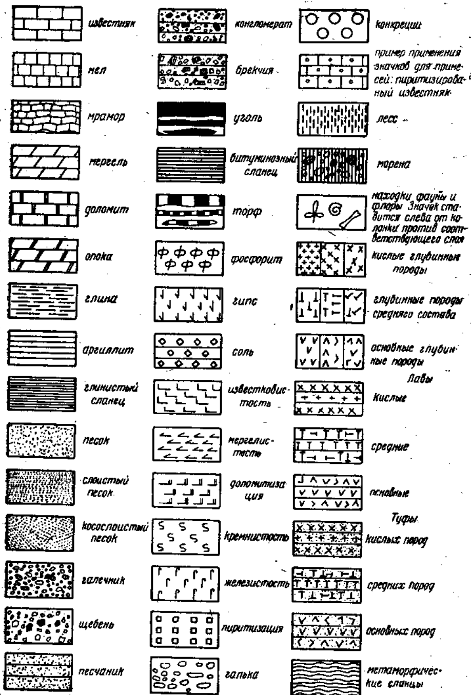
Рис. 103. Литологическая легенда для колонок (по Милановскому).
