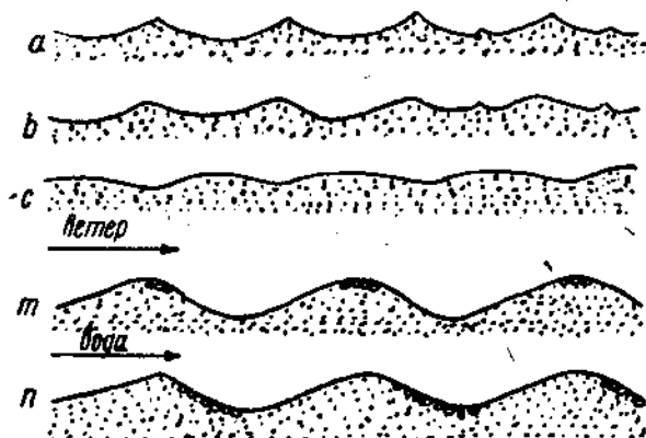
Рис. 58. Сечение ряби на поверхности песчаников. а — с — донная рябь стоячих бассейнов, m — ветровая и n — на дне потоков.
