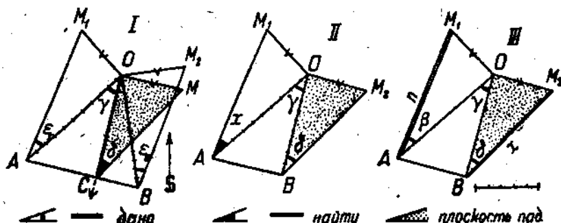
Рис. 128. I — определение залегания построением по двум углам наклона; II — определение угла в разрезе не вкост простирания; III — определение мощности по любому направлению.
