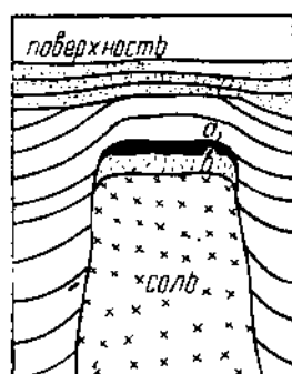
Рис. 13. Схематический разрез соляного купола. Над солью: b — гипс и ангидрит, a — галит (известник) (по Лахее).
