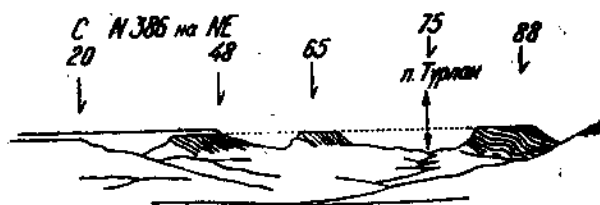
Рис. 83. набросок панорамы (поверхность пенеплена).
