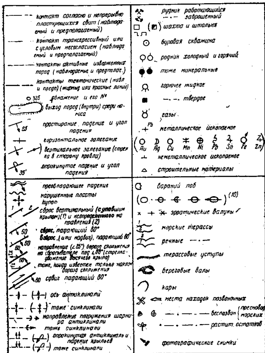
Рис. 71. Полевые обозначения. В скобках некоторые обозначения других стран.
