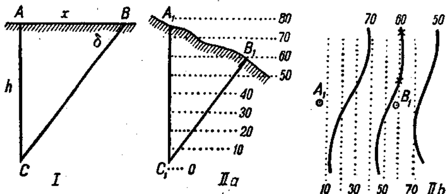
Рис. 121. Нахождение точки B на поверхности по подземной точке C . I — при горизонтальной поверхности, II — при наклонной.
