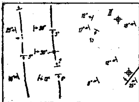
Рис. 118. I — структурная карта в горизонталях, II — то же различными значками (по Willis).
