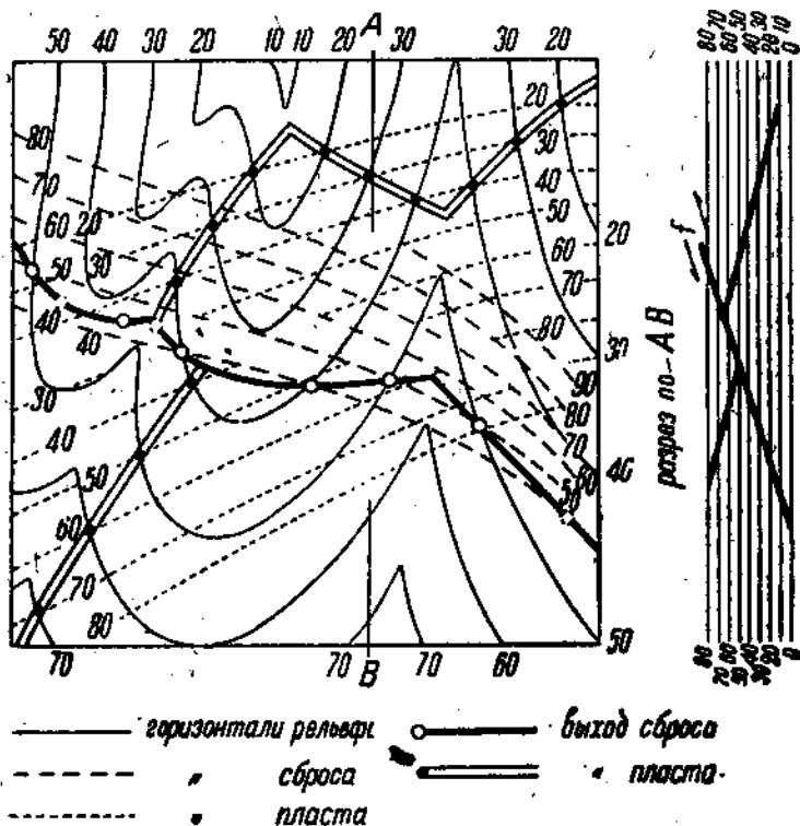
Рис. 88. Построение выхода сброса и сброшенного пласта.
