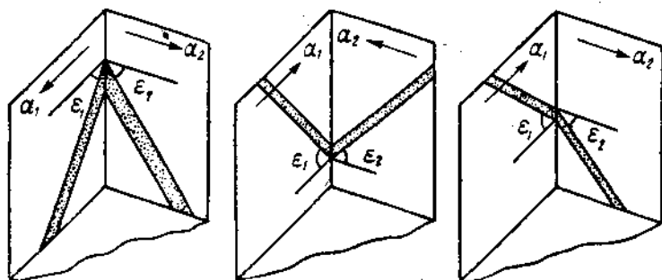
Рис. 126. Определение залегания по наклонам пласта \epsilon_1 и \epsilon_2 в шурфе; азимуты \alpha_1 и \alpha_2 берутся в направлении наклонов.
