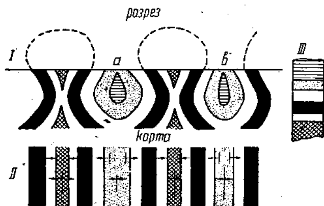
Рис. 14. Веерообразные складки. I — разрез, II — карта (показаны оси складок и падения крыльев), III — колонка.
