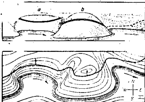
Рис. 77. Ложные складки. Сверху вид с правого берега, снизу — в плане.
