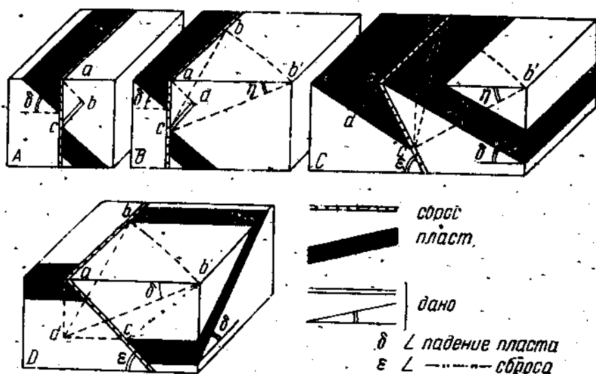
Рис. 141. Нахождение величины перемещения по разрыву.
