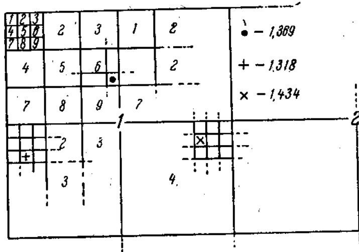
Рис. 70. Американская система фиксации точек на карте.
