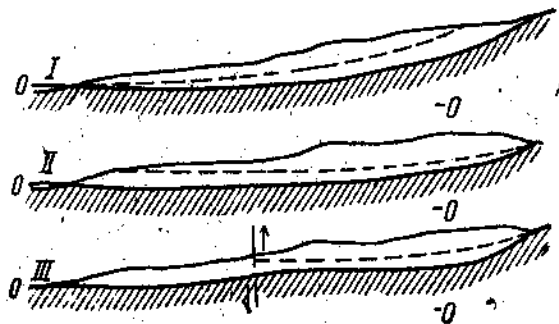
Рис. 69. Продольные профили долины. Пунктир — профили террасы.
