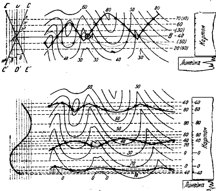
Рис. 86. Построение выхода пласта: сверху — плоскостного, внизу — цилиндрической складки с горизонтальным шарниром, слева — в разрезе. Пунктир — горизонтали пласта.
