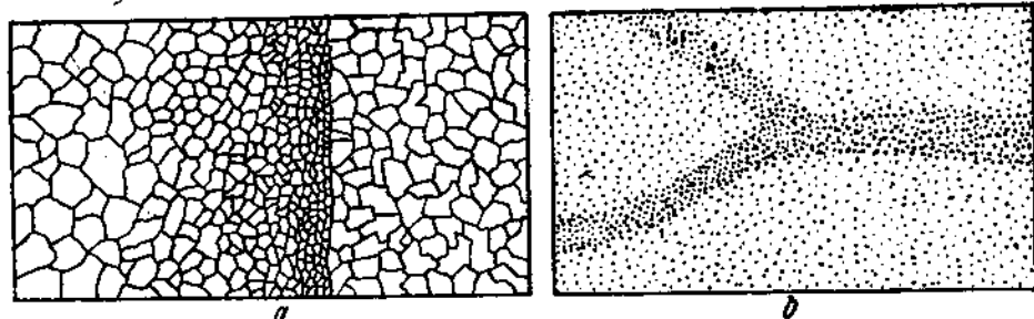
Рис. 64. а — резкий контакт двух изверженных пород; левая порода моложе, так как ее структура тонкозернистее у контакта, где кристаллизация около холодной правой породы была затруднена, б — ветвистая дайка со слепым контактом.
