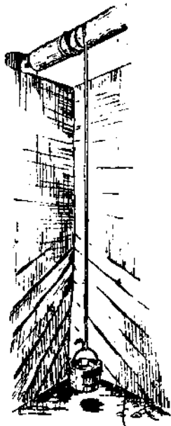
Рис. 74. Два направления наклона в шурфе.
