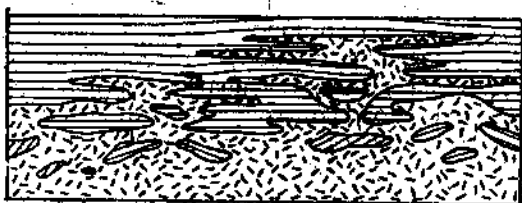
Рис. 67. Деталь контакта между сланцами (штриховка) и интрузией. Внедрение изверженной породы в сланцы легче происходило вдоль слоистости.
