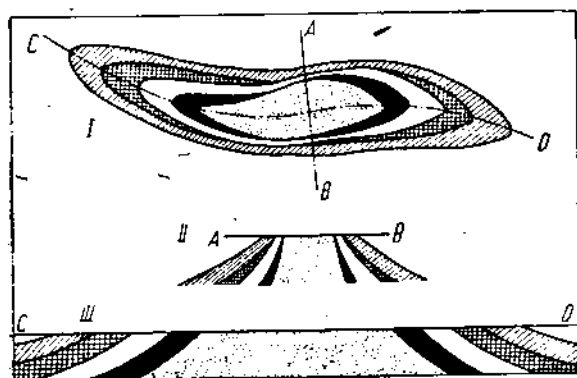
Рис. 12. Диапировая складка. Карта и разрезы по AB и CD .
