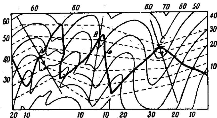
Рис. 83. Приближенное построение выхода по нескольким замерам залегания (в точках А, В и С).
