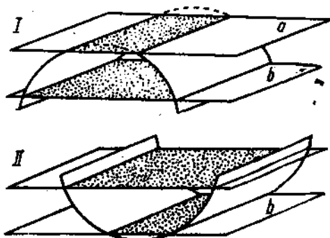
Рис. 22. Расширение полос на карте у смытого, поднятого крыла антиклинали I и обратное у синклинали II ; a — поверхность до поднятия. b — после поднятия и разрыва.
