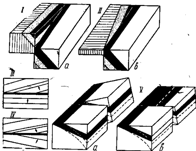
Рис. 17. Влияние затухающих сбросов (вращательных) на выходы пластов на крыльях. I—IV — продольные сбросы, V — поперечный.
