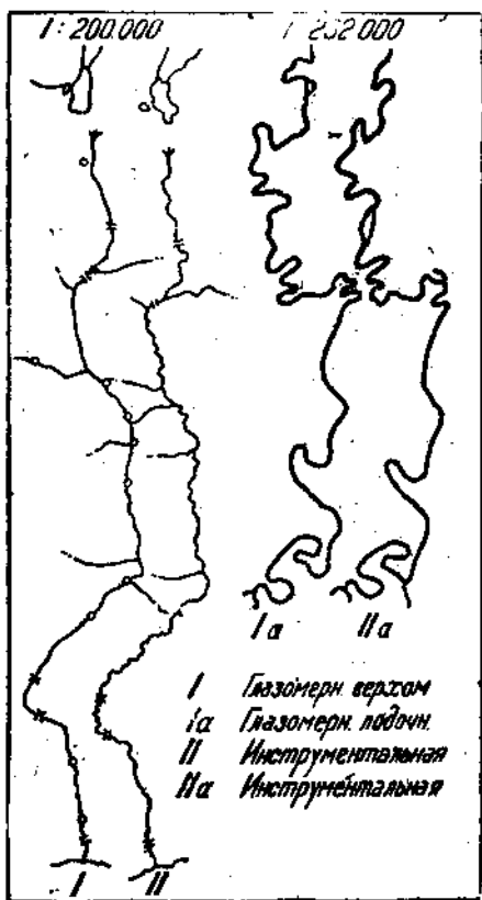
Рис. 33. Примеры глазомерных съёмок I и Ia; тех же маршрутов, снятых инструментально — II и IIa.
