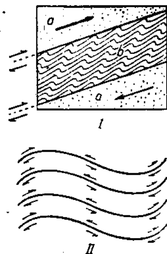
Рис. 61. I — некомпетентный пласт между двумя компетентными; II — дифференциальное движение соседних пластов при параллельных складках.
