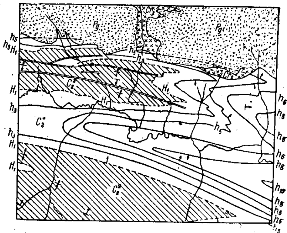
Рис. 42. Северо-западный угол Первозвановского планшета. Масштаб 1\frac{1}{2} в. в 1 д. (см. рис. 41).
