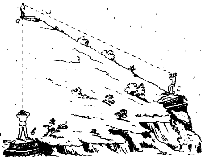
Рис. 75. Определение залегания по двум направлениям наклона ( ab и ac ).
