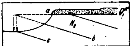
Рис. 85. Смешение фаун „проектированием“.
