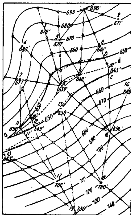
Рис. 112. Построение подземного рельефа пласта по точкам его абсолютных отметок (по Farrell).
