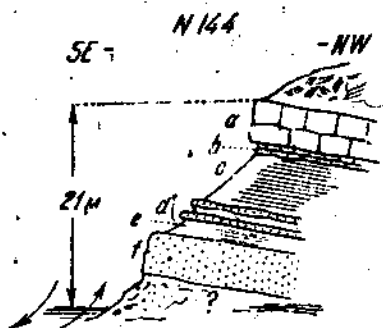
Рис. 82. Зарисовка обнажения (разрезом) на берегу реки.
