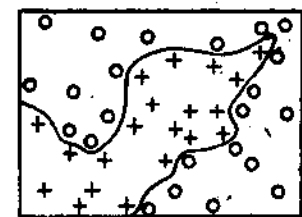
Рис. 91. Проведение границы интрузии (кресты) среди вмещающих пород (кружки).
