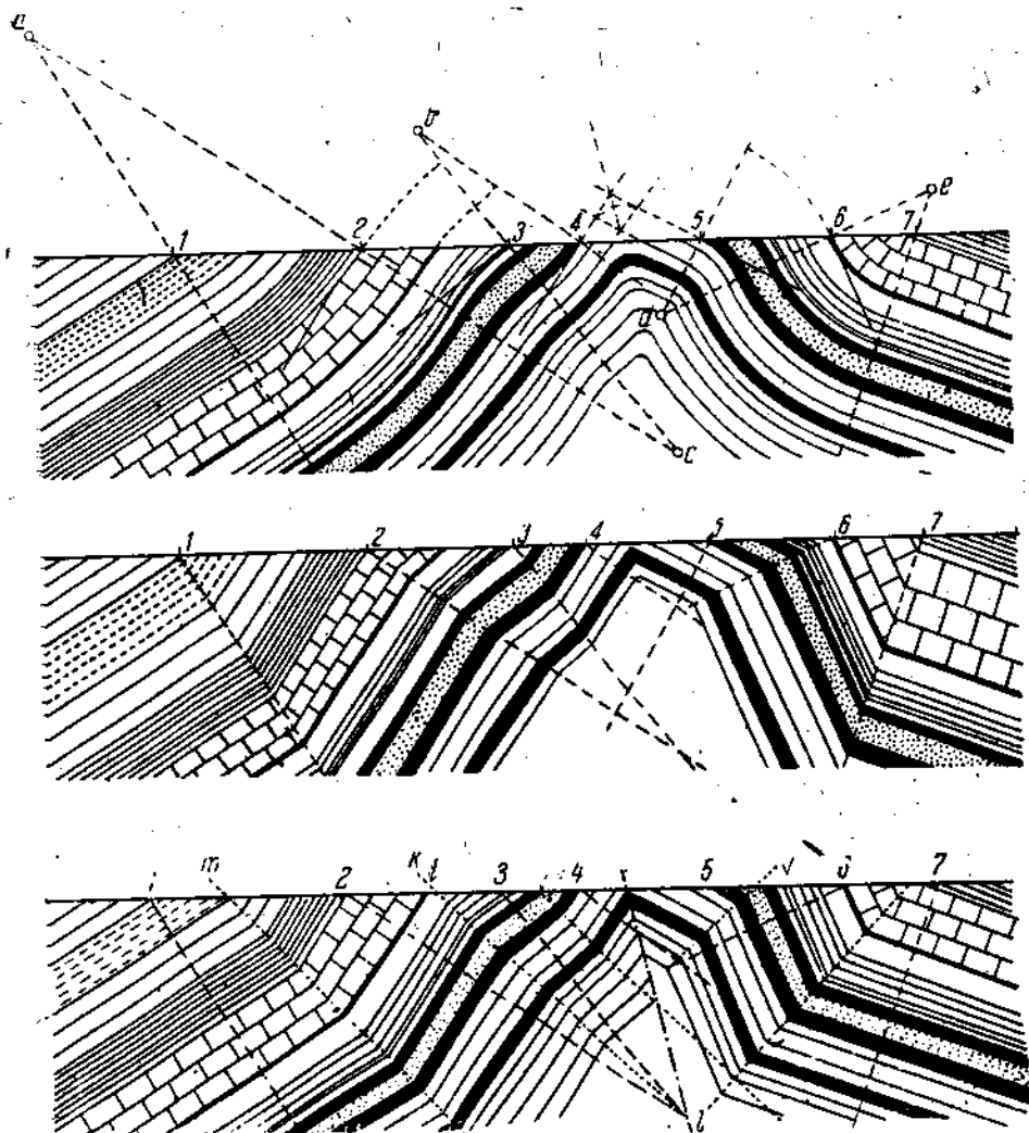
Рис. 96. Построение геологического разреза: сверху — в предположении постепенного изменения падения, посередине — в предположении, что падение меняется резко в точках измерения залегания, внизу — в предположении, что пласты меняют падение по биссектрисам ( mn , kl и др.) между перпендикулярами к линиям падений. В верхнем и нижнем построении мощности постоянны. Точки 1, 2, 3, ..., 7 — места измеренных падений.
