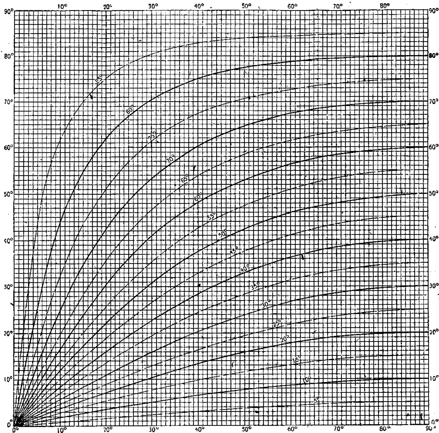
Рис. 133. Диаграмма для определения угла наклона в косвенном разрезе. Кривые — истинные углы падения; по оси ординат (сбоку) — углы в косвенном разрезе, по оси абсцисс (снизу) — углы между простиранием пласта и азимутом разреза. Например: простирание пласта NE 20°, пад. SE 110° \angle 45°, разрез проведен по NE 57°; 57 - 20 = 37 . Следя кверху по перпендикуляру 37° до пересечения с кривой 45°, находим на этом пересечении горизонтальную линию, соответствующую углу наклона пласта на разрезе \alpha = 31^\circ (по Greenly).
