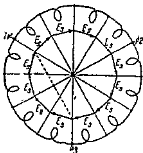
Фиг. 56. Векторная диаграмма э. д. с. E_s , индуктируемых в секциях обмотки статора синхронного генератора.
