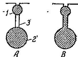
Фиг. 186. Переход от схемы Бушерио с двумя клетками к схеме с фасонными проводами В.
