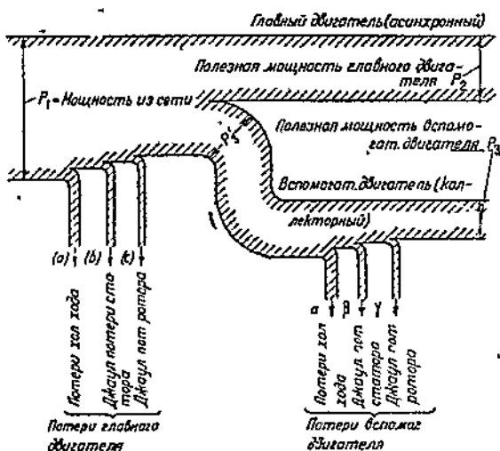
Фиг. 281. „Энергетическая“ диаграмма схемы Кримера.
