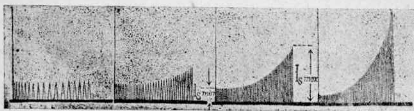
Фиг. 124. Кривые распределения плотности тока I_s по высоте провода при разных частотах ( f = 12,5; 25, 50, 100 Hz). Размеры провода 5 \times 28 mm.
