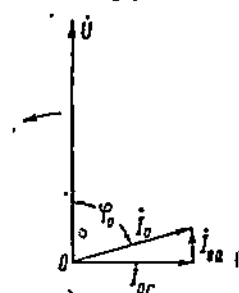
Фиг. 107. Разложение тока холостого хода I_0 на активную и реактивную I_{0r} составляющие.
