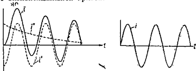
Фиг. 172. Осциллограммы тока включения.
