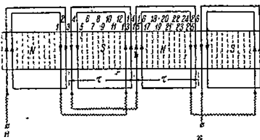
Фиг. 15. Схема однофазной катушечной обмотки ( q = 4 , 2p = 4 , K = 2p = 4 ).
