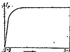
Фиг. 169. Кривая изменения силы тока ротора I_2 в зависимости s при включенной большой самоиндукции L .
