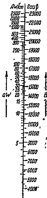
Фиг. 336. Но- мограмма ам- первитков для листово- го железа.
