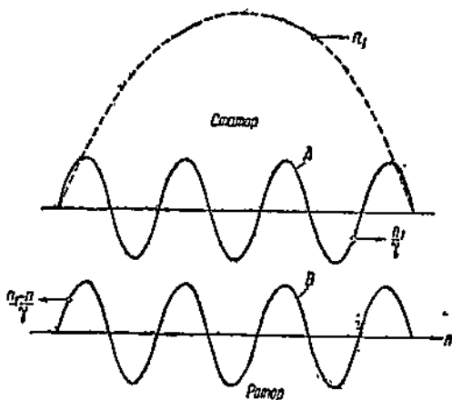
Фиг. 102. Чертеж, поясняющий возникновение синхронных моментов от зубцовых гармоник.
