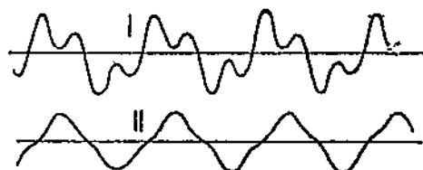
Фиг. 130. I — кривая тока в верхнем волокне провода; II — кривая суммарного тока, текущего по всему сечению провода.
