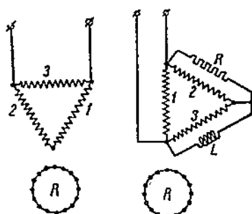
Фиг. 242. Однофазный двигатель Штейнметца.
