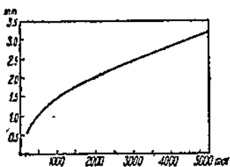
Фиг. 331. Зависимость величины воздушного зазора от диаметра ротора.
