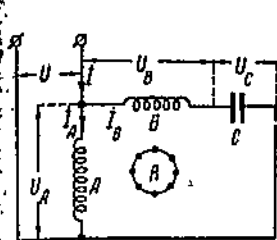
Фиг. 249. Однофазный „конденсаторный“ двигатель.
