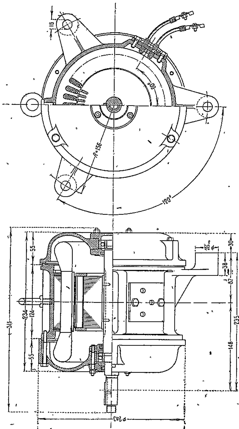
Фиг. 379. Асинхронный двигатель завода им. Дзержинского.
