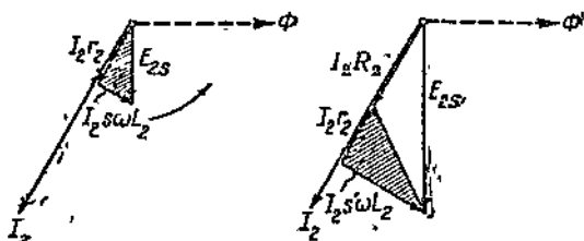
Фиг. 258. Диаграмма при разном скольжении ротора.
