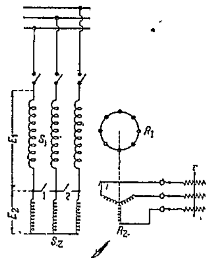
Фиг. 196. Пуск в ход с „разгонным“ вспомогательным двигателем.
