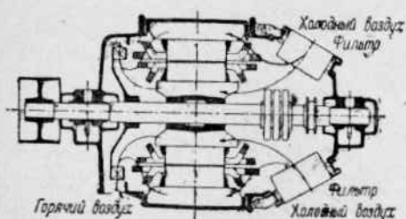
Фиг. 350. Двигатель с воздушными фильтрами.
