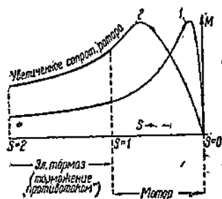
Фиг. 161. Кривые крутящих моментов (1 — для короткозамкнутого ротора; 2 — для ротора со включенным сопротивлением).
