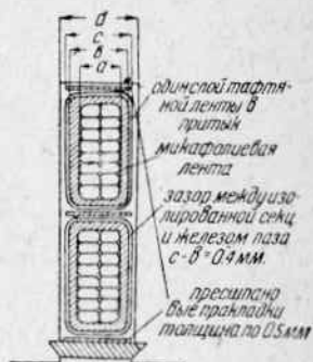
Фиг. 46. Открытый паз статора.
