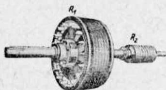
Фиг. 265. Каскадный агрегат для прокатного стана (завод Эрликон в Швейцарии). I — главный асинхронный двигатель на 1 600 л. с.; II — вспомогательный двигатель на 257 л. с.; R_1 — ротор главного двигателя; R_2 — ротор вспомогательного двигателя.
