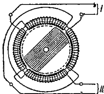
Фиг. 2. Схема двигателя Тесла.
