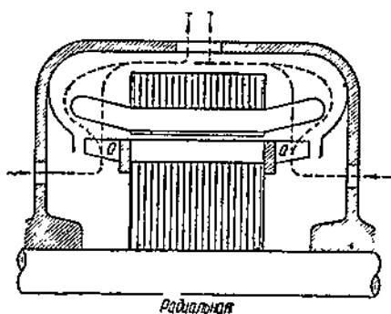
Фиг. 369. Радиальная система вентиляции.
