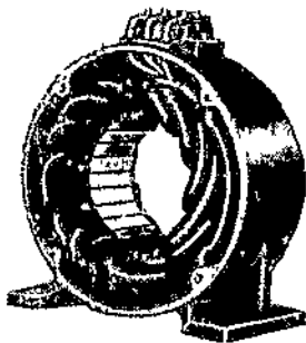
Фиг. 31. Статор асинхронного двигателя с симметричной катушечной обмоткой ( m=3 , q=1 , 2p=8 , K=3 \cdot 4=12 ).
