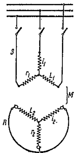
Фиг. 309. Включение статора двигателя на зажимы сети при замкнутом роторе.
