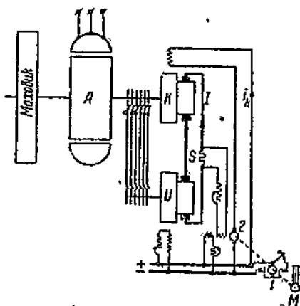
Фиг. 273. Каскад с вольтодобавочной машиной.
