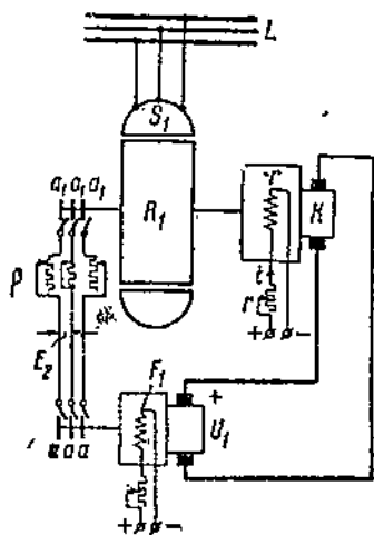
Фиг. 270. „Каскад“ с конвертером и машиной постоянного тока.
