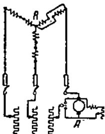
Фиг. 298. Схемы включения возбуждителя A в цепь ротора.
