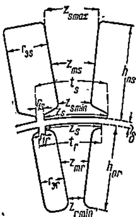
Фиг. 332. Зубцы статора и ротора.
