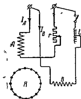
Фиг. 239. Однофазный двигатель (А — рабочая обмотка; В — вспомогательная обмотка).
