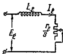
Фиг. 82. Эквивалентная схема ротора.
