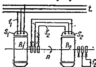
Фиг. 263. Каскадное соединение (автора).
