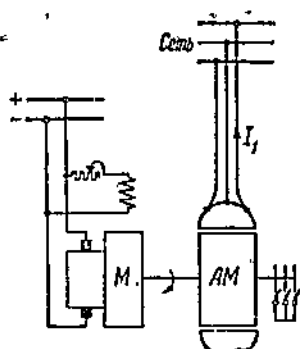
Фиг. 155. Работа асинхронной машины в качестве генератора.
