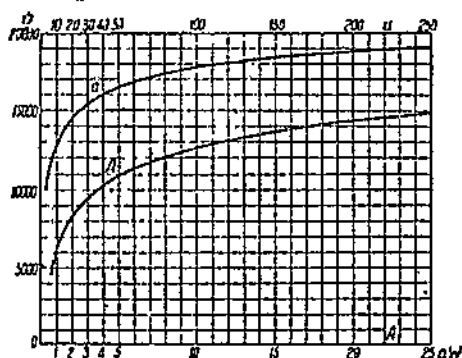
Фиг. 335. Кривые намагничивания.
