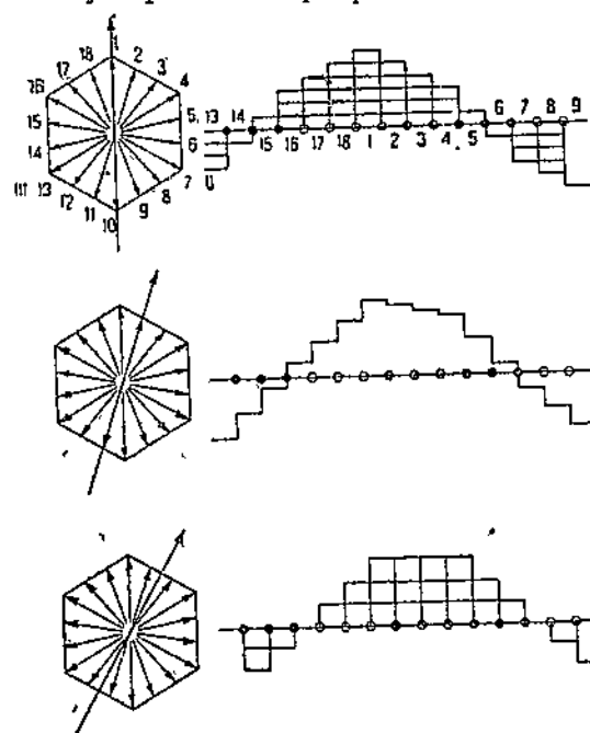
Фиг. 68. Построение кривой м. д. с. для трехфазной обмотки ( q = 3 ).
