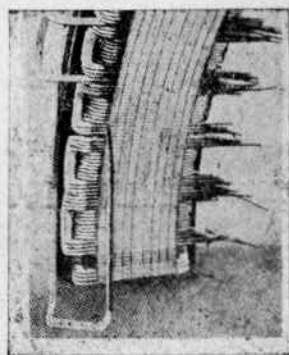
Фиг. 42. Шаблонная обмотка, заложённая в полузакрытые пазы. Свободные концы катушек еще не спаяны.
