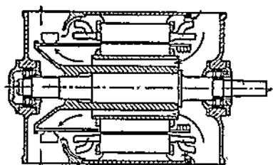
Фиг. 374. Ротор с увеличенным активным сопротивлением.
