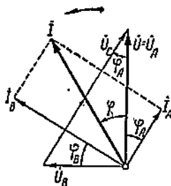
Фиг. 249. Однофазный „конденсаторный“ двигатель.
