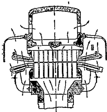
Фиг. 371. Пути движения воздушной струи при радиальной вентиляции.
