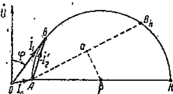
Фиг. 148. Круговая диаграмма для схемы замещения фиг. 145 при замкнутом рубильнике А.
