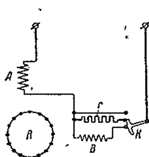
Фиг. 240. Однофазный двигатель.
