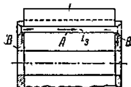
Фиг. 114. Схема расположения болтов, стягивающих тело ротора.
