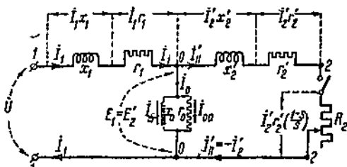
Фиг. 144. Эквивалентная схема для векторной диаграммы фиг. 143 (левый чертеж).
