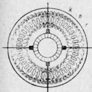
Фиг. 288. Схема двухфазного компенсатора Шербиуса.
