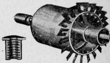
Фиг. 95. Ротор с косо расположенными пазами.
