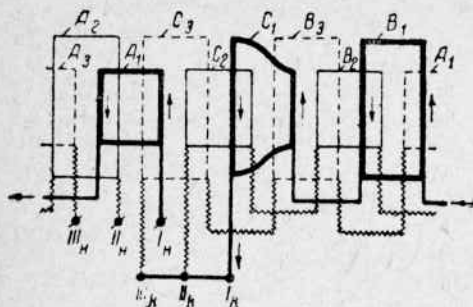
Фиг. 21. Схема трехфазной катушечной обмотки при нечетном p ( m=3 , q=1 , 2p=6 , K=3 \cdot 3=9 ) с одной несимметричной шпуйей C_1 .
