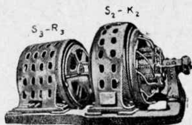
Фиг. 285. Агрегат Шербиуса, состоящий из асинхронного генератора S_3 - R_3 и коллекторной машины S_2 - K_2 (фиг. 283).
