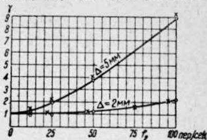
Фиг. 127. Отношение плотности тока в крайнем верхнем волокне к плотности тока в крайнем нижнем волокне при разных частотах.
