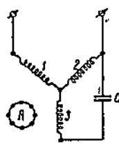
Фиг. 250. Однофазные „конденсаторные“ двигатели.
