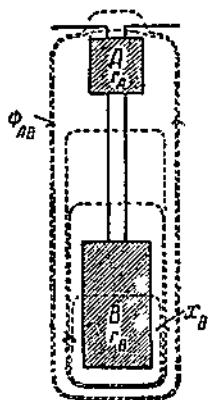
Фиг. 207. Паз ротора Бушера.
