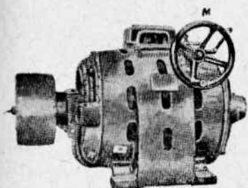
Фиг. 179. Внешний вид двигателя по первой схеме Бушера.
