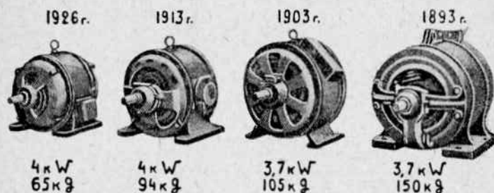
Фиг. 329. Уменьшение веса и размеров асинхронных двигателей.
