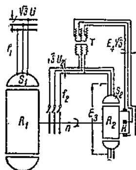
Фиг. 277. Каскад Кремера с шунтовым коллекторным двигателем.
