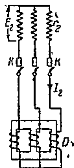
Фиг. 171. Схема включения дроссельной катушки D в цепь ротора асинхронного двигателя.
