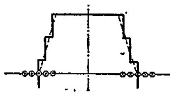
Фиг. 65. Кривая м. д. с. одной фазы q = 5 .
