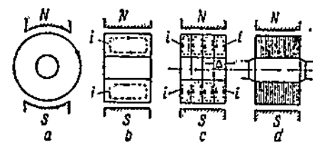
Фиг. 109. Вихревые токи в железе ротора.
