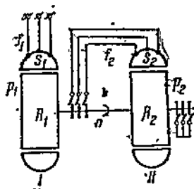
Фиг. 259. Каскадное соединение двух асинхронных двигателей.
