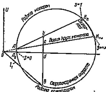
Фиг. 154. Моторный и генераторный режим на диаграмме.
