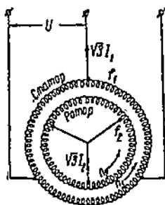
Фиг. 71. Первичная и вторичная цепи асинхронного двигателя (соединение в треугольник).
