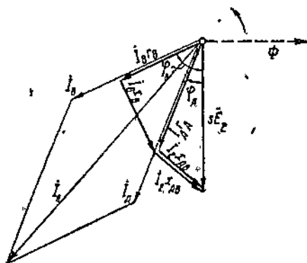
Фиг. 209. Диаграмма токов и напряжений в роторе Бухеро.
