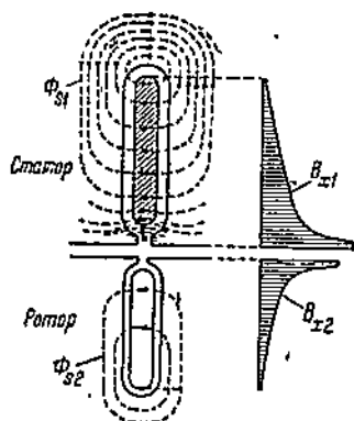
Фиг. 340. Поток рассеяния в пазах статора и ротора.
