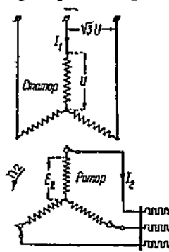
Фиг. 70. Первичная и вторичная цепи двигателя (соединение в звезду).
