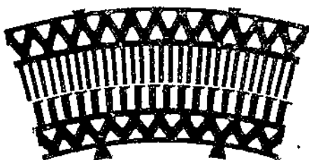
Фиг. 372. Железо статора и ротора мощного двигателя.
