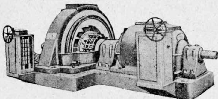
Фиг. 265. Каскадный агрегат для прокатного стана (завод Эрликон в Швейцарии). I — главный асинхронный двигатель на 1 600 л. с.; II — вспомогательный двигатель на 257 л. с.; R_1 — ротор главного двигателя; R_2 — ротор вспомогательного двигателя.
