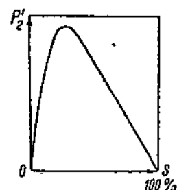
Фиг. 96. Кривая зависимости мощности ротора P'_2 от скольжения s .
