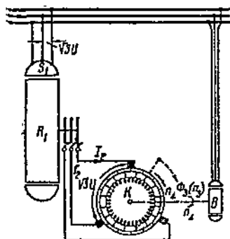
Фиг. 286. Схема соединения асинхронного двигателя S_1 с R_1 с компенсатором сдвига фаз K .
