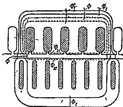
Фиг. 83. Поток асинхронного двигателя.
