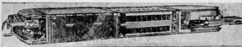
Фиг. 376. Двигатель врубовой машины на 22,5 kW Харьковского электромеханического завода.
