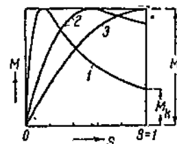
Фиг. 91. Кривые зависимости крутящего момента M от скольжения s при различных соотношениях x_1 и r_2 .
