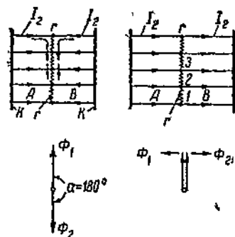
Фиг. 178. Взаимное расположение потоков \Phi_1 и \Phi_2 и статоров двигателя Бушера; распределение токов в его роторе при пуске в ход (левый чертеж) и нормальной работе (правый чертеж).
