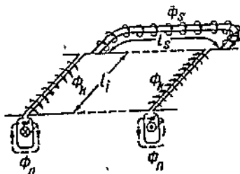
Фиг. 341. Поток рассеяния в отдельных частях обмотки.
