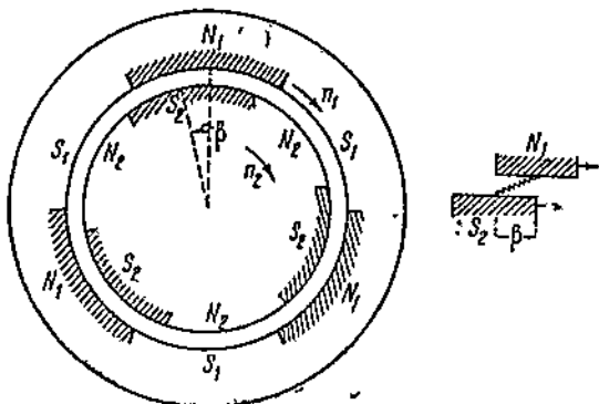
Фиг. 93. Чертеж, поясняющий возникновение „гистерезисного“ момента.
