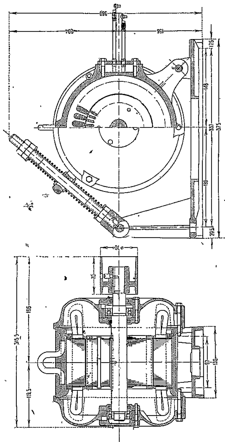
Фиг. 378. Двигатель Московского завода имени Лепсе мощностью в 0,4 к.в.
