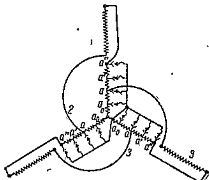
Фиг. 205. Рабочее соединение обмотки ротора.
