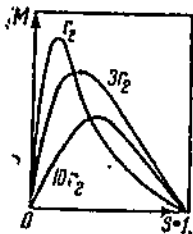
Фиг. 228. Кривые моментов вращения.
