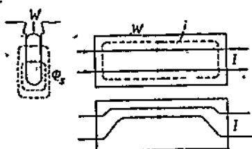
Фиг. 118. Влияние потока рассеяния на токораспределение в проводнике.
