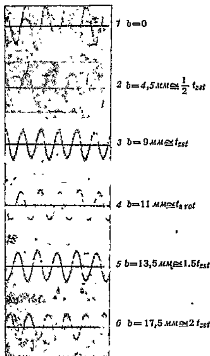
Фиг. 106. Влияние скоса пазов ротора на высшие гармоники. Мотор ТА 12/4 завода им. Лепсе. Холостой ход при 220V. Измерительный проводничок расположен в верхней части паза статора. b — скос паза в мм.
