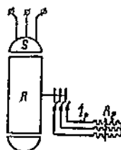
Фиг. 163. Включение пускового реостата ( R_2 ) в цепь ротора асинхронного двигателя.
