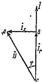
Фиг. 141. Векторная диаграмма для схемы фиг. 140.
