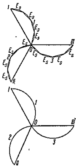
Фиг. 39. Векторная диаграмма напряжений для разрезной обмотки согласно фиг. 38.
