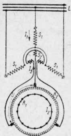
Фиг. 292. Компенсированный двигатель Гейланда.
