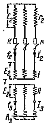
Фиг. 170. Схема включения реостата R_3 в цепь ротора через посредство трансформатора T .
