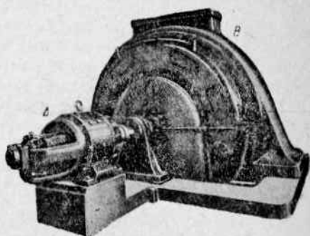
Фиг. 295. Синхронно-индукционный двигатель. А — возбудитель; В — двигатель.
