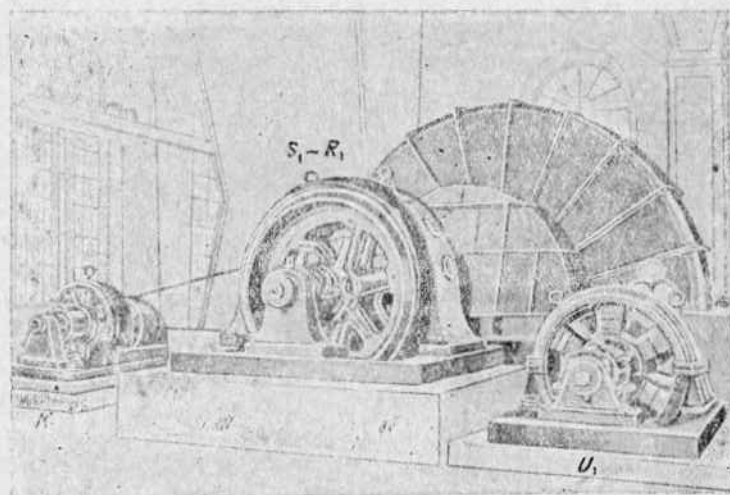
Фиг. 271. Каскадное соединение асинхронного двигателя с конвертером (фиг. 270). Мощность асинхронного двигателя 890 kW. Двигатель приводит во вращение шахтный вентилятор. S_1—R_1 — главный двигатель; K — двигатель постоянного тока; U_1 — одноякорный преобразователь. Регулирование происходит в пределах 285—170 об/мин.
