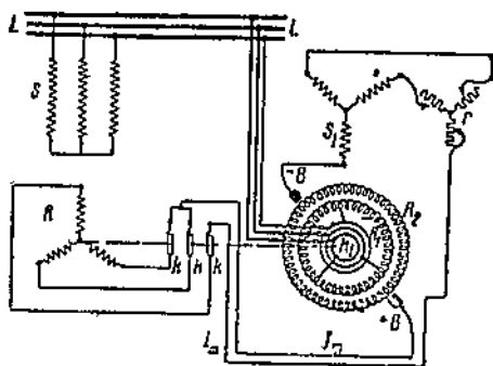
Фиг. 303. Синхронно-индукционный двигатель S-R с преобразователем-возбудителем S_1-R_2 (схема автора).
