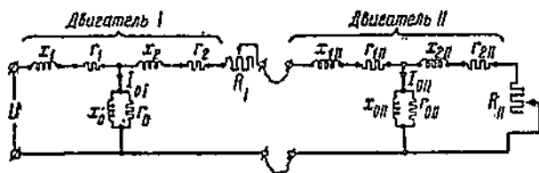
Фиг. 261. Схема замещения для „каскада“.
