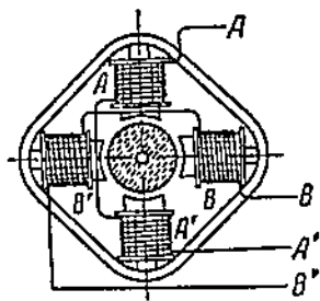
Фиг. 1. Схема двигателя Феррариса с массивным железным ротором в виде цилиндра без обмотки.
