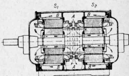
Фиг. 180. Разрез двигателя Брунка.
