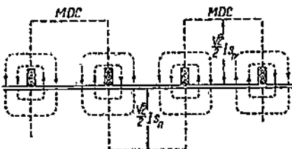
Фиг. 62. Распределение кривой м. д. с. для однофазной обмотки при q = 1 .
