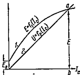
Фиг. 160. Характеристика самовозбуждающегося асинхронного генератора.
