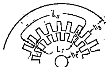
Фиг. 334. Магнитная цепь асинхронного двигателя.
