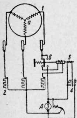
Фиг. 300. Схема с автоматическим включением возбудителя.
