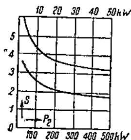
Фиг. 320. Средние значения скольжения в функции мощности.
