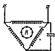
Фиг. 250. Однофазные „конденсаторные“ двигатели.
