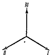
Фиг. 29. Векторная диаграмма напряжения, соответствующая фиг. 27, при правильном соединении катушек.
