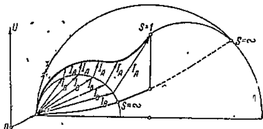
Фиг. 210. Диаграмма токов в роторе Бушера.
