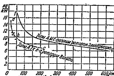
Фиг. 321. „Удельный вес“ (в кг на один kW) в функции мощности машины.
