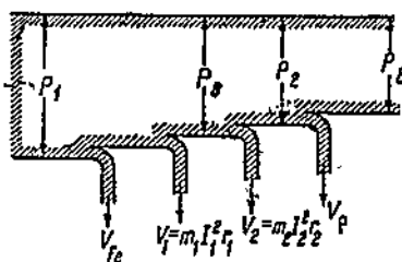
Фиг. 88. Энергетическая диаграмма асинхронного двигателя. Мощность P_s является, как будет видно ниже, весьма характерной величиной в теории асинхронных двигателей.
