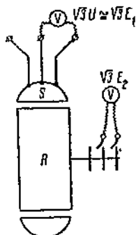
Фиг. 74. Схема асинхронного двигателя, включенного к сети с разомкнутой вторичной цепью.
