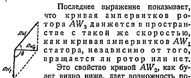
Фиг. 81. Пространственная диаграмма ампервитков статора и ротора.
