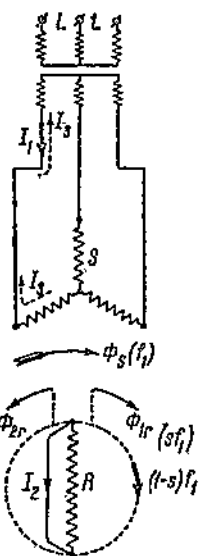
Фиг. 262. Двигатель с однофазным ротором.
