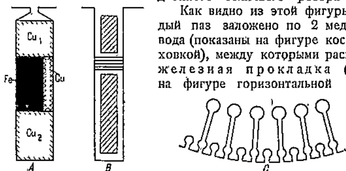
Фиг. 189. А — ротор GEC; В — ротор SSW; С — ротор с двойным числом проводов пусковой обмотки. Cu_1 — пусковая обмотка; Cu_2 — рабочая обмотка; Fe — железный стержень; Cu — медный стержень.
