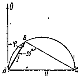
Фиг. 142. Векторная диаграмма фиг. 141, повернутая на угол 90^\circ .
