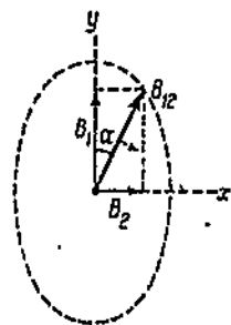
Фиг. 11. Эллиптическое вращающееся магнитное поле.
