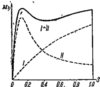
Фиг. 185. Кривые крутящего момента двигателя Бушерио согласно схеме фиг. 169.
