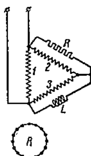
Фиг. 243. Двигатель Штейнметца.
