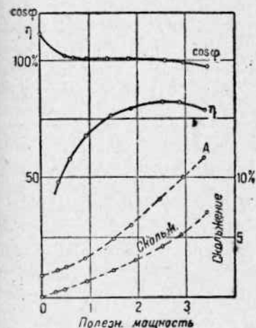
Фиг. 294. Рабочие кривые компенсированного двигателя.
