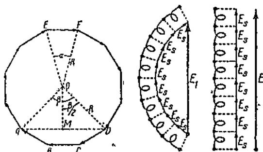
Фиг. 57—58. Сложение э. д. с. для случая совпадающих осей витков (правый чертеж) и случая витков, расположенных по окружности статора (левый чертеж).
