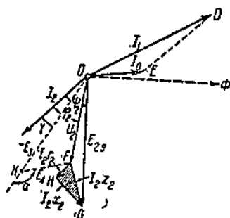
Фиг. 276. Векторная диаграмма для схемы Кремера (фиг. 275).
