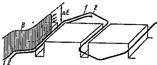
Фиг. 313. Блуждающая волна с „крутым фронтом“.
