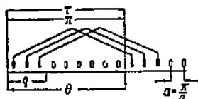
Фиг. 60. Определение обмоточного коэффициента для однофазной обмотки при q=3 .
