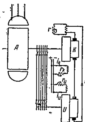
Фиг. 272. „Каскад“ с шестифазным конвертором.
