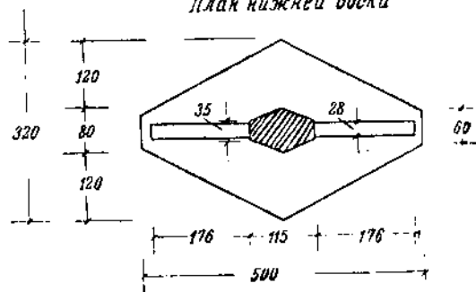
Плак нижней доски
