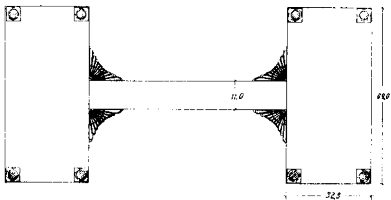
План нижней доски
