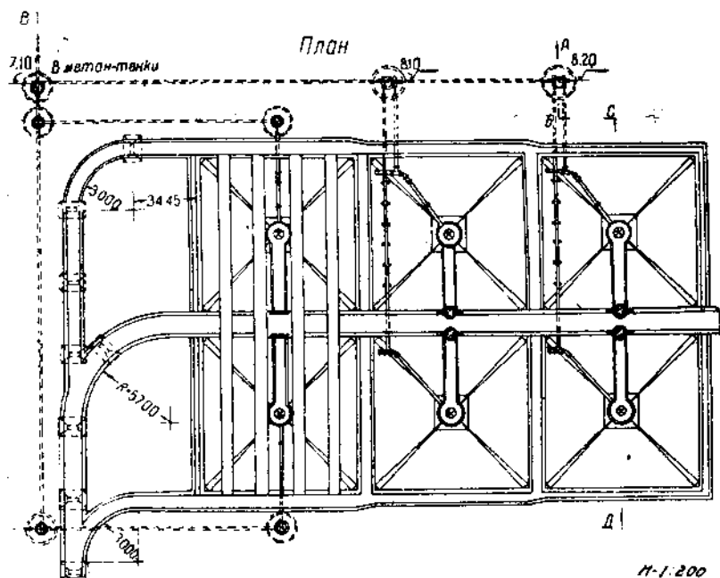
Рис. 16. План первичных отстойников Кожуховской станции аэрации.
