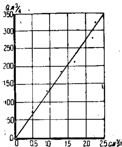
Рис. 18. Влияние нагрузки на вынос взвешенных веществ из отстойника.
