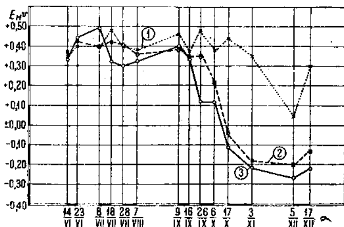
Рис. 57. E_h воды из осушительных канав Люблинских полей фильтрации: Водоотводная—1, Осушительная—2, Тальвег—3.
