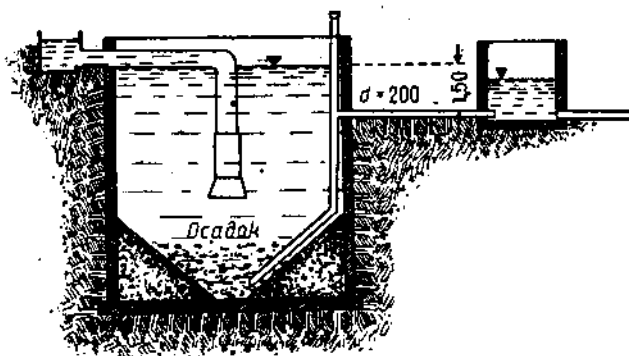
Рис. 27. Схема удаления осадка из вертикального отстойника.
