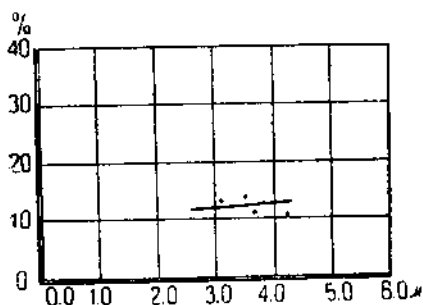
Рис. 22. Процент выноса взвешенных веществ из отстойника при различной длине опускаемой трубы.
