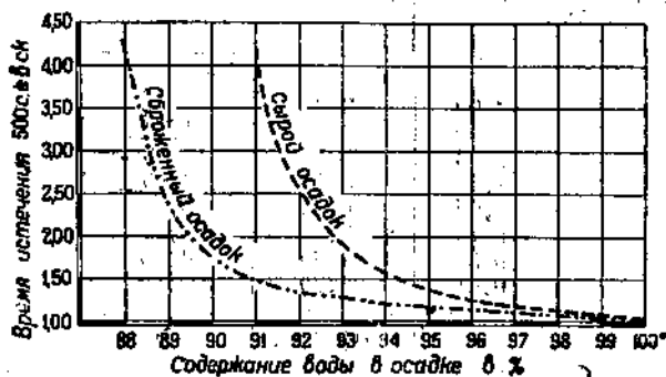
Рис. 30. Относительная вязкость сырого и сброженного осадков.
