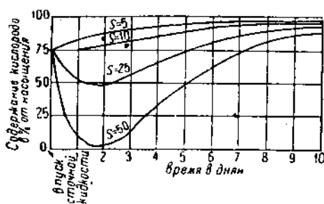
Рис. 61. Изменение величины реэрации в водоеме ниже спуска сточных вод по Маггу.
