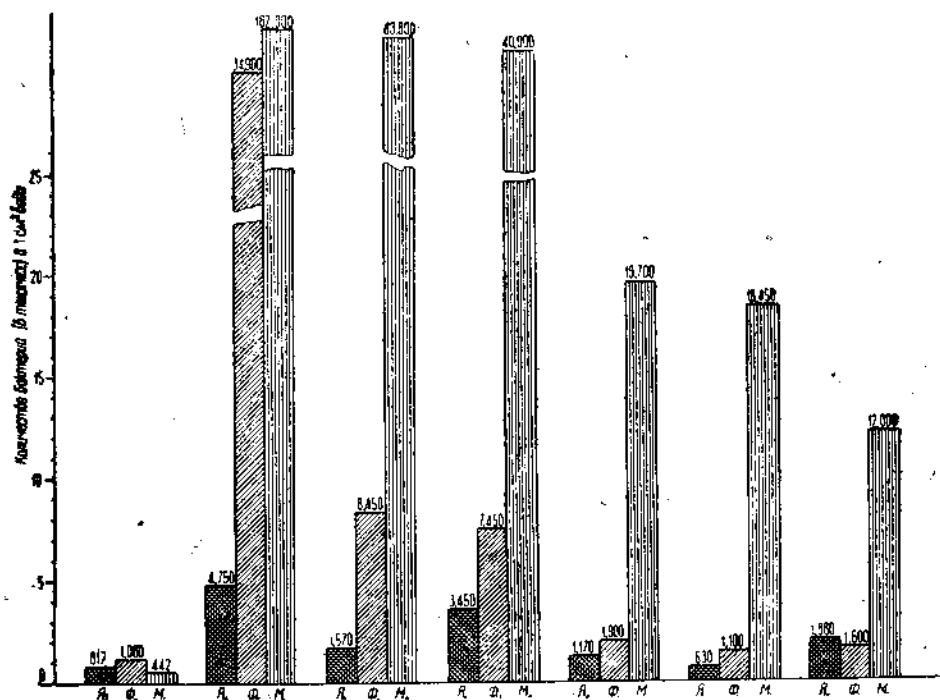
Рис. 69. Скорость отмирания бактерий в воде р. Пехорки зимой (счет на мясо-пептонном агаре при 37°С).
