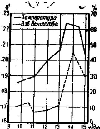
Рис. 20. Влияние колебаний температуры на вынос взвешенных веществ из отстойника. Наблюдение 4/VII 1931 г.
