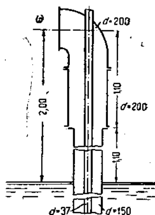
Рис. 47. «Конструкция № 11».
