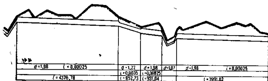
Рис. 6. Продольный профиль самотечной части Люберецкого канала.
