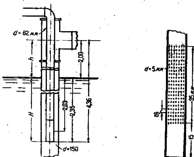
Рис. 41. Эрлифт Кожуховской станции (Москва) № 1—3.
