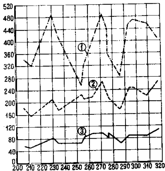
Рис. 50. Сравнительное определение в сточной жидкости: 1—БПК с K=0,1 2—окисляемости по Абботу, 3—окисляемости по Кубелю с БПК с собственной константой, нанесенной на абсциссу.
