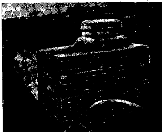
Рис. 1. Наружный вид трещин кирпичной кладки смотрового колодца на обмороженном Люберецком водоводе.
