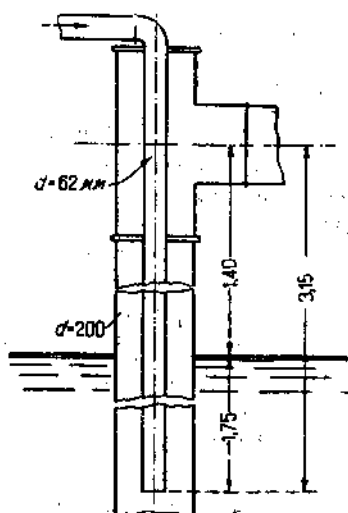
Рис. 43. Эрлифт Кожуховской станции № 5.
