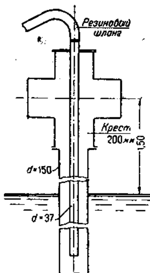
Рис. 45. «Конструкция № 7».
