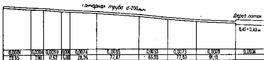
Рис. 26. Закрытый гончарный илопровод на сушильные площадки.
