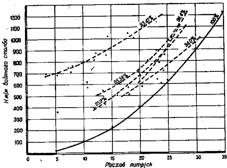
Рис. 40. Зависимость сопротивлений от расхода осадка по закрытому трубопроводу.
