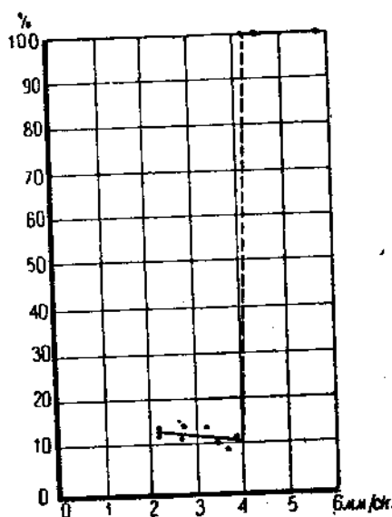
Рис. 25. Процент выноса взвешенных веществ из отстойника при различной величине средней скорости движения жидкости в сечении отстойника на уровне щита.
