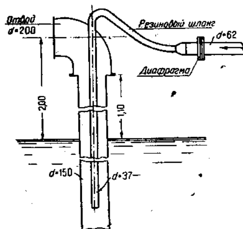
Рис. 46. «Конструкция № 8».
