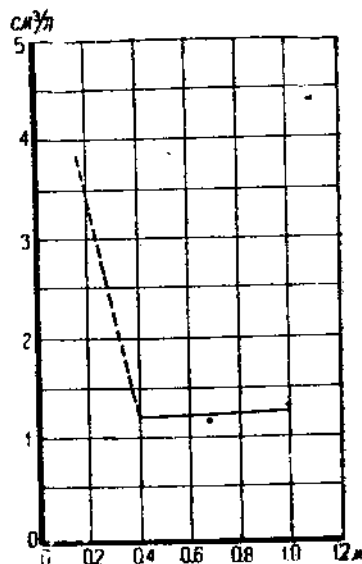
Рис. 23. Вынос взвешенных веществ из отстойника при различной ширине щели между щитом и концом трубы.
