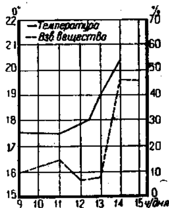
Рис. 19. Влияние колебаний температуры на вынос взвешенных веществ из отстойника. Наблюдение 2/VII 1931 г.
