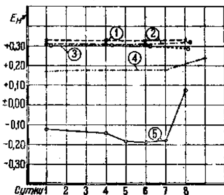
Рис. 55. Люблинская опытная станция определила E_h : 1, 2, 4 — воды, очищ. на аэрофильтрах; 3 — воды из перколятора № 20; 5 — сточная жидкость.
