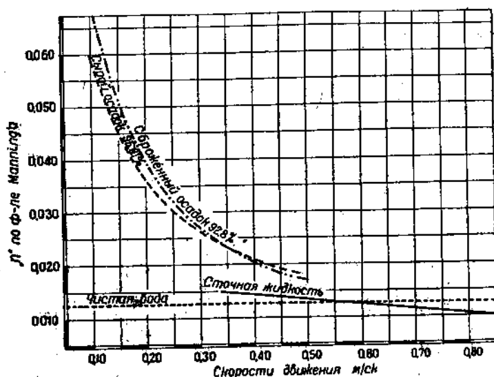
Рис. 36. Влияние скоростей течения на изменение коэффициента шероховатости для осадков при движении по лоткам.
