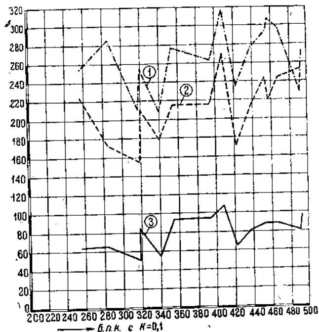
Рис. 49. Сравнительное определение в сточной жидкости: 1—БПК с собственной K , 2—окисляемости по Абботу и 3—окисляемости по Кубелю с БПК с K=0,1 , нанесенной на абсциссу.
