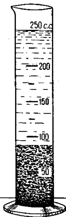
Рис. 28. Объемное определение влажности осадка (вид осадка через 15 мин.).
