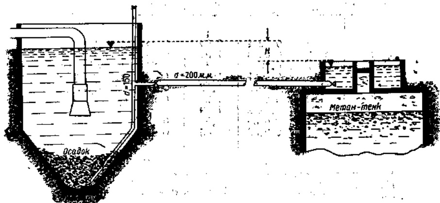
Рис. 38. Схема передачи осадка из вертикального отстойника в метан-танк по чугунной и гончарной трубе.
