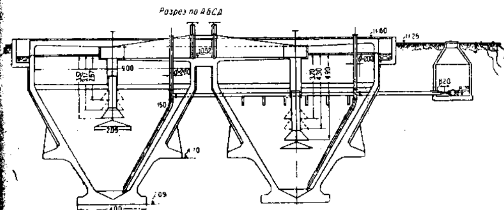
Рис. 17. Разрез первичных отстойников Кожуховской станции аэрации.
