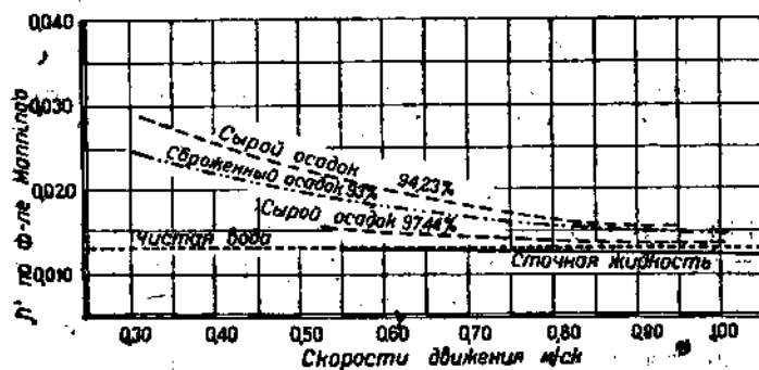
Рис. 37. Влияние скоростей течения на изменение коэффициента шероховатости для осадков при движении по лоткам.
