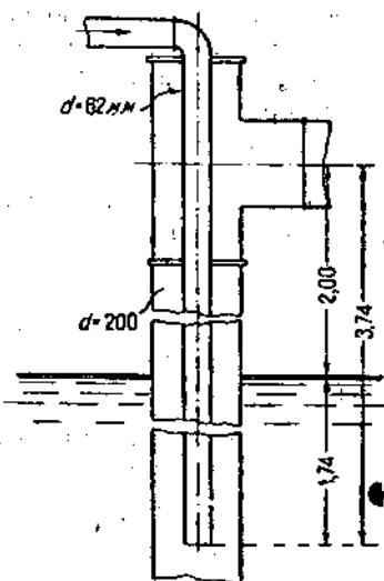
Рис. 42. Эрлифт Кожуховской станции № 4.
