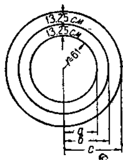
Рис. 11. Схема расчета напряжений от удлинения внутреннего полукольца.
