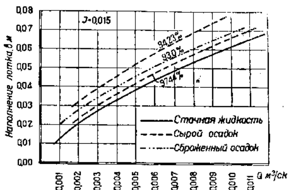
Рис. 31. Непосредственные измерения расходов осадков и сточной жидкости по лотку с уклоном 0,015.
