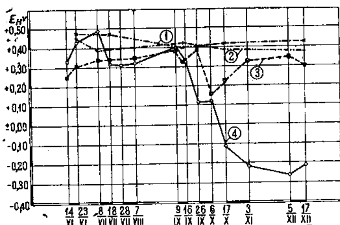
Рис. 56. E_h воды из осушительных канав Люблинских полей фильтрации. Канавы № 43—1; канавы № 41—2; канавы № 30—3 и Тальвег—4.
