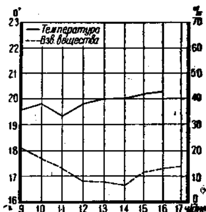
Рис. 21. Влияние колебаний температуры на вынос взвешенных веществ из отстойника. Наблюдение 9/VII 1931 г.
