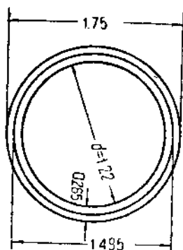
Рис. 7. Поперечные размеры элементов канала d=1,22 м.
