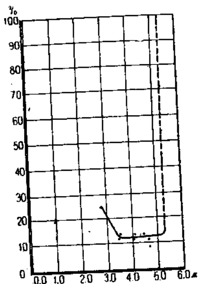
Рис. 24. Процент выноса взвешенных веществ из отстойника при различной глубине погружения щита.
