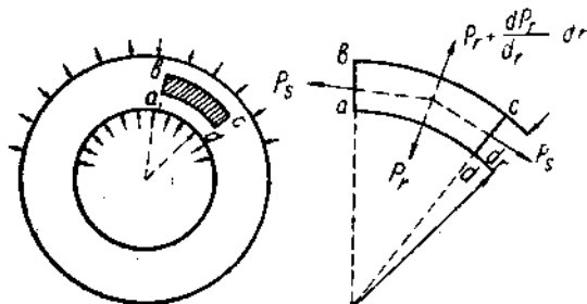
Рис. 12. Схема расчетного элемента канала.
