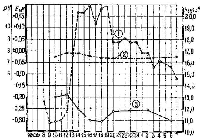
Рис. 54. Часовые пробы сточной жидкости из разводящих канав;
