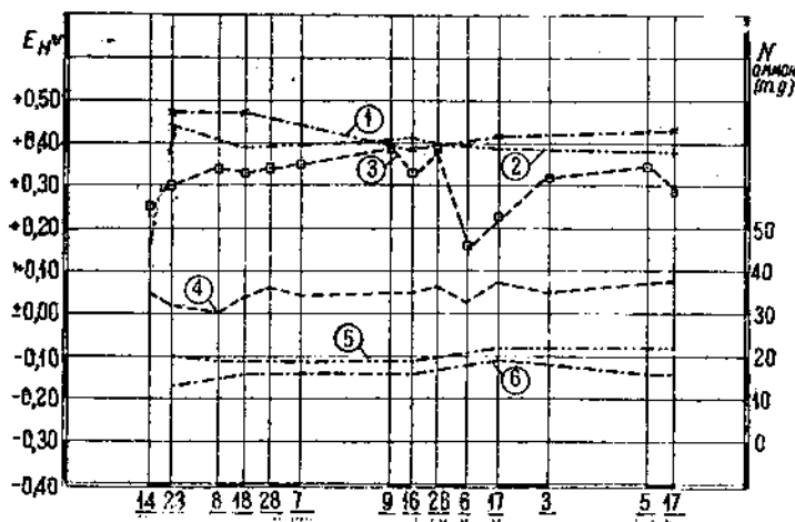
Рис. 58. Канавка № 43: E_h —1, азот аммонийный 6. " № 41: E_h —2, " " 5. " № 30: E_h —3, " " 4.
