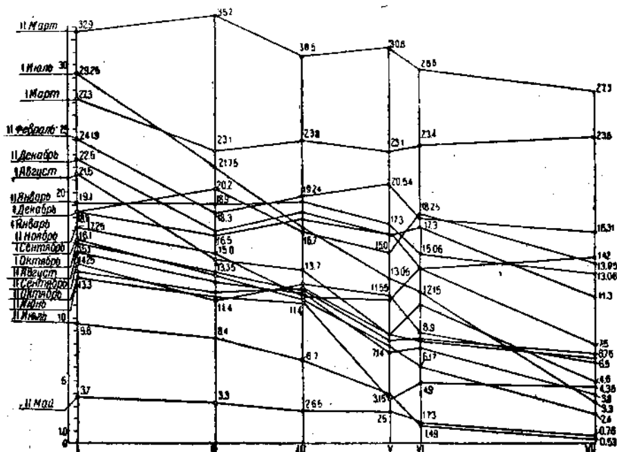
Рис. 67. Содержание азота аммонийного в воде р. Пехорки.
