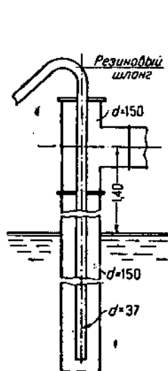
Рис. 44. Эрлифт «Конструкция № 6».
