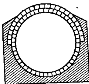
Рис. 4. Поперечный вид канала со стулом.
