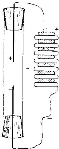
Схема опыта Никольсона и Карлейля в 1800 г.: разложение воды током. Electroдами служили медные проволоки.
