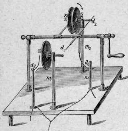
Машина Никольсона (1788 г.) — „удвоитель“, позволяющий, используя электричество через влияние, усиливать заряд на круге и, таким образом, узнавать знак очень слабого заряда. (Рисунок из „Gesch. der Electricität“ — Albrecht'a.)
