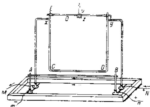
Станок, изготовленный по заказу Ампера в 1820 г. для демонстрации взаимодействия прямых токов. (Из мемуара Ампера 1820 г.)
