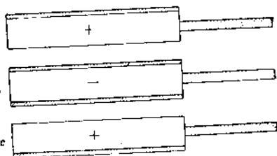
Схема, объясняющая работу „дубликатора“ Беннета (1787 г.). Круг a покрыт лаком сверху; круг b покрыт лаком, как изолятором, с обеих сторон; круг c — покрыт лаком снизу.
