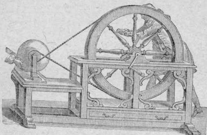
Электрическая машина трения 1747 г. Стекланный шар электризуется трением о ладони рук (из первого сочинения по электричеству, написанного Нолле в 1747 г.).
