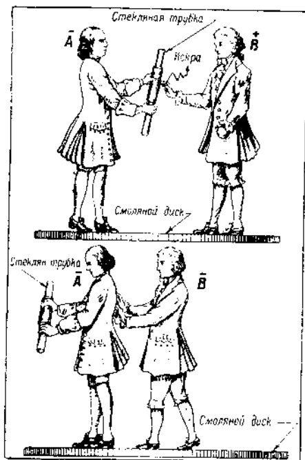
Опыт Франклина, приведший его к „уни- тарной теории“ электричества. Экспери- ментирующие стоят на смоляном диске. При первом опыте они заряжаются противо- положным электричеством, при втором (внизу)—одноименно.
