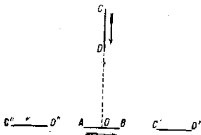
Взаимодействие двух перпендикулярных между собой элементов токов.
