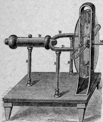
Электрическая машина со стеклянным диском Рамздена 1768 г.
