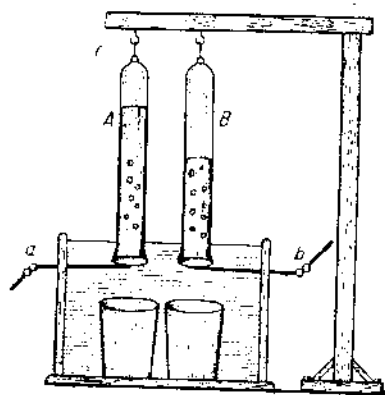
Один из первых приборов для разложения воды, где в стеклянных робирках собирались водород и кислород (построен Риттером в 1801 г.).
