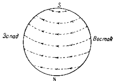
Схема, объясняющая исходную гипотезу всей теории Ампера о существовании „земного тока“ с востока на запад.
