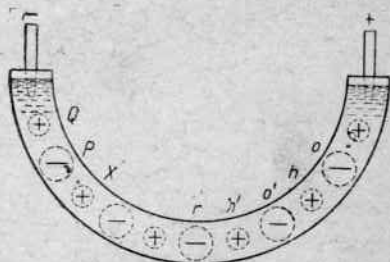
Теория электролиза Гротгуса в 1805 г. (Схема из мемуара Гротгуса 1806 г.)
