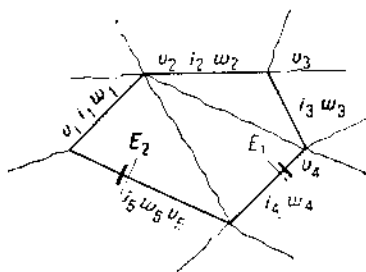
Схема для пояснения 2-го правила Кирхгофа.
