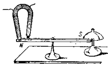
Схема, объясняющая устройство первого электрического звонка Генри в 1831 г.
