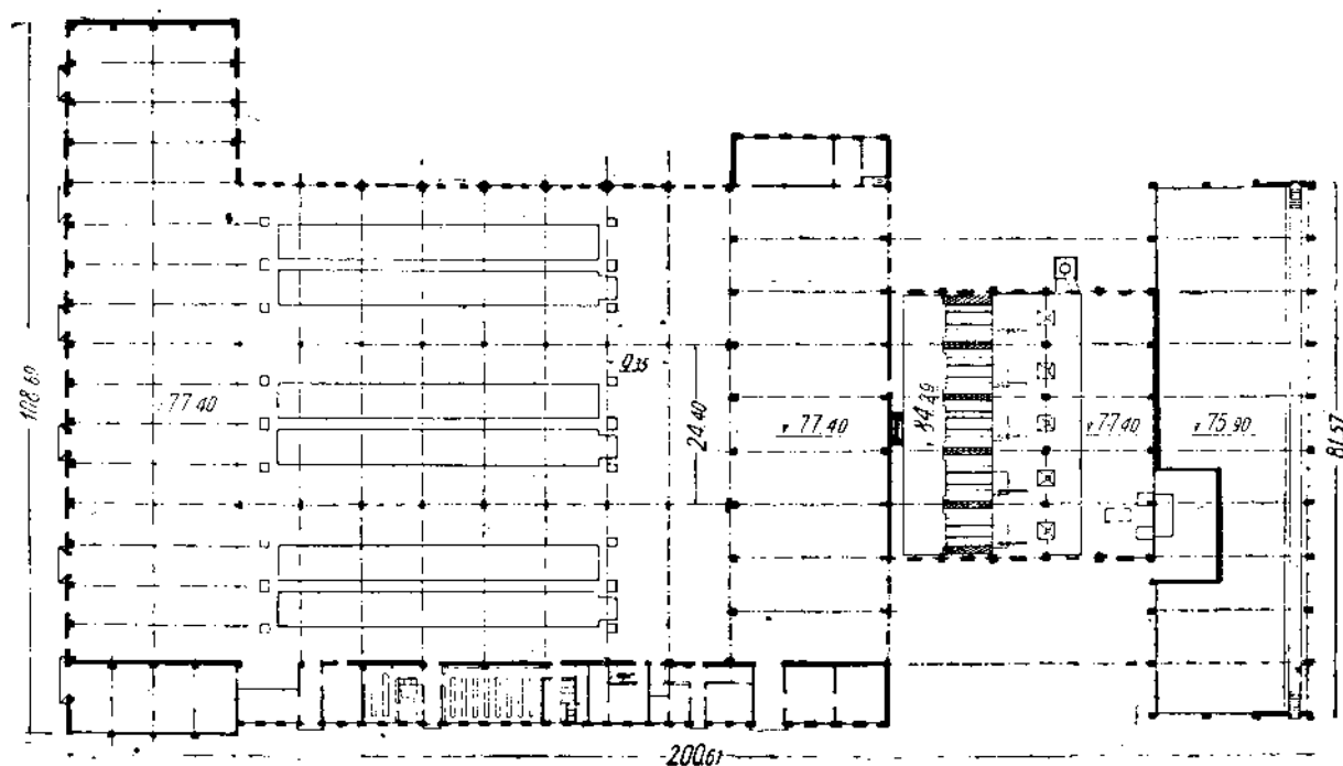
ГУНДОБИН Н. П., АРХ.-ХУД., ГР. ИНЖ., ОМИНИН Е. Н., СОЛОВЬЕВА В. В., КОНДРАТЬЕВ И. Д., АРХ.-ХУД., ЗАРХИ Л. И., ИНЖ. ПУТЕЙ СООБЩЕНИЯ. ДНЕПРОВСКИЙ АЛЮМИНИЕВЫЙ КОМБИНАТ. ЭЛЕКТРОДНЫЙ ЗАВОД. ПОСТРОЕНО В 1933 г.
