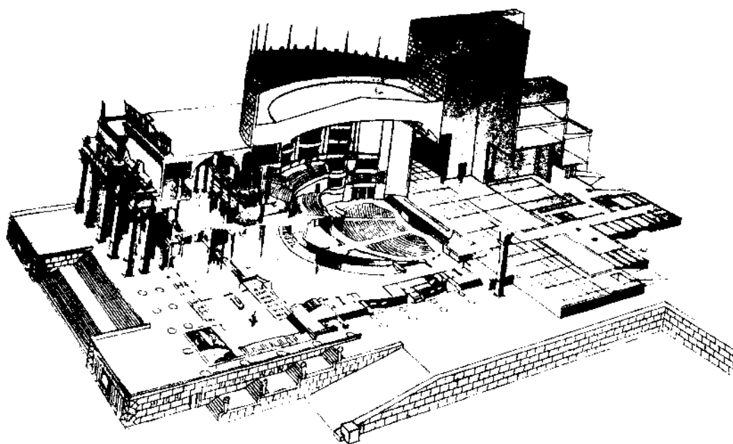
АКСОНОМЕТРИЯ РАЗРЕЗА
