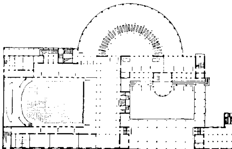
ГЕГЕЛЛО А. И., АРХ.-ХУД., ГР. ИНЖ., КРИЧЕВСКИЙ Д. Л., ГР. ИНЖ. ПРОЕКТ КИНО-ТЕАТРА В МОСКОВСКОМ РАЙОНЕ В ЛЕНИНГРАДЕ. ПЕРСПЕКТИВЫ И ПЛАН I ЭТАЖА.
