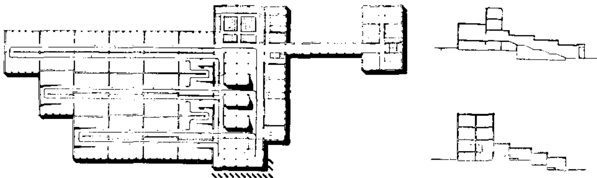
СРЕДНЕ-АЗИАТСКИЙ МУЗЕЙ РЕВОЛЮЦИИ в г. ТАШКЕНТЕ 1928 г. БАРУТЧЕВ А. К., ГИЛЬТЕР И. А. АРХИТ.-ХУДОЖНИКИ. ЛЕНИНГРАД
