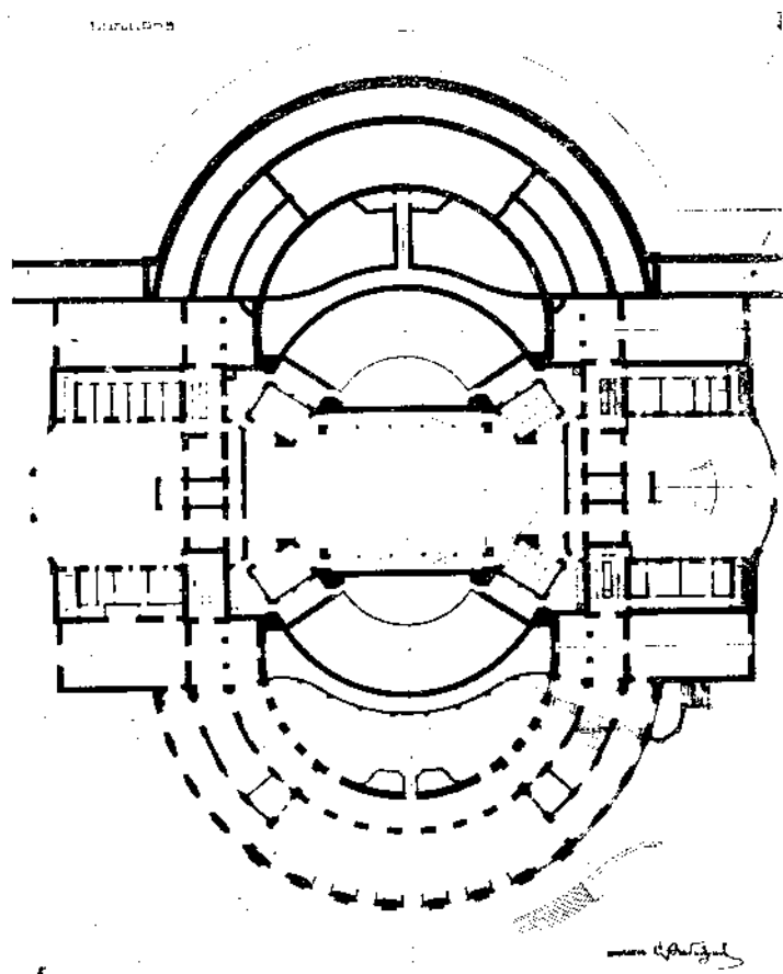
ТАМАНЬЯН А. И. АКАД. АРХИТ. НАРОДНЫЙ АРХИТ. СССР АРМЕНИИ. НАРОДНЫЙ ДОМ В ЕРИВАНИ. ФАСАД ЗИМНЕГО ТЕАТРА. ПЛАН 1-го и 2-го ЭТАЖЕЙ. ПОСТРОЙКА НАЧАТА В 1931 г.
