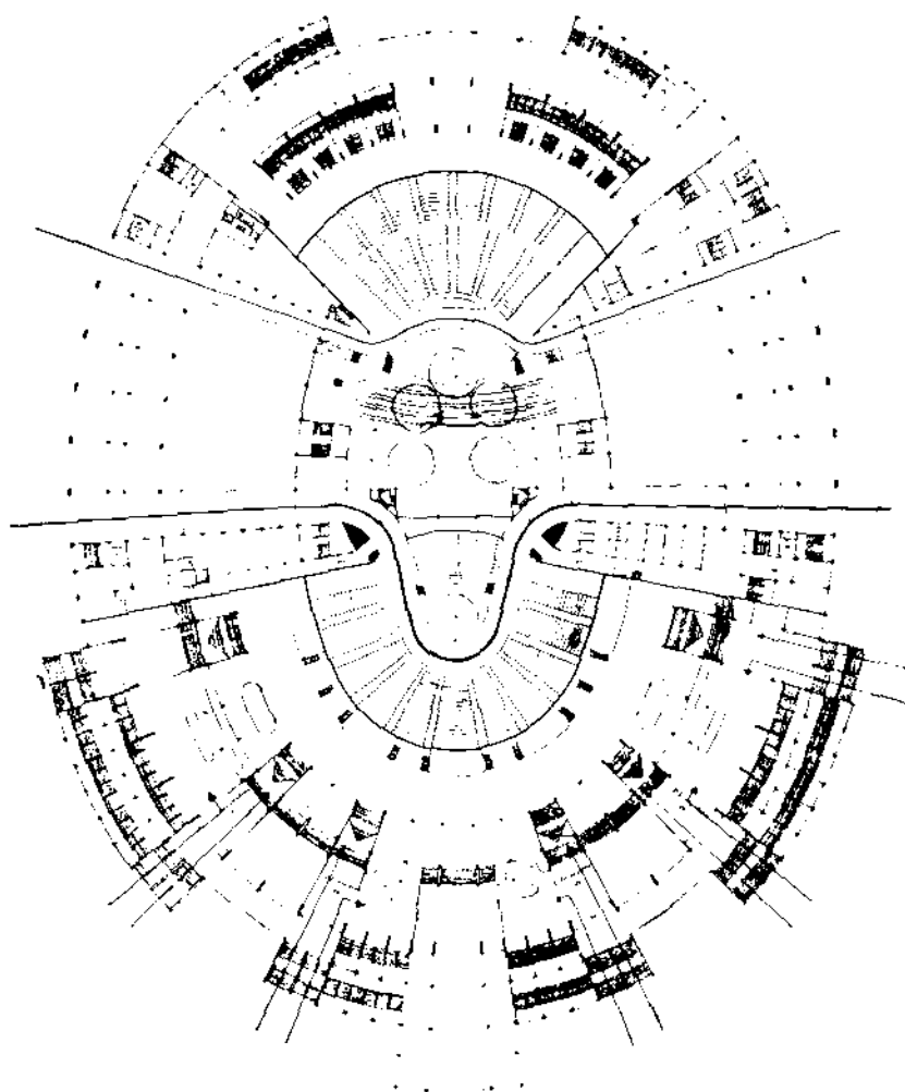
КОНКУРСНЫЙ ПРОЕКТ ДВОРЦА СОВЕТОВ. ПРИОБРЕТЕН СТРОИТЕЛЬСТВОМ. ПЛАН 1 ЭТ. И РАЗРЕЗ ПО ПРОДОЛЬНОЙ ОСИ.
