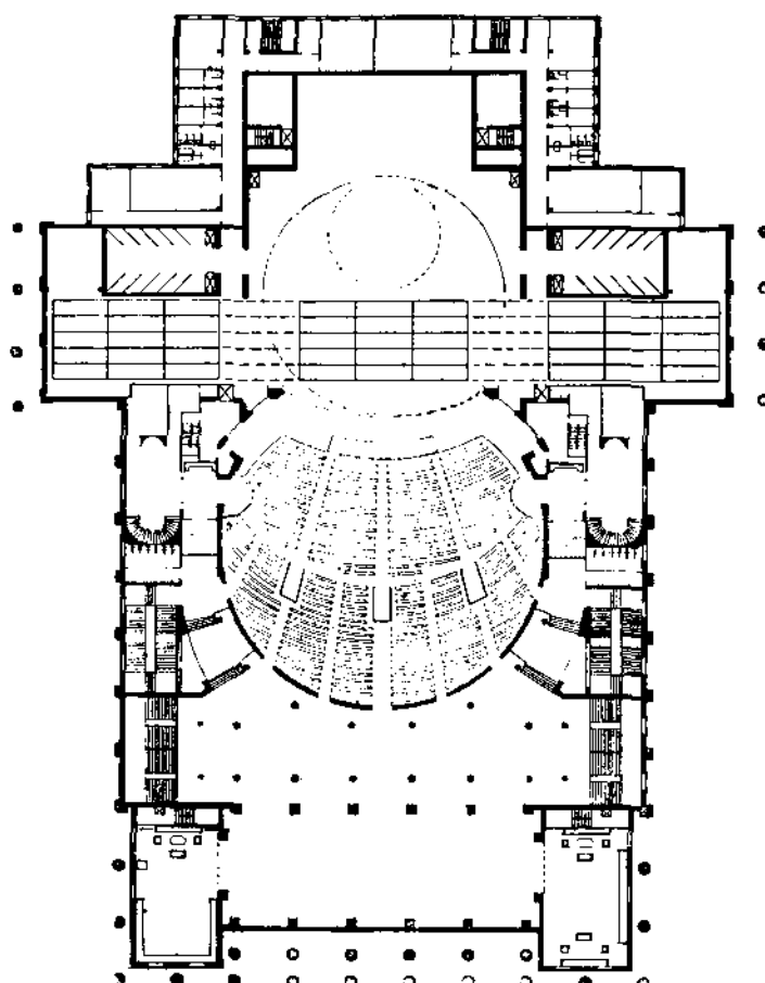
ТЕАТР КРАСНОЙ АРМИИ В МОСКВЕ. ВТОРОЙ ВАРИАНТ.
