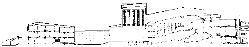
РАЗРЕЗ ПО КЛУБНОЙ ЧАСТИ.
