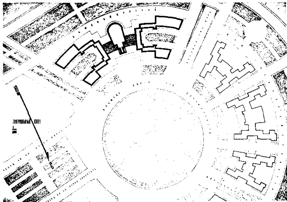
СЕРАФИМОВ С. С., ЗАНДБЕРГ-СЕРАФИМОВА М. А., АРХ.-ХУД. ЛЕНИНГРАД. ДОМ ПРОЕКТОВ ХАРЬКОВ. ПОСТР. В 1930-1934 г.
