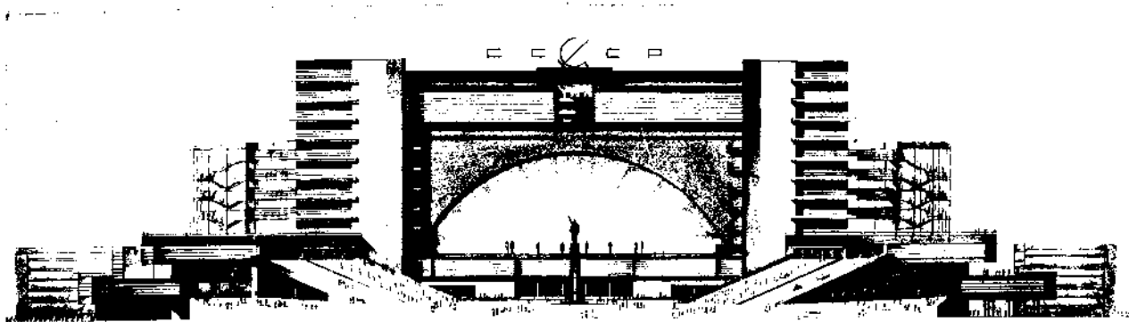
ГЛАВНЫЙ ФАСАД.
