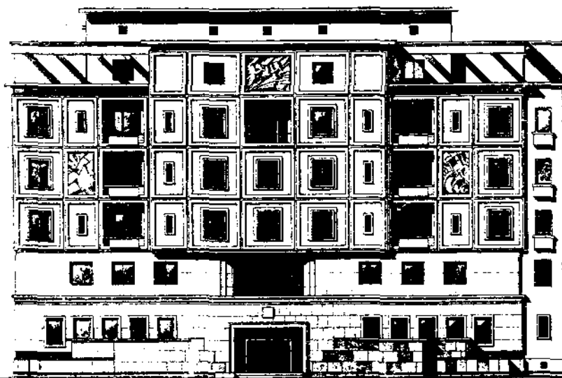
Ф А С А Д.
