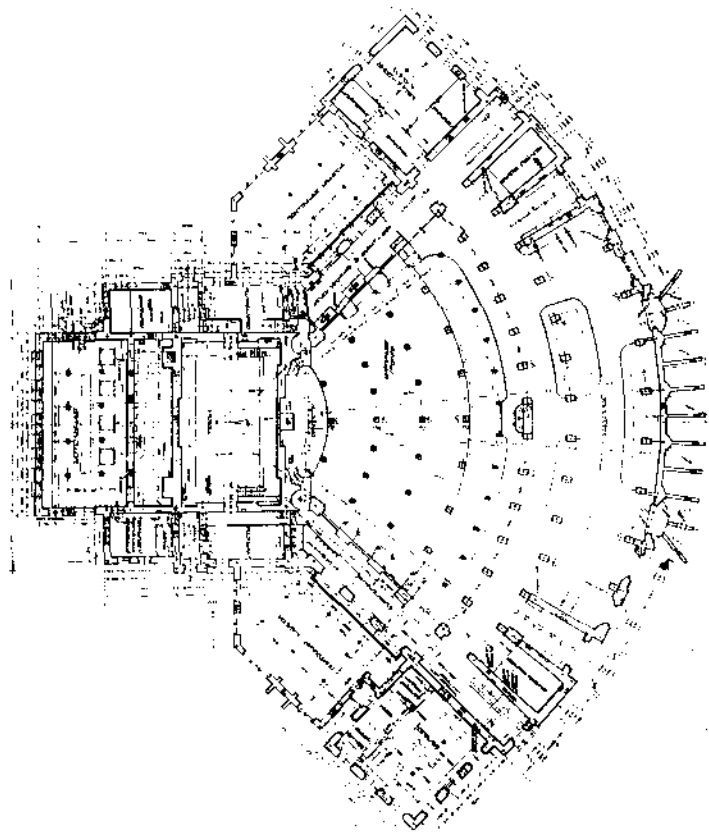
ДМИТРИЕВ А. И. АКАД. АРХ., ГР. ИНЖ. ЛЕНИНГРАД. ДВОРЕЦ РАБОЧЕГО ИМ. СТАЛИНА В ХАРЬКОВЕ.
