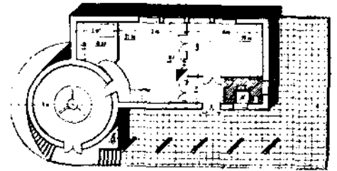
ТВЕЛЬКМЕЙЕР Л. Б. АРХ.-ХУД. Л.-ГРАД. ОБСЕРВАТОРИЯ В Г. СТАЛИНАБАДЕ. ПОСТРОЕНА В 1932 Г.
