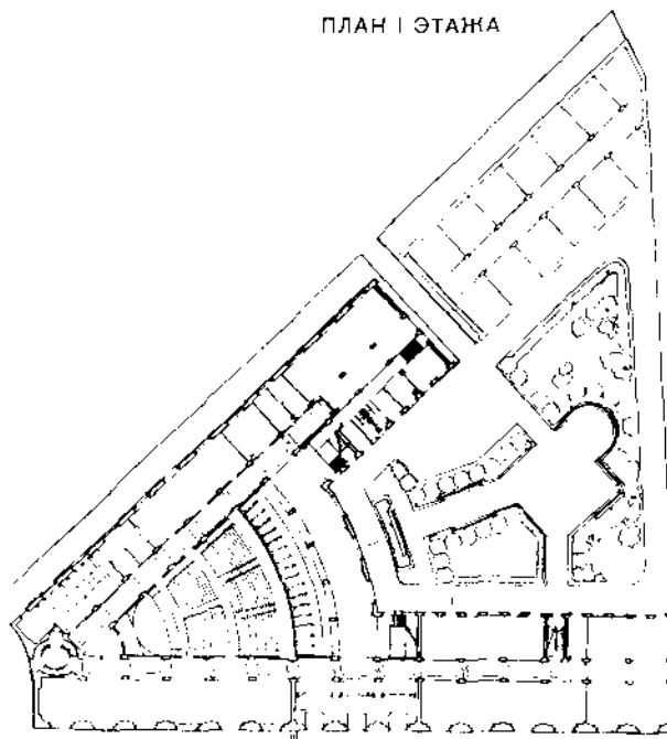
ПРОЕКТ ЗДАНИЯ АКАДЕМИИ ЛЕГКОЙ ПРОМЫШЛЕННОСТИ. СОВЕТСКИЙ ПР. УГ. КРАСНОЙ КОННИЦЫ. ЛЕНИНГРАД.
