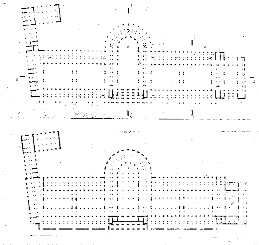
УНИВЕРМАГ НАРКОМСНАБА СССР В ЛЕНИНГРАДЕ. КАТОНИН Е. И., КАТОНИН Л. С., ГАЙКОВИЧ В. А., АРХ.-ХУД.-КИ КАТОНИН С. И. ИНЖ.
