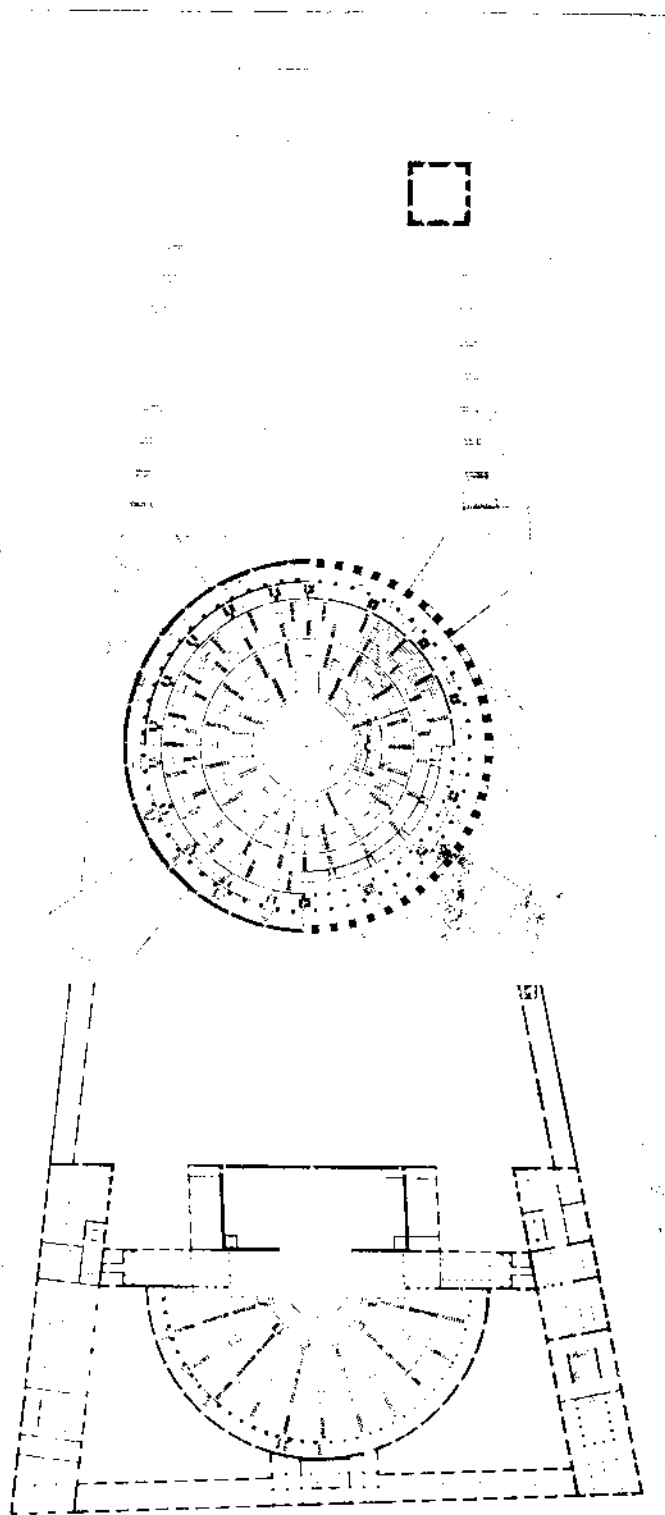
ЖОЛТОВСКИЙ, И. В., АКАД. АРХИТ. МОСКВА. ПРОЕКТ ДВОРЦА СОВЕТОВ В МОСКВЕ. ПРОЕКТ ПОЛУЧИВШИЙ ВЫСШУЮ ПРЕМИЮ НА КОНКУРСЕ.
