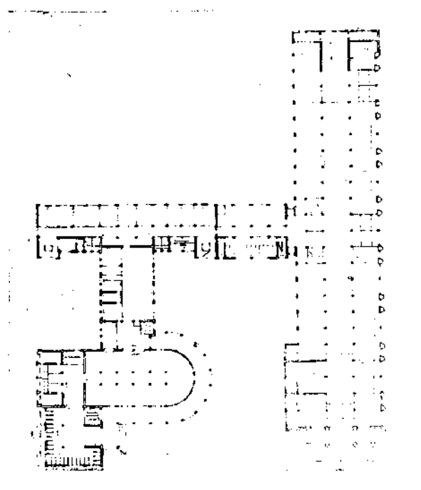
ПРОЕКТ УНИВЕРМАГА И СТОЛОВОЙ В СТАЛИНГРАДЕ. ПЕРСПЕКТИВА И ПЛАН ПЕРВОГО ЭТАЖА.
