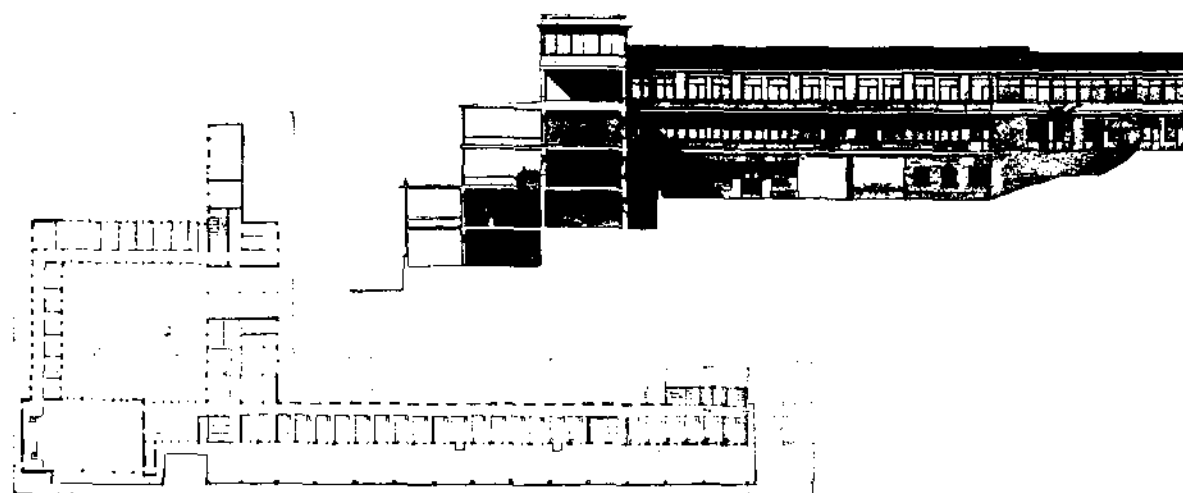
СЕЛЯКОВА-ШУХАЕВА Е. Н., СЕЛЮГИН Г. В. АРХ.-ХУД., ПРИ УЧАСТИИ РЕЙМЕРС Е. К. АРХ.-ХУД. И СТУД. АРХ.-ФАКА АКАДЕМ.-ХУДОЖЕСТВ ШУХАЕВОЙ М. И ГАНКЕВИЧ В. ЛЕНИНГРАД. КОНКУРСНЫЙ ПРОЕКТ ДОМА ОТДЫХА И.Т.Р. В НОВЫХ ГАГРАХ. 1933 г.
