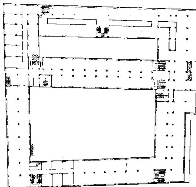
ПЛАН 2 ЭТАЖА
