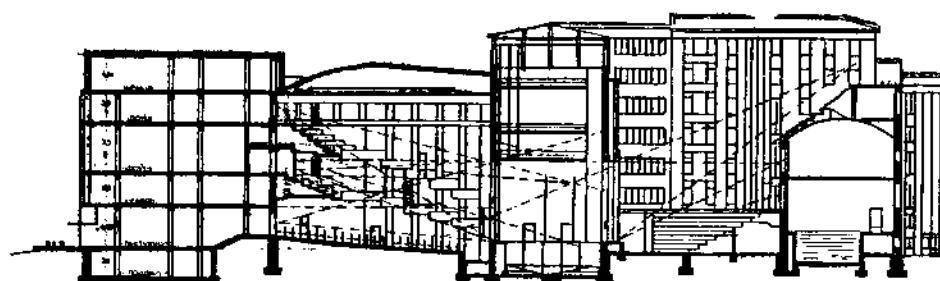
ОВСЯННИКОВ С. О. АРХИТЕКТОР-ХУДОЖНИК, ПОМПЕЕВ Б. С. АРХИТЕКТОР. НАРОДНЫЙ ДОМ В Г. РИГЕ (ЛАТВИЯ). 2-я ПРЕМИЯ НА МЕЖДУНАР. КОНКУРСЕ. 1929 г.
