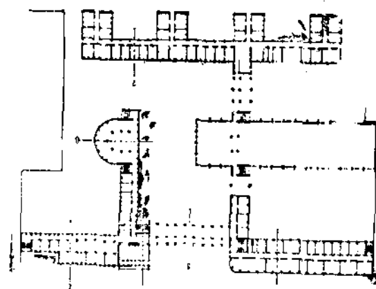
ПРОЕКТ ЗДАНИЯ НАУЧНО-ИССЛЕДОВАТ. ИН-ТА „МЕХАНОБР“.
