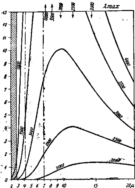
Рис. 76а. Спектральное распределение интенсивности теплового излучения по Планку для разных температур; заштрихованная часть изображает ультрафиолетовую область (до 0,28 \mu ); видимая часть спектра лежит между пунктирными линиями. Сразу видно полное согласие с наблюдениями (см. рис. 75).
