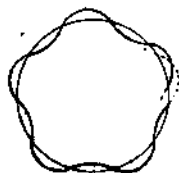
Рис. 54. Круговое движение волны; однозначное волновое движение может образоваться только в том случае, если длина окружности равна целому кратному длине волны.
