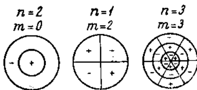
Рис. 56. Некоторые формы колебаний натянутой круглой мембраны; как это принято в квантовой механике, число радиальных узловых линий обозначено через n - 1 , число азимутальных узловых линий — через m ; n и m суть квантовые числа колебательного состояния.
