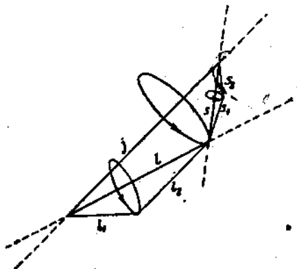
Рис. 68. Схема связи Расселя-Саундера или связи ( l_s ). В первом приближении моменты орбит электронов складываются в общий орбитальный момент l , затем моменты спина складываются в один результирующий момент спина, и, наконец, l и s складываются вместе в один общий вращательный момент j .
