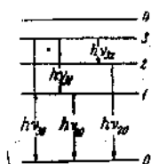
Рис. 31. Комбинационный принцип Ритца.
