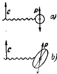
Рис. 85. Пронхождение деполяризации вследствие анизотропии поляризуемости. а) В случае изотропной молекулы индуцированный дипольный момент колеблется в направлении электрического вектора световой волны. б) В случае анизотропной молекулы он колеблется под углом к направлению E , что и вызывает деполяризацию рассеянного света.
