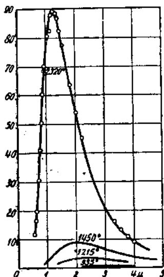
Рис. 75. Распределение интенсивности в зависимости от длины волны по измерениям Люммера и Прингсгейма.
