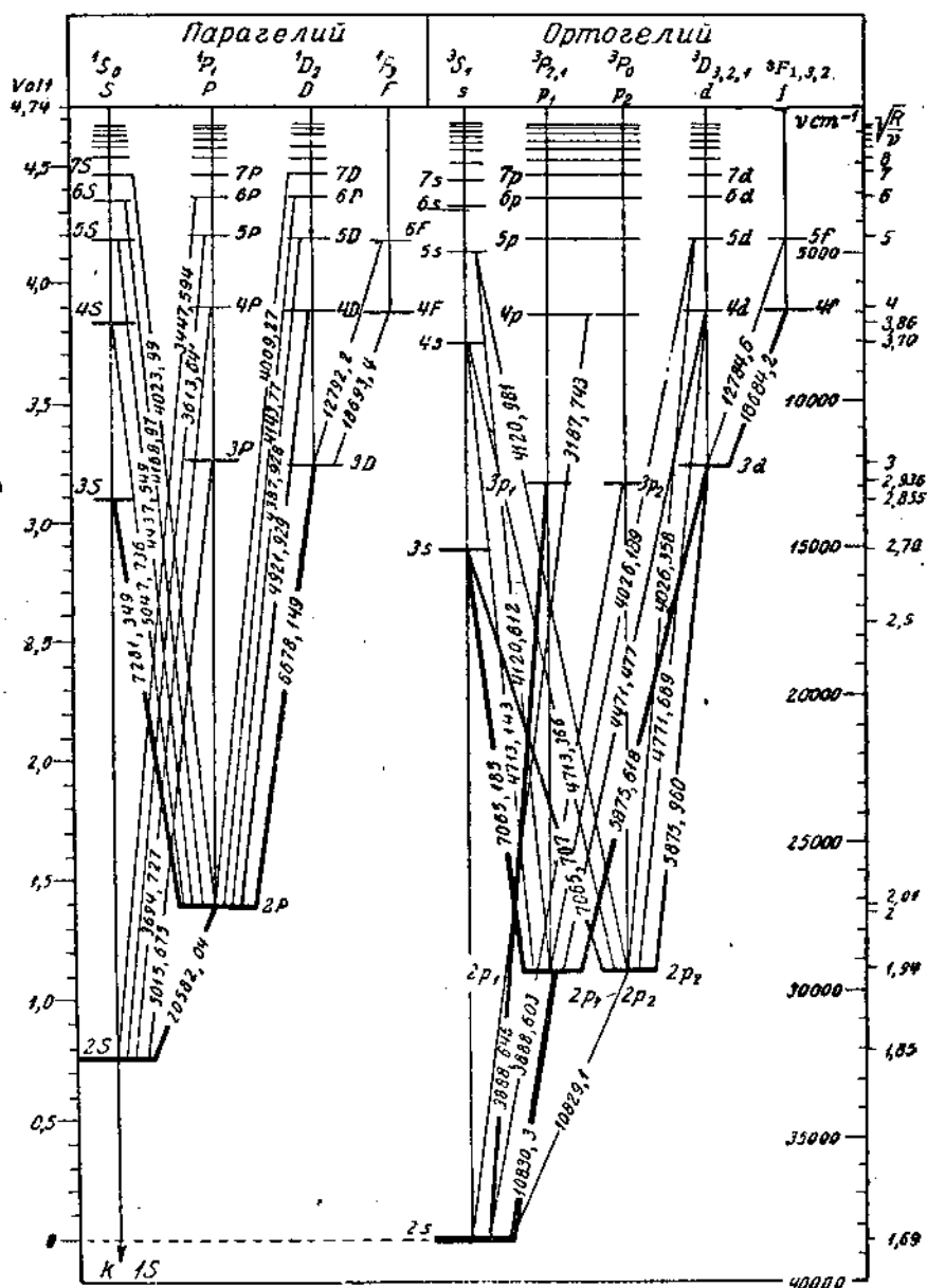
Рис. 69. Схема термов гелия. Не существует линий, соответствующих переходам между термами орто- и парагелия. При не слишком большой разрешающей силе ортогелий имеет дублетный спектр (по Grotrian'y).
