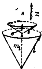
Рис. 64. Векторная модель в случае эффекта Пашена-Бака (переход к нормальному эффекту Зеемана). Так как энергии момента орбиты и спина в магнитном поле больше, чем магнитное взаимодействие между орбитой и спином, то моменты орбиты и спина прецессируют отдельно друг от друга вокруг направления поля.
