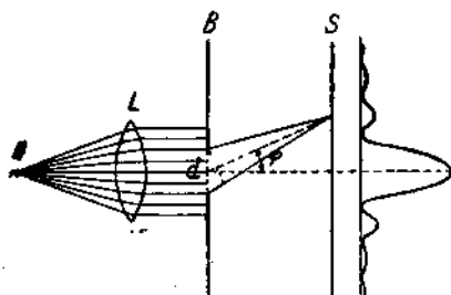
Рис. 27. Явление диффракции луча при прохождении сквозь узкую щель. Изображение имеет большой максимум интенсивности для угла отклонения \varphi = 0 и кроме того ряд равноотстоящих максимумов интенсивности, становящихся все слабее с увеличением угла отклонения.
