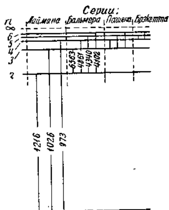
Рис. 39. Схема термов водородного атома. Здесь нанесены важнейшие линии водородного спектра, как переходы между двумя термами Бальмера (частично с указанием длин волн).
