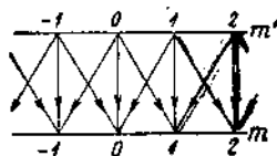
Рис. 48. Переходы в магнитном поле: на основании правил отбора \Delta m = 0, \pm 1 имеют место только переходы, указанные стрелками; так как термы с различным m в однородном магнитном поле лежат на равном расстоянии друг от друга, то каждая спектральная линия расщепляется в магнитном поле только на три линии (нормальный эффект Зеемана).
