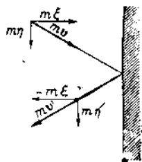
Рис. 2. Диаграмма импульсов в случае упругого удара молекулы о стенку; энергия, величина импульса и его составляющая, параллельная стенке, при ударе не изменяются, а составляющая, перпендикулярная к стенке, изменяет знак; поэтому при ударе молекулы стенке сообщается импульс, равный 2m\xi .
