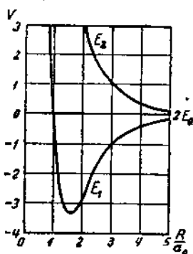
Рис. 88. Потенциальные кривые при гомеополарной связи ( H_2 ). Мы имеем кривую с потенциальным минимумом (притяжение) и кривую, соответствующую чистому отталкиванию (по Гейтлеру и Лондону, см. п. 47).
