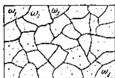
Рис. 3. Разделение объема газа на клетки для определения наиболее вероятного распределения плотности молекул газа.
