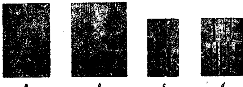
Рис. 59. Расщепление спектральных линий в магнитном поле (по Е. Баку 4 и А. Ланде). а — нормальный триплет Лоренца в случае линии кадмия 6489 (нижние линии колеблются перпендикулярно к магнитным силовым линиям, а верхние — параллельно к ним); б — аномальный эффект Зеемана у D-линий натрия (наверху с магнитным полем, а внизу без него); с и d изображают эффекты Зеемана у линий хрома (верхние линии колеблются параллельно полю, а нижние — перпендикулярно).
