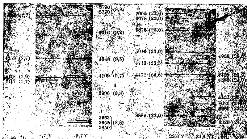
Рис. 32 и 33. Возбуждение спектральных линий ударом электронов (по Герцу). В спектре появляются только те линии, для которых потенциал возбуждения (числа в скобках) меньше энергии электронов (показаны под снимками). Рис. 32 относится к ртути а рис. 33—к галлию. Длины волн показаны в огистремах (Hertz, Z. Physik 22, 24).
