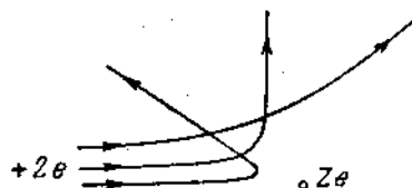
Рис. 25. Отклонение \alpha -частиц ядром с зарядом, равным Z ; пути \alpha -частиц представляют собой гиперболы.
