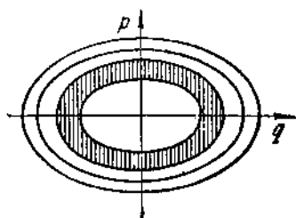
Рис. 41. Фазовые орбиты линейного вибратора; в плоскости pq фазовая точка описывает эллипс, площадь которого есть целое кратное h\nu (по А. Зоммерфельду, Строение атома и спектры).
