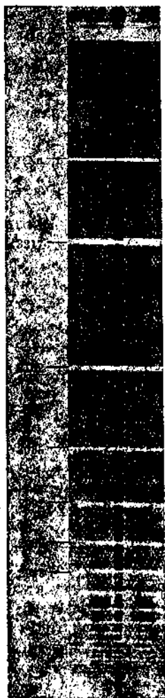
Рис. 49. Спектр испускания паров калия; между двумя верхними линиями калия показана одна линия натрия (по Н. Калла, Z. Physik 76).
