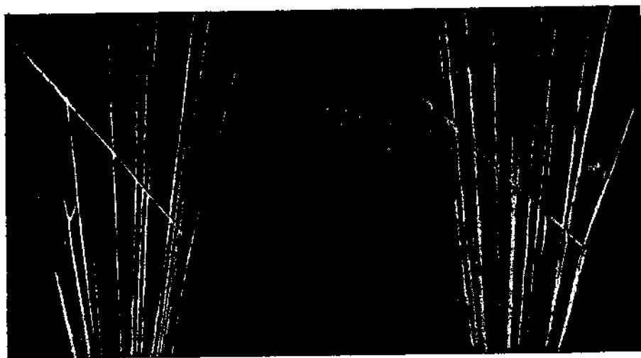
Рис. 22. Стереоскопический Вильсоновский снимок процесса расщепления атома (по Блеккету). Превращение азота с поглощением \alpha -частицы. Ясно видно разделение луча (пути \alpha -частицы); из двух ветвей более слабая соответствует протону, выбитому из ядра азота, а более сильная — ядерному остатку.
