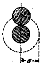
Рис. 7. Газокинетическое сечение столкновения. Центры тяжести двух молекул могут приблизиться только на расстояние \sigma ( \sigma = диаметру молекулы).
