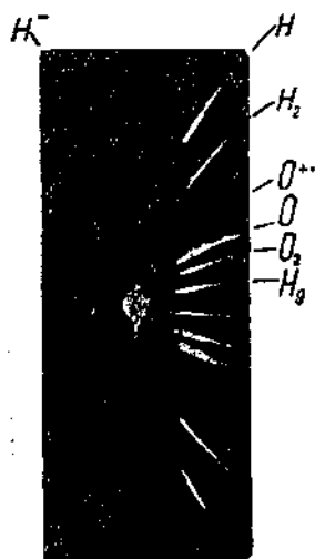
Рис. 15. Параболы катодных лучей по Дж. Дж. Томсону. На основании этих снимков отклонений может быть установлена связь между отдельными параболом и химическими элементами и соединениями. Электрические и магнитное отклоняющие поля параллельны к касательным в вершинах парабол (по Geiger-Scheel, Handbuch der Physik 22).
