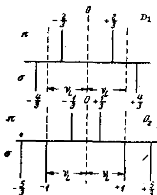
Рис. 95. Расщепление D-линий натрия при аномальном эффекте Зеемана. За единицу взято расщепление при нормальном эффекте. Сверху указаны три \pi -составляющие, поляризованные параллельно к полю, а внизу — \sigma -составляющие, поляризованные в перпендикулярном к полю направлении.
