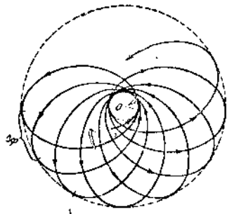
Рис. 44. Орбита электрона вокруг ядра, если принять в расчет релятивистскую переменность массы (розетка); движение двукратно-периодично, перигелий P перемещается при одном обороте на угол \Delta\phi (по Зоммерфельду).
