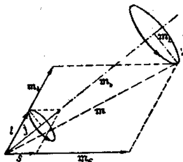
Рис. 61. Векторная модель при аномальном эффекте Зеемана. Направление результирующего вращательного импульса не совпадает с направлением результирующего магнитного момента; эффективной является только составляющая m_{||} , параллельная j ; другая составляющая m_{\perp} в среднем равна нулю вследствие вращения всей системы векторов вокруг j (общего вращательного импульса).
