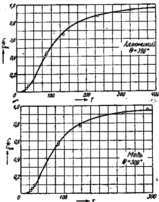
Рис. 77. Изменение теплоемкости при низких температурах по Дебаю; кружочки представляют собой измеренные точки, а кривые соответствуют теории Дебая.
