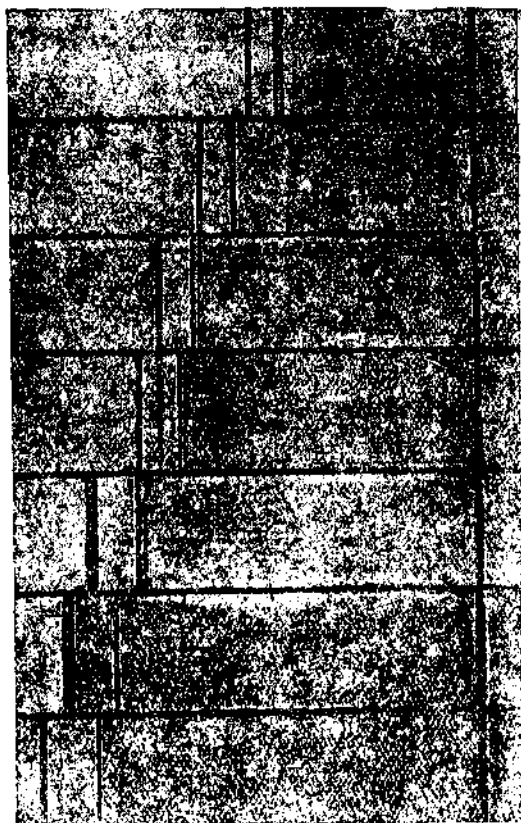
Рис. 51. Снимки вращения кристалла К-серии между мышьяком ( Z = 33 ) и ренгем ( Z = 47 ). Ясно видно усиление жесткости с возрастанием порядкового числа. Слева виден след отклоненного первичного луча (по Зомерфельду).
