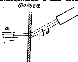
Рис. 24. Схема опыта для наблюдения движения \alpha -частиц; с помощью счетчика Гейгера можно сосчитать число \alpha -частиц, которые отклоняются на определенный угол \theta , от своего первоначального направления.
