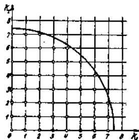
Рис. 79. Подсчет числа собственных колебаний; число колебаний с длиной волны > \lambda равно числу узловых точек сетки, находящихся внутри окружности, а это число приблизительно равно площади квадрата круга.
