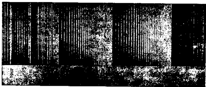
Рис. 89. Полосы азота (в видимой части спектра). Видны тонкие „триплеты“, соответствующие различным вращательным переходам (на -1, 0, 1 ); правильный ряд этих триплетов образует полосу вращения с определенной границей (квантом). Все эти отдельные полосы соответствуют скачку колебательного квантового числа и электронному скачку, смещающему систему в видимую часть спектра.
