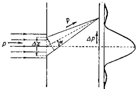
Рис. 36. Диффракция электронов от щели.
