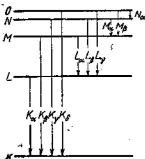
Рис. 52. Схема термов рентгеновских уровней (по Косселю) с переходами, соответствующими рентгеновским линиям.
