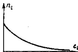
Рис. 4. Закон распределения Больцмана: при равной величине ячеек, клетки с большей энергией содержат меньшее количество частиц, чем клетки с меньшей энергией.
