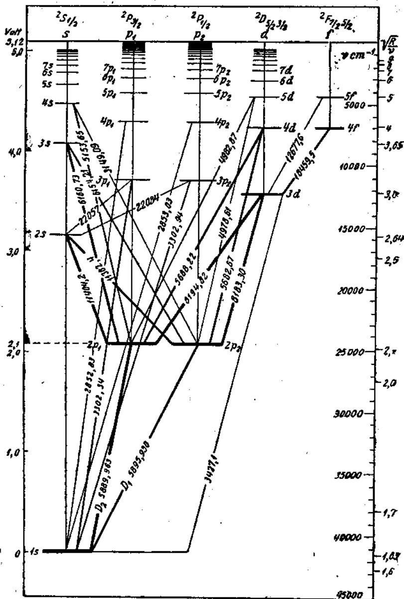
Рис. 66. Схема термов натрия при учете электронного спина. Схематически показаны энергии термов в электрон-вольтах (считая от основного состояния), а справа — частоты в волновых числах, которые испускаются при переходе от границы серии вниз, а также значения \sqrt{\frac{R}{n}} (по W. Gretrian, Graphische Darstellung der Spektren, II Teil).
