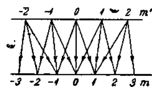
Рис. 62. Переходы при аномальном эффекте Зеемана; так как расщепление в отдельных группах термов различно, то в общем получается столько же отдельных линий, сколько вообще возможно переходов.
