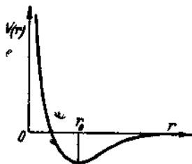
Рис. 86. Потенциальная кривая в зависимости от расстояния между обоими объединенными в молекулу атомами. Положение равновесия находится на расстоянии r_0 .
