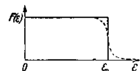
Рис. 80. Кривая распределения Ферми. Сплошная ломаная линия соответствует абсолютному нулю ( T=0 ), пунктирная — температуре, отличной от нуля.
