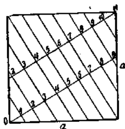
Рис. 78. Прямое собственное колебание в ящике; на каждое ребро должно прийти целое число полуволи (в нашем примере k_1 = 11 , k_2 = 7 ).
