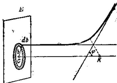
Рис. 93. Относительная частота рассеяния в определенном телесном углу.
