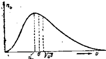
Рис. 5. Максвелловский закон распределения скоростей с указанием наиболее вероятной скорости ( v_0 ), средней скорости ( v ) и корня квадратного из среднего квадрата скорости ( \sqrt{v^2} ).
