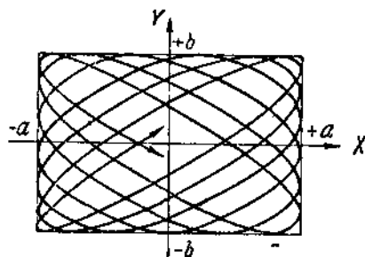
Рис. 43. Изображение фазовой кривой для системы с двумя степенями свободы, в которой обе частоты \nu_1 и \nu_2 несоизмеримы (фигуры Лиссажу) (по Зоммерфельду).
