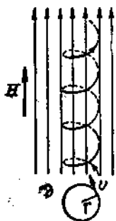
Рис. 12. Движение электрона в постоянном магнитном поле H ; путь движения вообще есть винтовая линия (ось ее параллельна магнитному полю); в частном случае, когда движение электрона перпендикулярно к магнитному полю, этот путь есть окружность.
