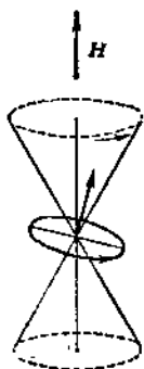
Рис. 46. Волчкообразное движение нормали к орбите электрона во внешнем поле; нормаль описывает изображенный на рисунке конус.
