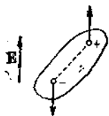
Рис. 82. Момент вращения, испытываемый во внешнем электрическом поле молекулой с постоянным дипольным моментом.
