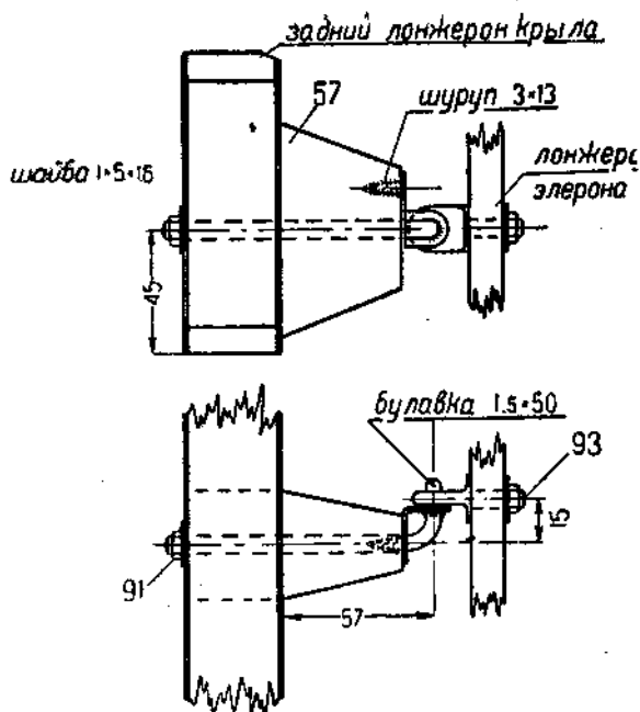
Фиг. 28. Шарнир элерона
