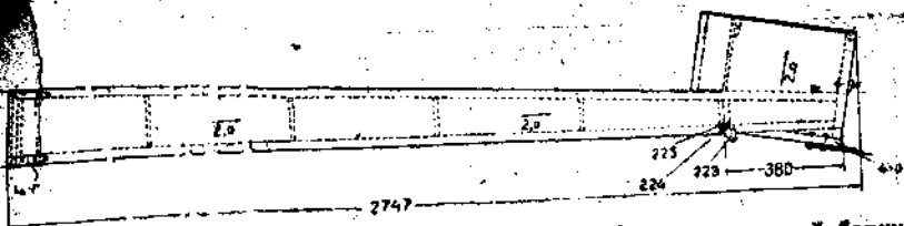
Фиг. 9. Схема хвостовой балки
