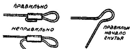
Фиг. 34. Заделка стальной проволоки
