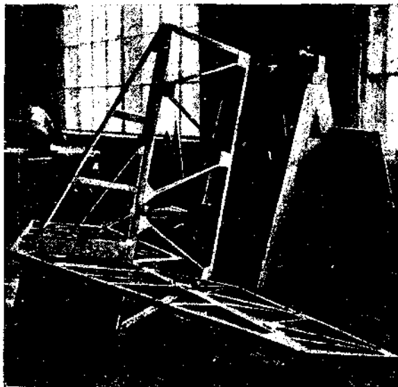
Фиг. 11. Оперение в собранном виде
