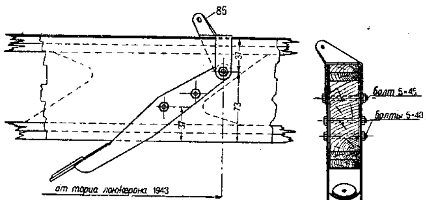
Фиг. 26. Крепление подкоса на заднем лонжероне
