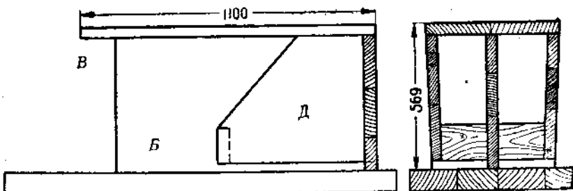
Фиг. 31. Приспособление для сборки обтекателя
