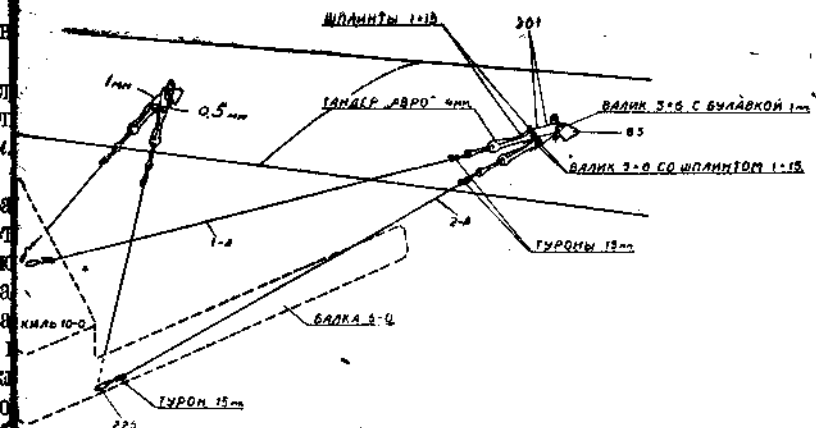
Фиг. 40. Схема расчалки хвоста
