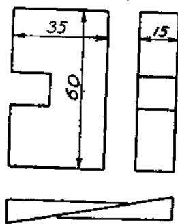
Фиг. 20. Хомутик для склейки
