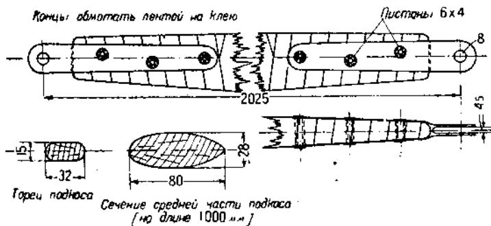
Фиг. 3. Подкос крыла
