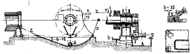
Разрѣзъ по А-В.
