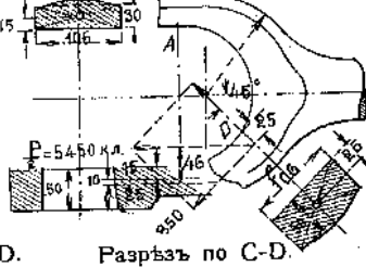
Разрѣзъ по С-Д.
