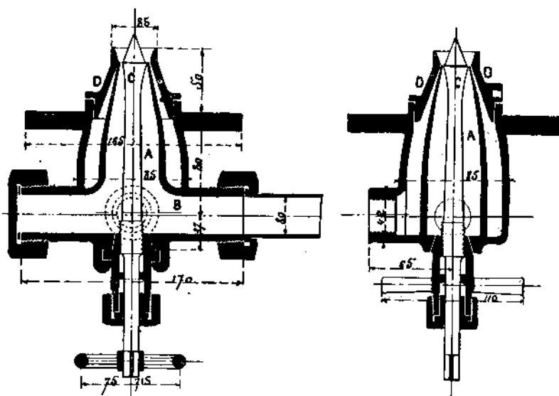
FIG. 182 et 183. — Brûleur système d'Allest.
