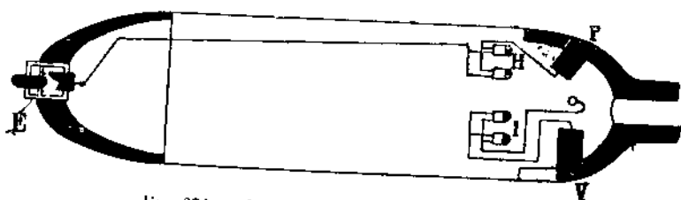
FIG. 272. — Détails de l'obus-torpille Zalinski.
