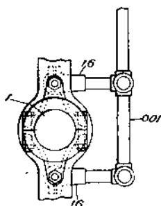
FIG. 225. Embrayage Norris.
