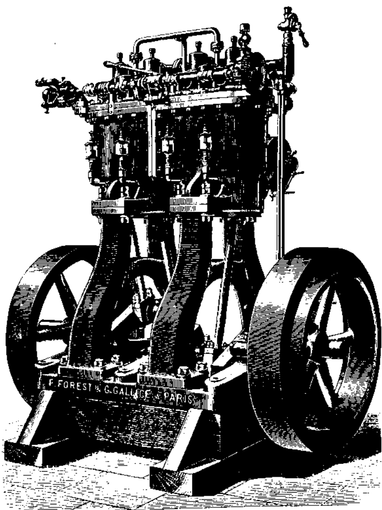
FIG. 181. — Moteur à renversement de marche Forest et Gallice.
