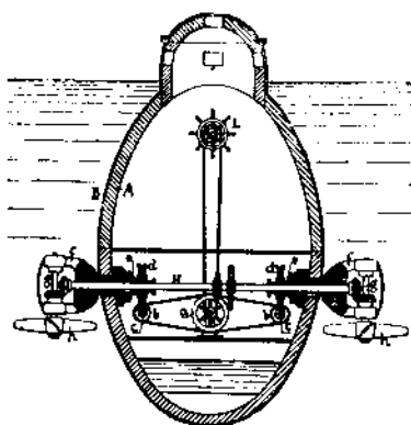
FIG. 26. — Hélices mobiles de Baker.
