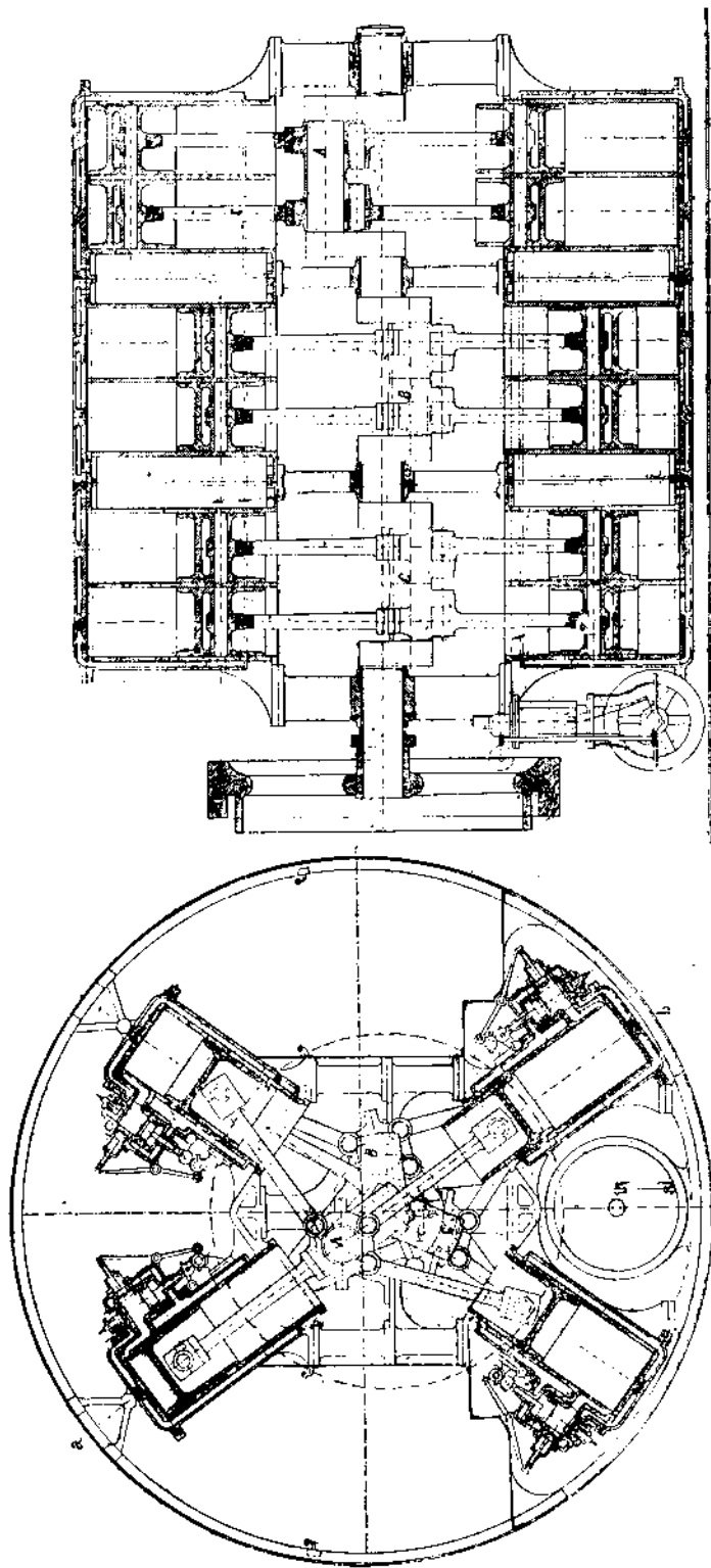
FIG. 193 et 194. — Coupes transversale et longitudinale d'un moteur à pétrole à 21 cylindres, système Forest.
