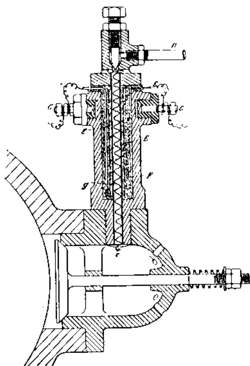
FIG. 171. Vaporisateur électrique Southey.
