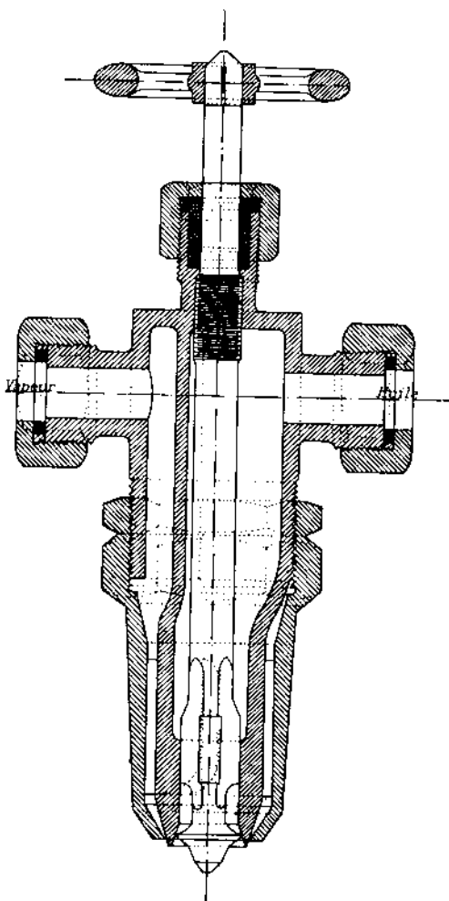
FIG. 151. — Brûleur Seigle.
