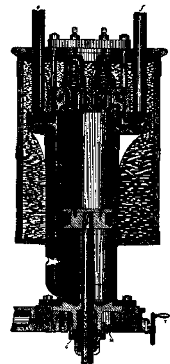
FIG. 305. — Compresseur de la Consolidated Ice Machine Co.
