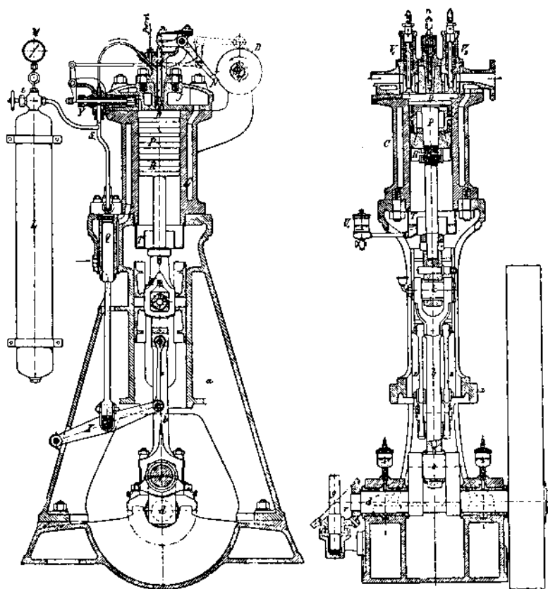
FIG. 202 et 203. — Machine Diesel de 20 chevaux (1897), à cylindre de 250 × 400. Coupes verticales orthogonales.
