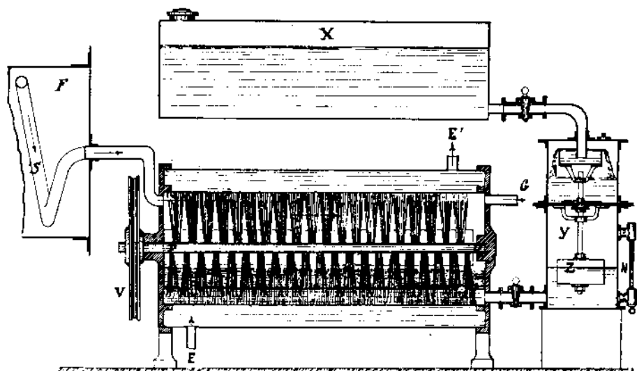
FIG. 159. — Carburateur Forest.
