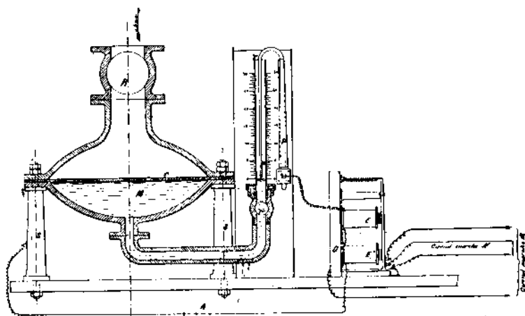
FIG. 12. — Manomètre à mercure, F. Forest.
