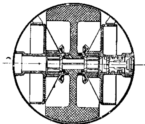
FIG. 253. — Le volant de la torpille Howell.
