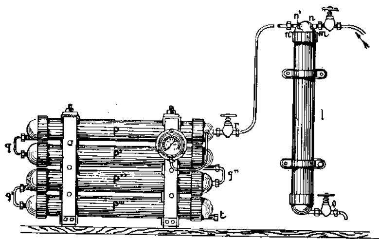
FIG. 304. — Accumulateur d'air.
