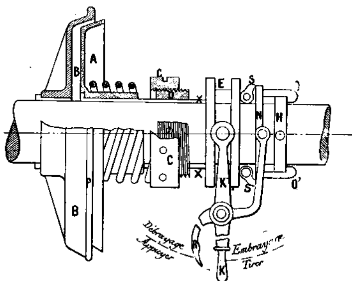
FIG. 296. — Embrayage Goubet.
