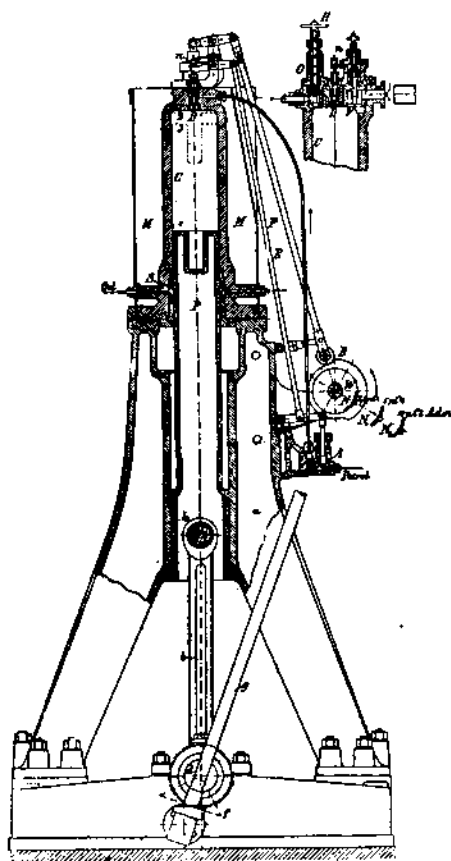
FIG. 201. — Moteur Diesel de 1893.
