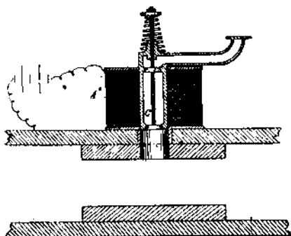
FIG. 172 et 173. Vaporisateurs électriques Rowbotham.
