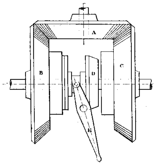
FIG. 214. — Changement de marche employé par la maison Herliq.
