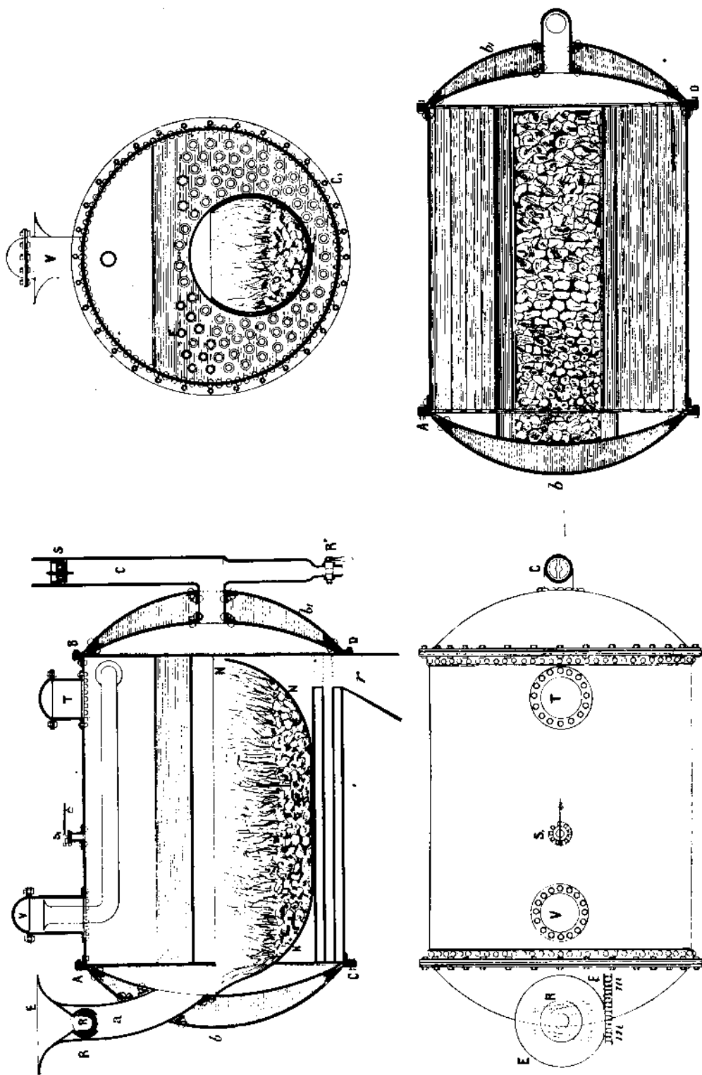
FIG. 132 à 135. — Chaudière du D r Payerne.
