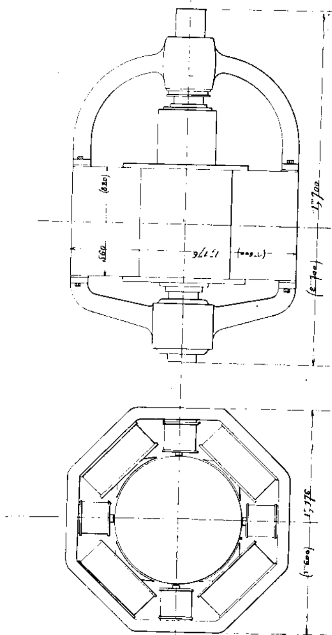
FIG. 130 et 131. — Schéma d'un électromoteur 150.000 watts.
