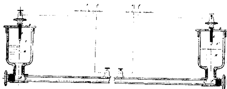
FIG. 19. — Niveau à mercure Forest.
