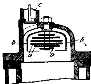
FIG. 168. — Vaporisateur Spiel.
