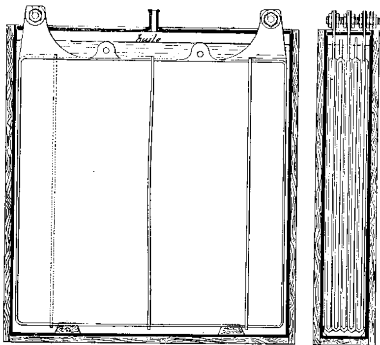
FIG. 95 et 96. — Accumulateur Laurent-Cély.
