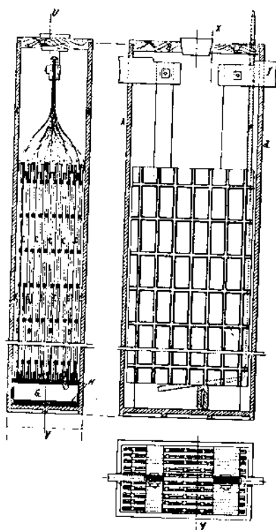
Fig. 92, 93 et 94. Accumulateur Commelin-Desmazures.
