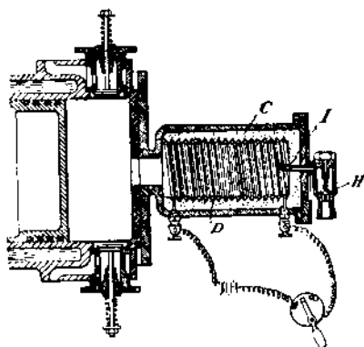
FIG. 169 et 170. — Vaporisateur Arrol.
